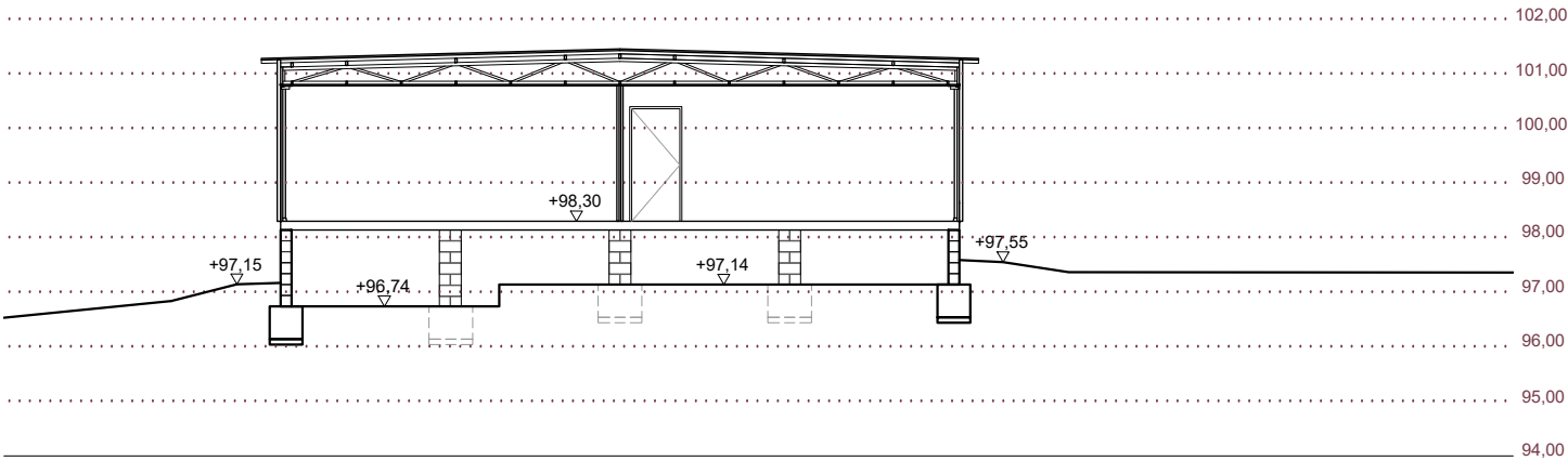
SECCIÓ H-H'
