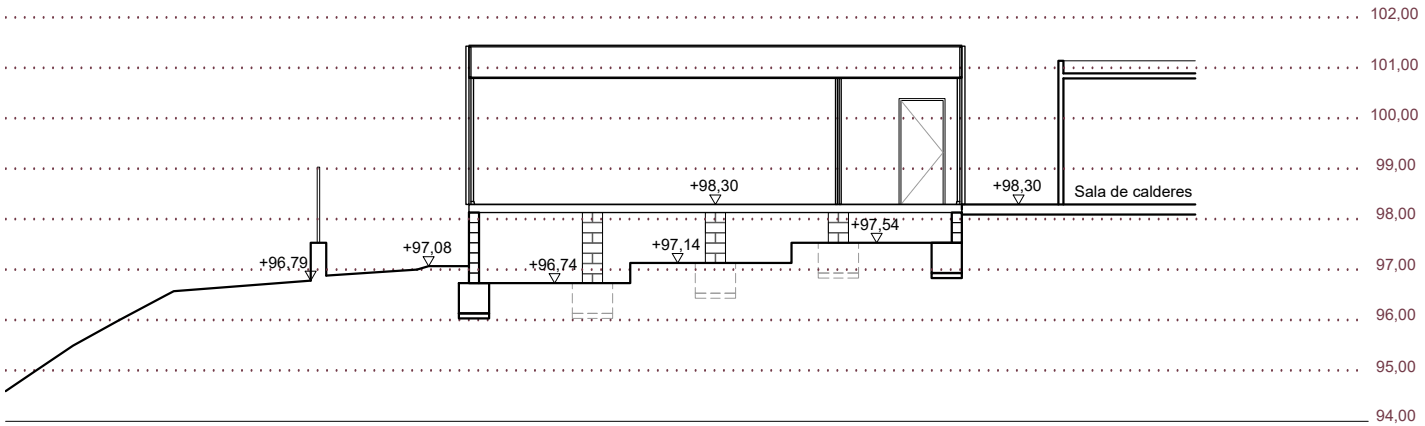
SECCIÓ D-D'
