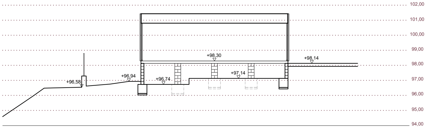
SECCIÓ B-B'
