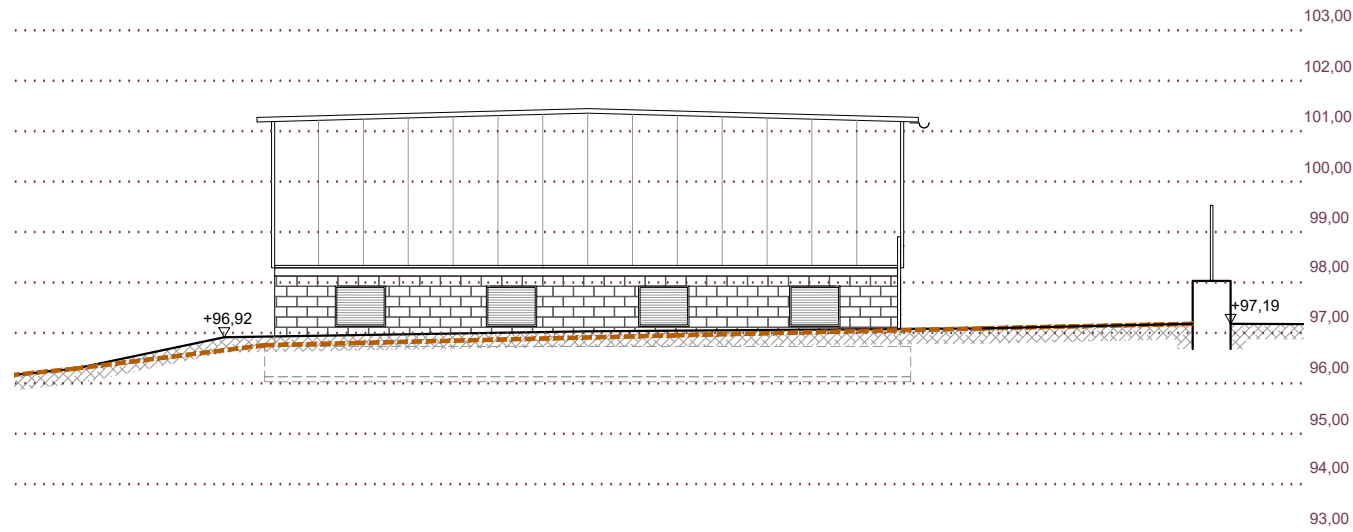
ALÇAT B
