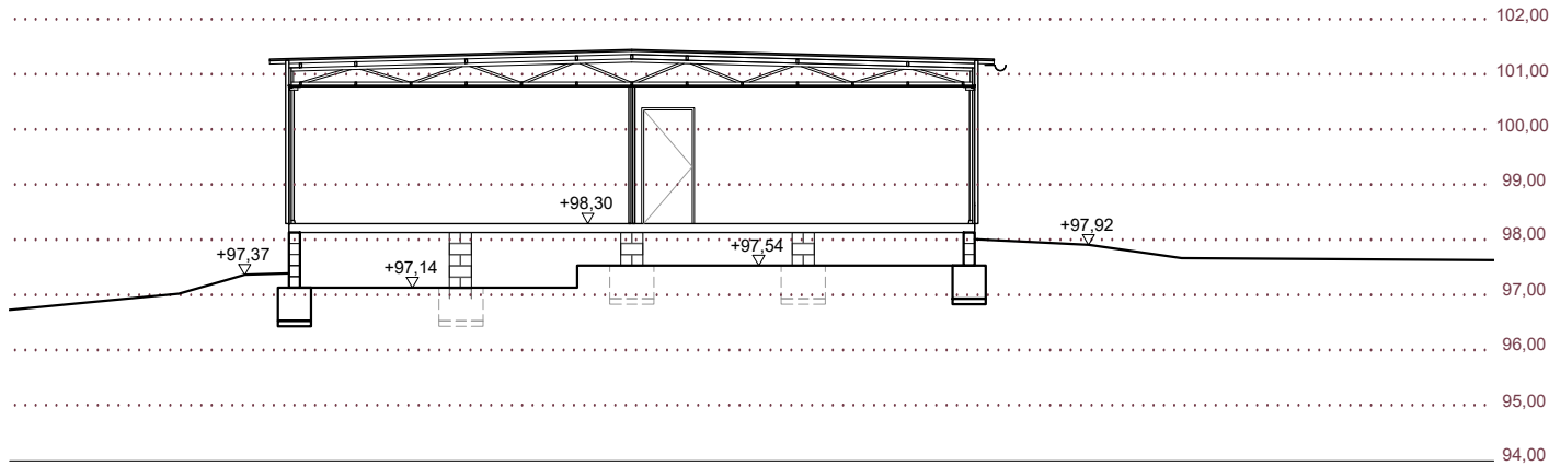
SECCIÓ G-G'
