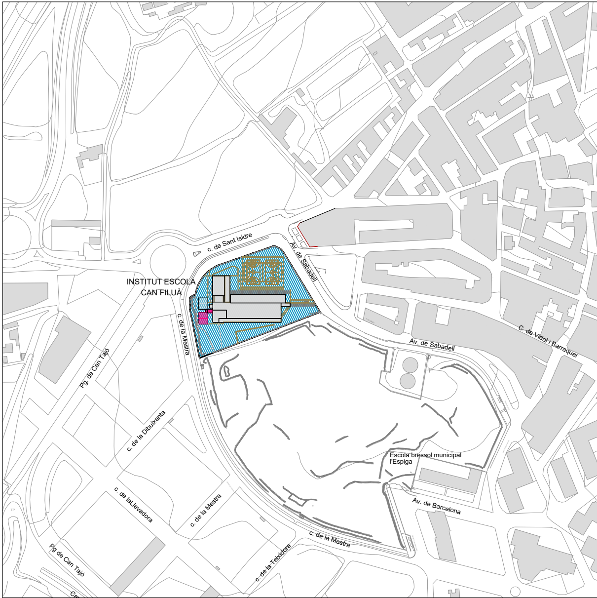
SITUACIÓ Esc. 1/2.000
