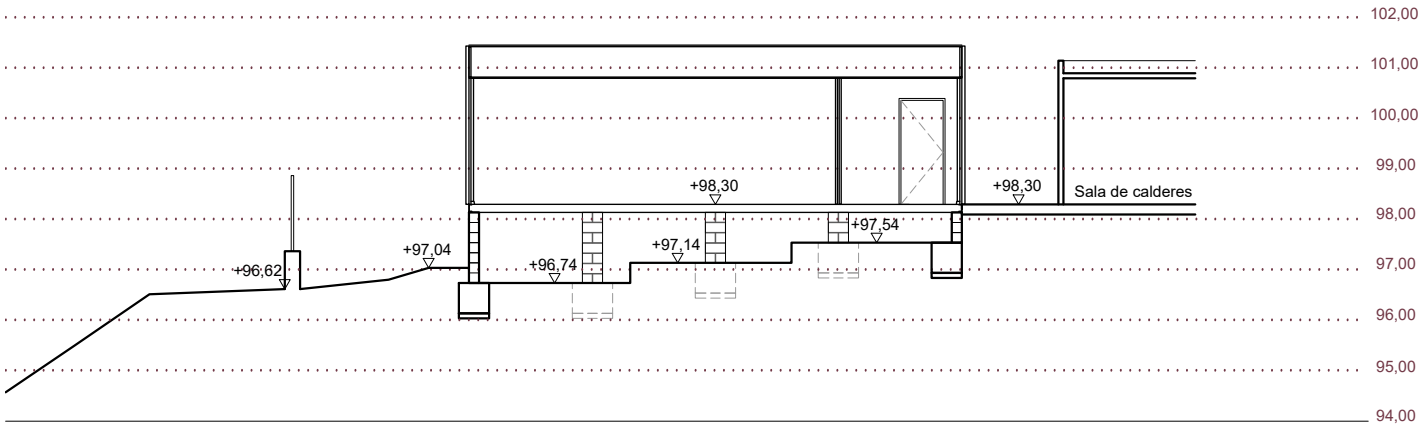
SECCIÓ C-C'
