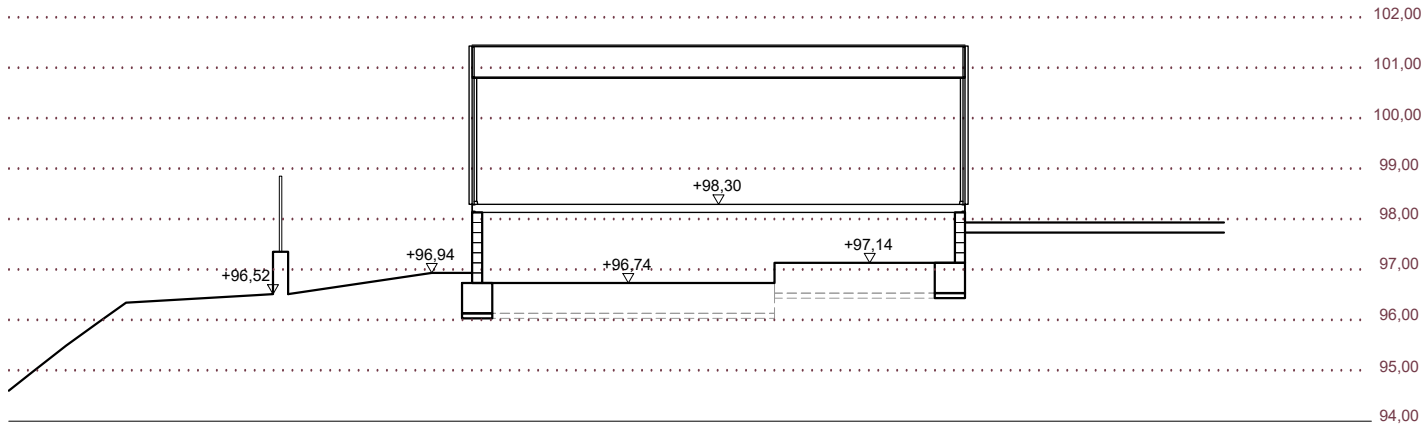
SECCIÓ A-A'
