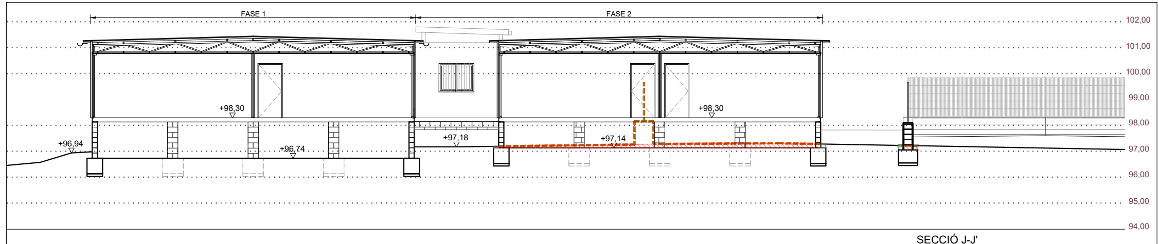
SECCIÓ J-J'
