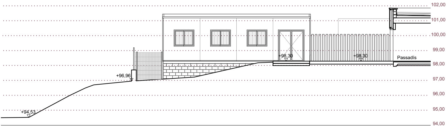
SECCIÓ E-E'
