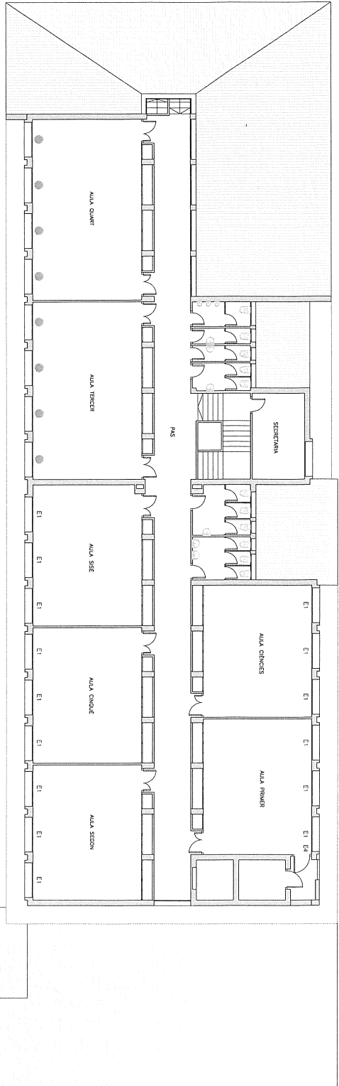
PLANTA PRIMERA E: 1/200
