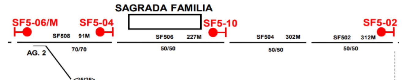
Figura 11. Interestació Sant Pau – Sagrada Família per via 2.
