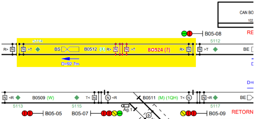
Figura 6. Nou circuit de via BO524 a l'enclavament de Can Boixeres.
