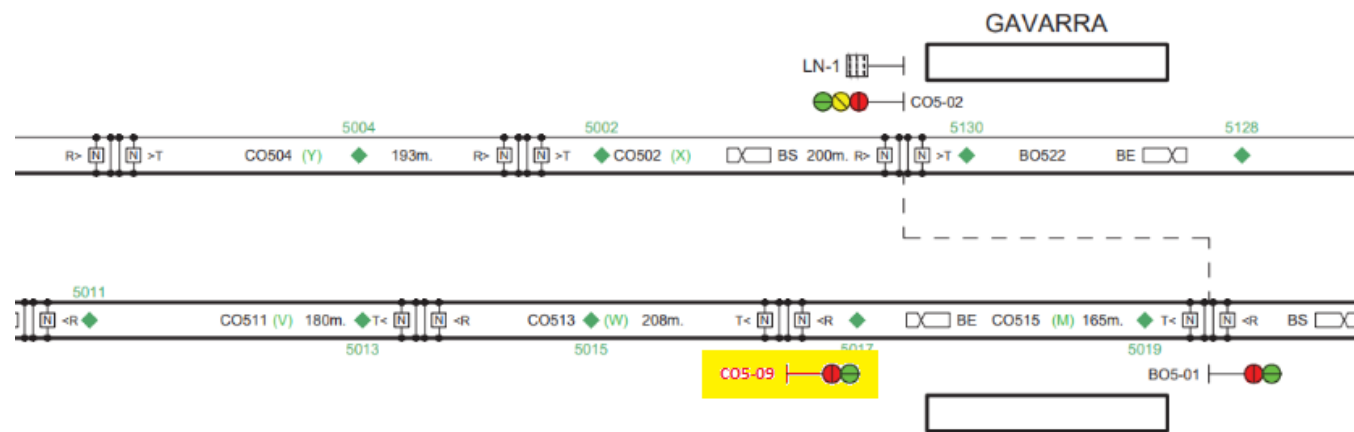
Figura 2. Nou senyal CO5-09.
