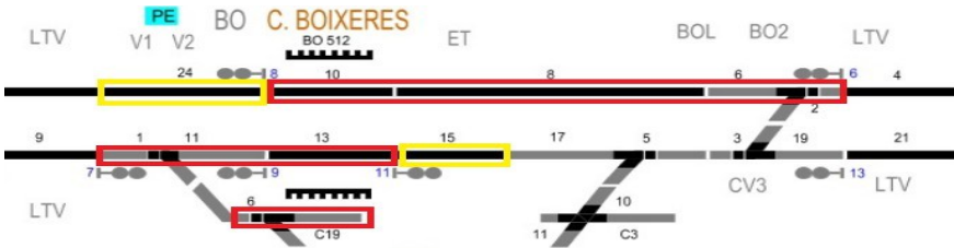
Figura 4. Modificació d' activació de l' aspecte verd en els senyals 6 i 7 de l' enclavament de Can Boixeres.
