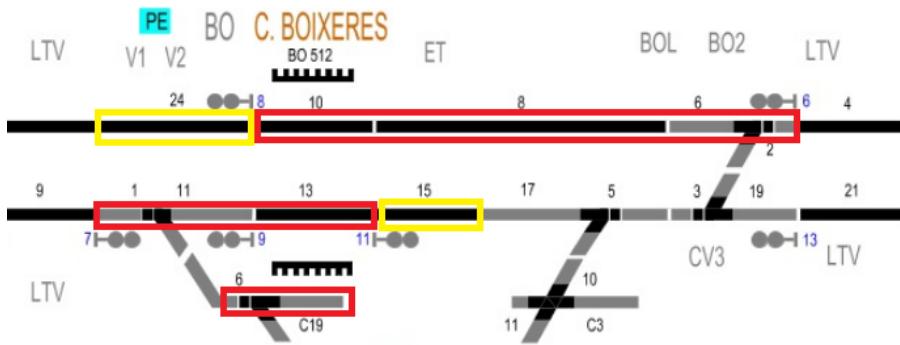
Figura 8. Activació de l'aspecte verd a les senyals 6 i 7 de l'enclavament de Can Boixeres.
