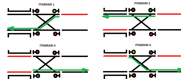
Figura 3. Nova funcionalitat de la volta automàtica alternativa.
