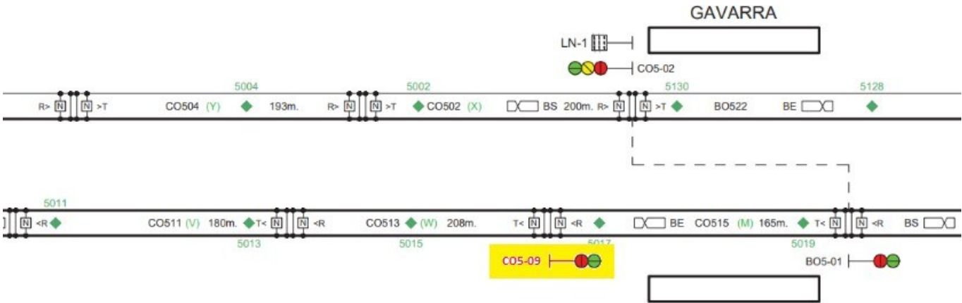
Figura 2. Nou senyal CO5-09 a instal·lar entre els circuits CO513 i CO515.
