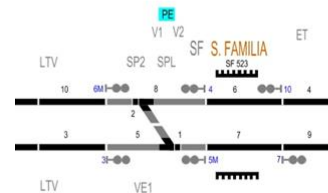
Figura 12. Configuració de via al canvi d'agulles del ENCE de Sagrada Família.
