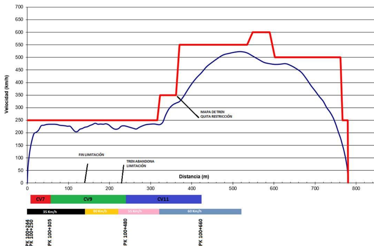
Figura 5. Perfil de velocitat a la interestació entre Cornellà V1 i Gavarra V1.
