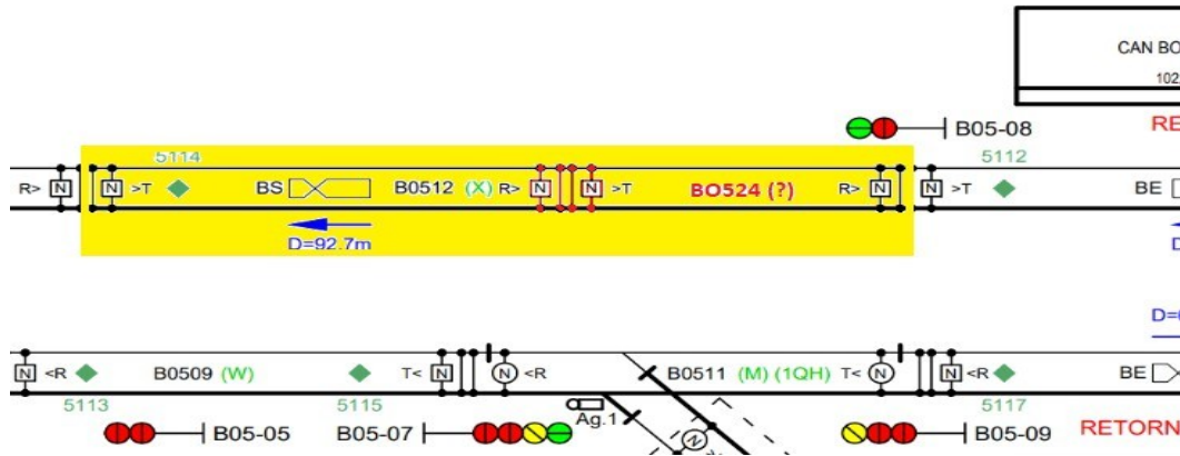
Figura 3. Nou circuit de via BO524 a l'enclavament de Can Boixeres.
