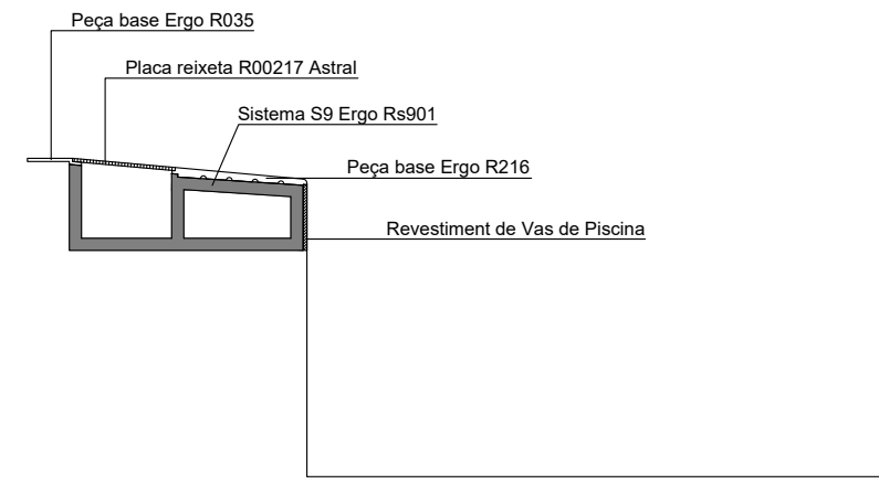
DETALL PISCINA DESVORDANT Esc 1/20
