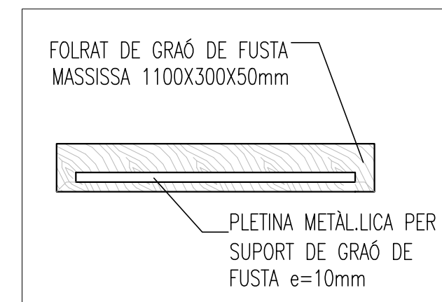
DETALL GRAÓ EN TRAM D'ESCALA DE PLANTA BAIXA A PLANTA PRIMERA
