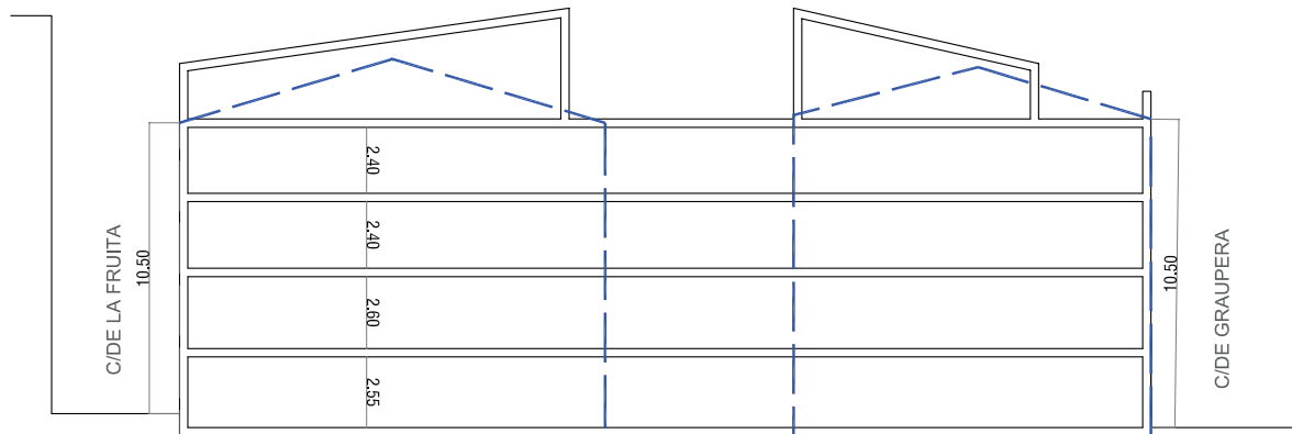
SECCIÓ LONGITUDINAL
