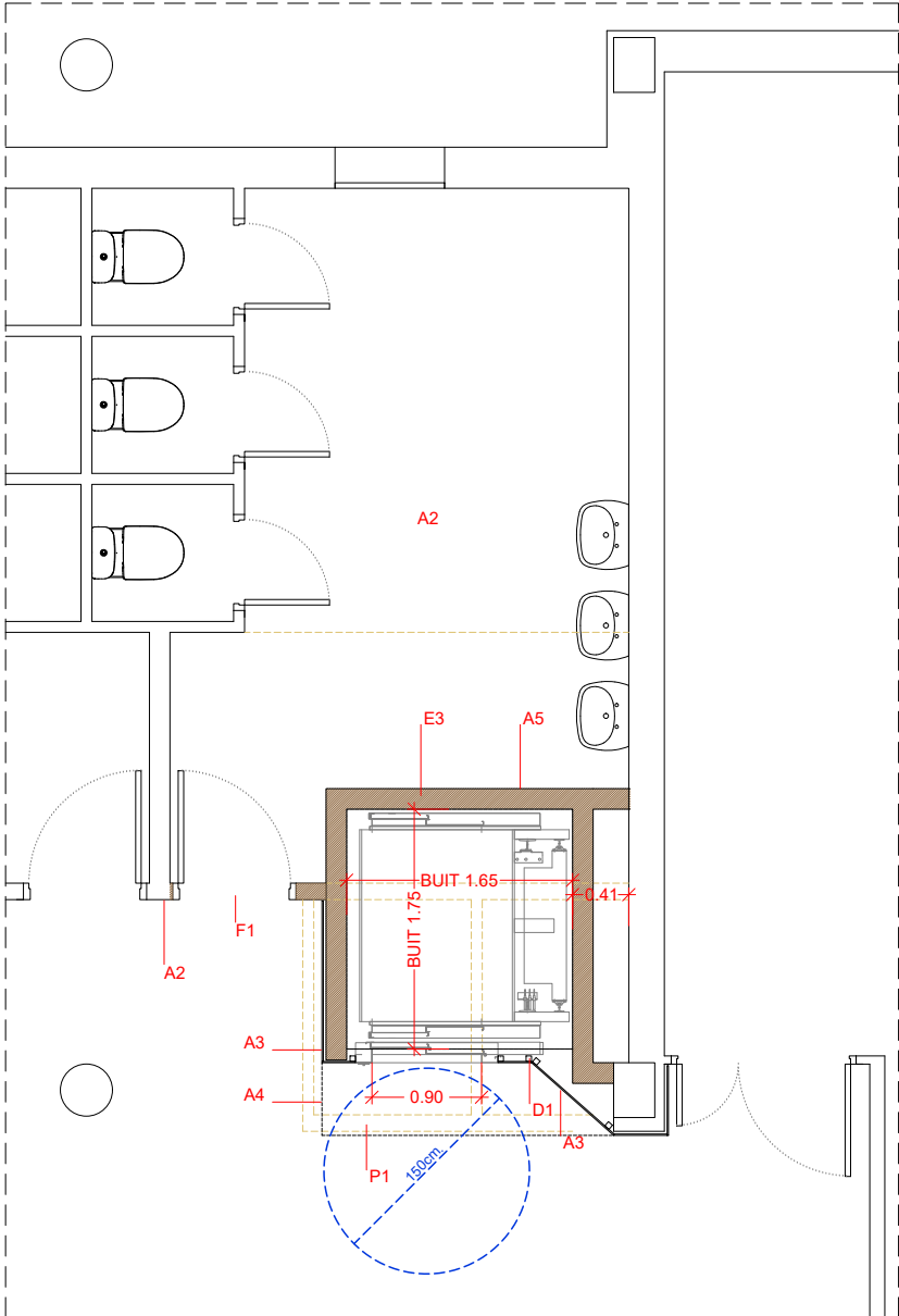
PLANTA PRIMERA
