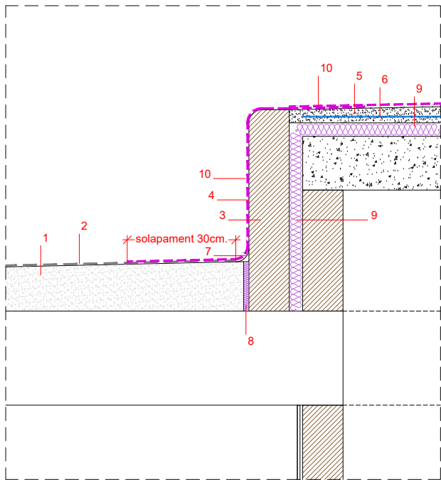
SECCIÓ CONSTRUCTIVA CV2 A3 1/20
