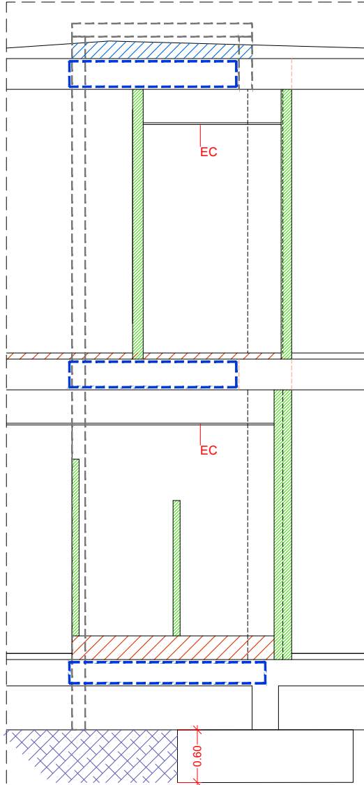
SECCIÓ L2
