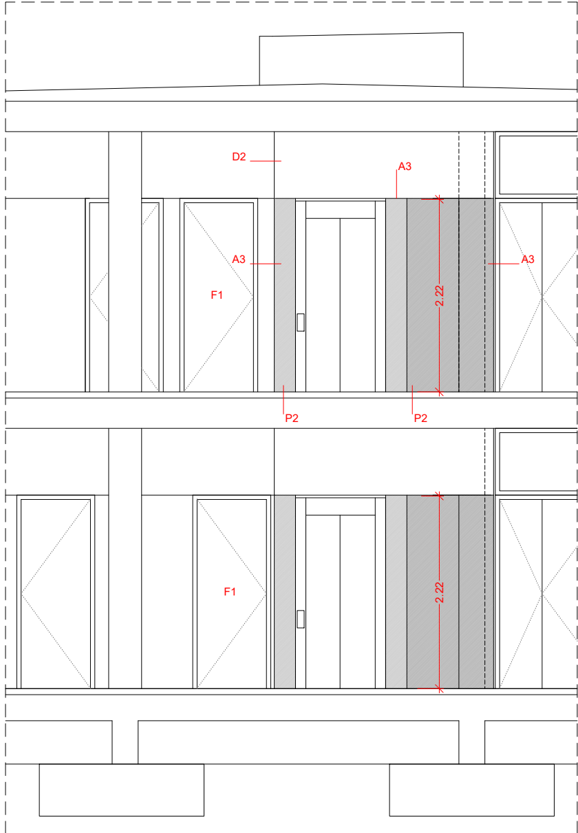
SECCIÓ T1
