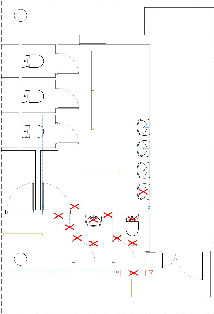
PLANTA PRIMERA
