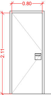
PORTA INTERIOR F1 2 UNITATS
