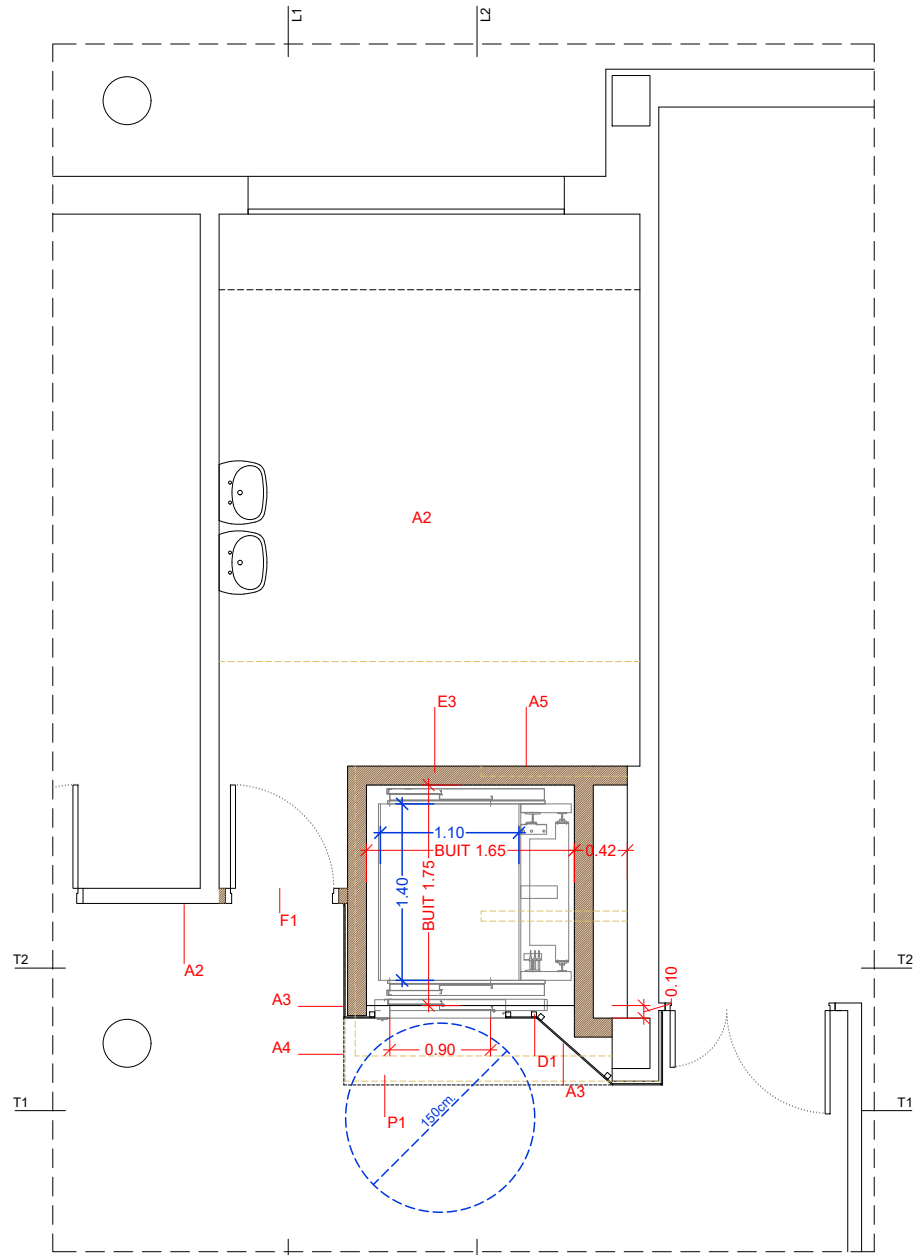
PLANTA BAIXA
