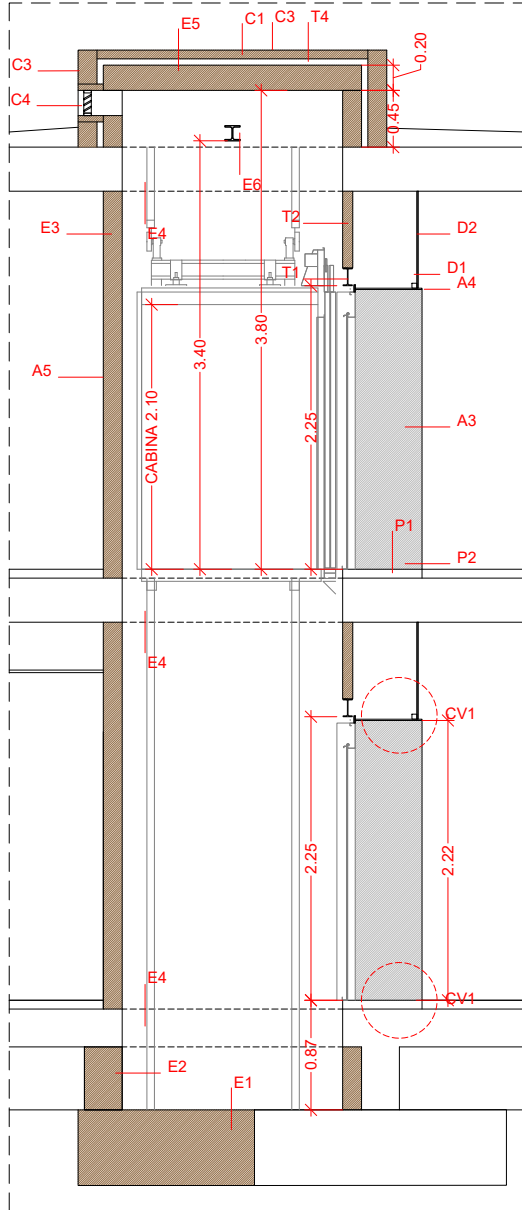
SECCIÓ L2
