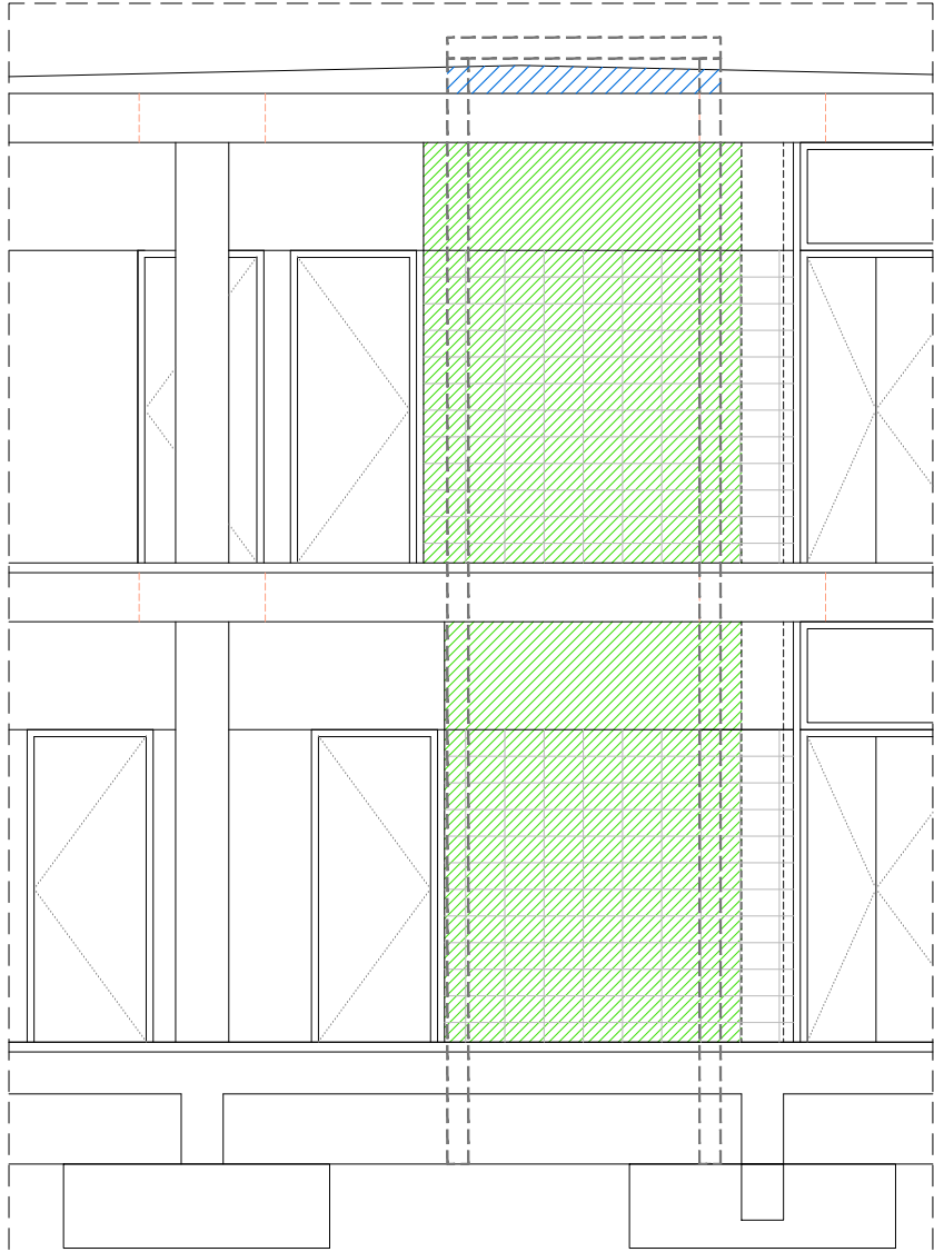
SECCIÓ T1
