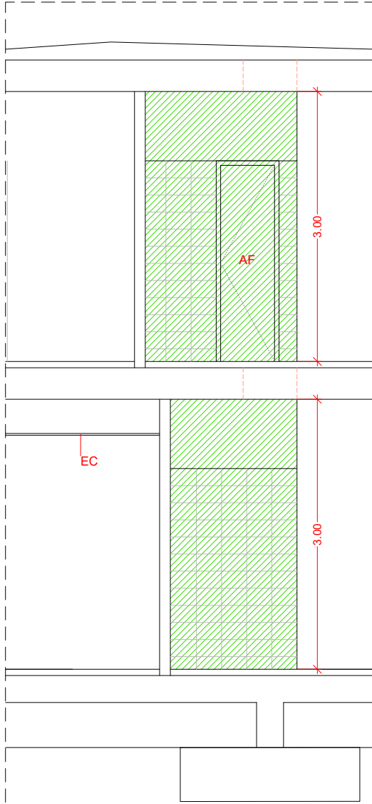
SECCIÓ L1
