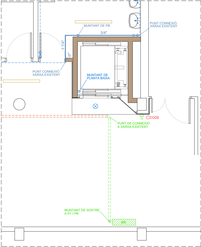
PLANTA PRIMERA
