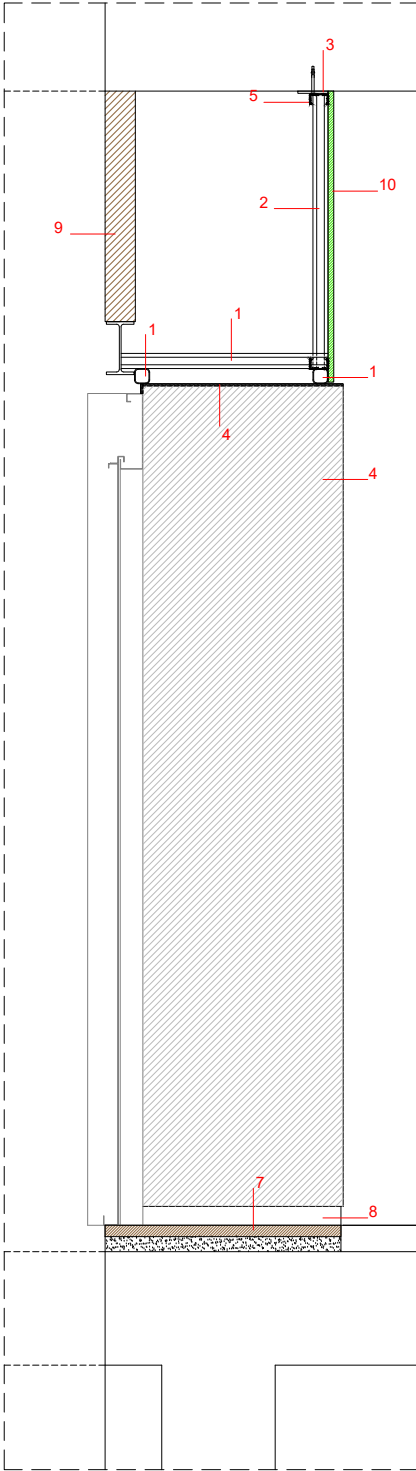
SECCIÓ CONSTRUCTIVA CV1 A3 1/20
