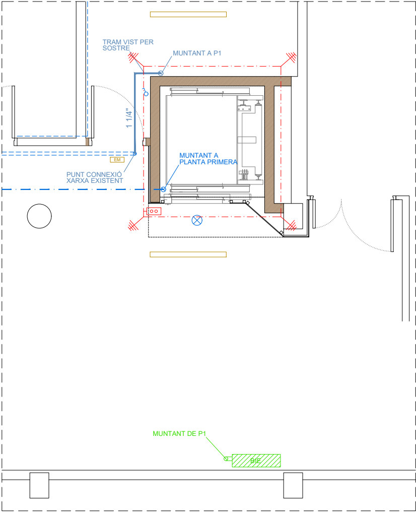
PLANTA BAIXA
