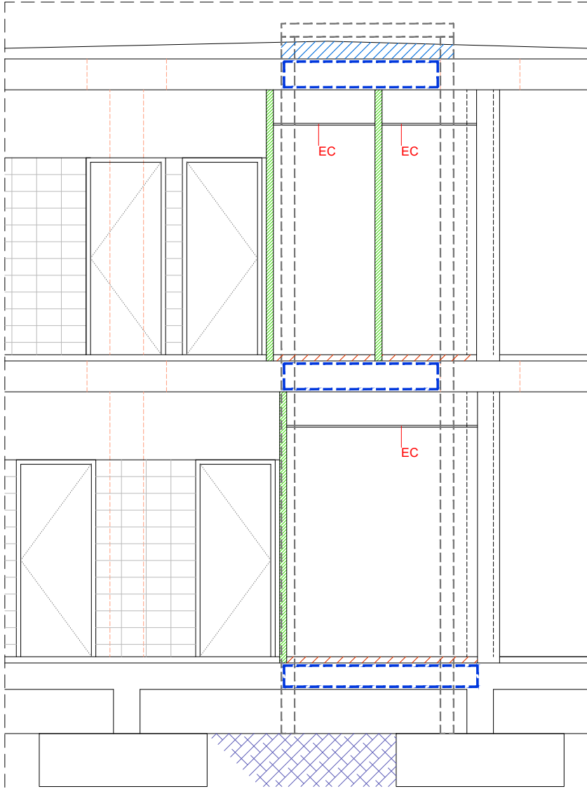
SECCIÓ T2
