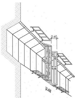
PROTECCIO A LES RASES
