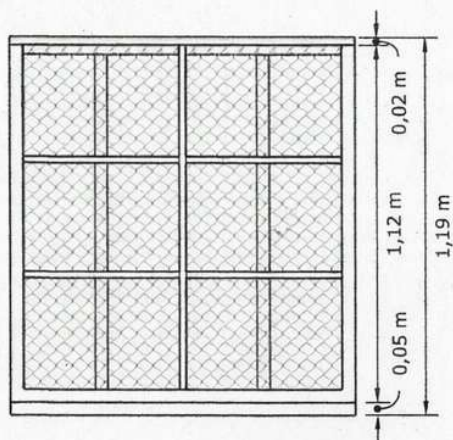
ALÇAT FRONTAL
