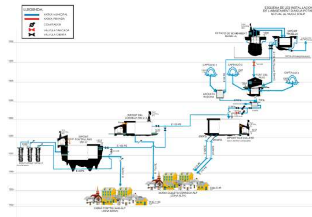
Imatge 2. Esquema hidràulic de la xarxa d'abastament d'Alp
