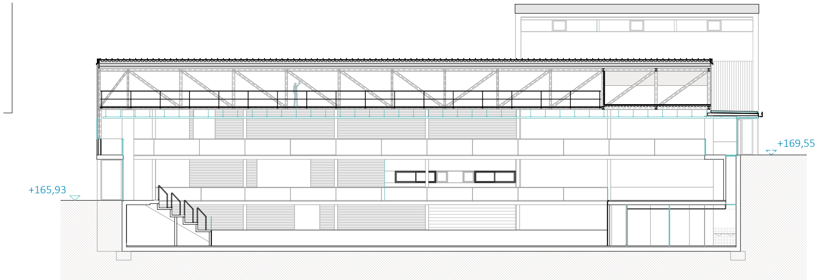
SECCIÓ TRANSVERSAL
