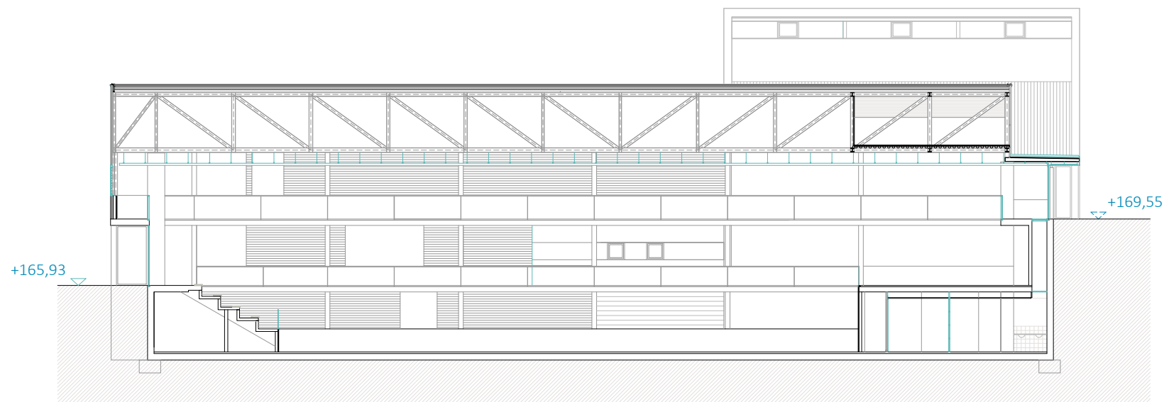
SECCIÓ TRANSVERSAL
