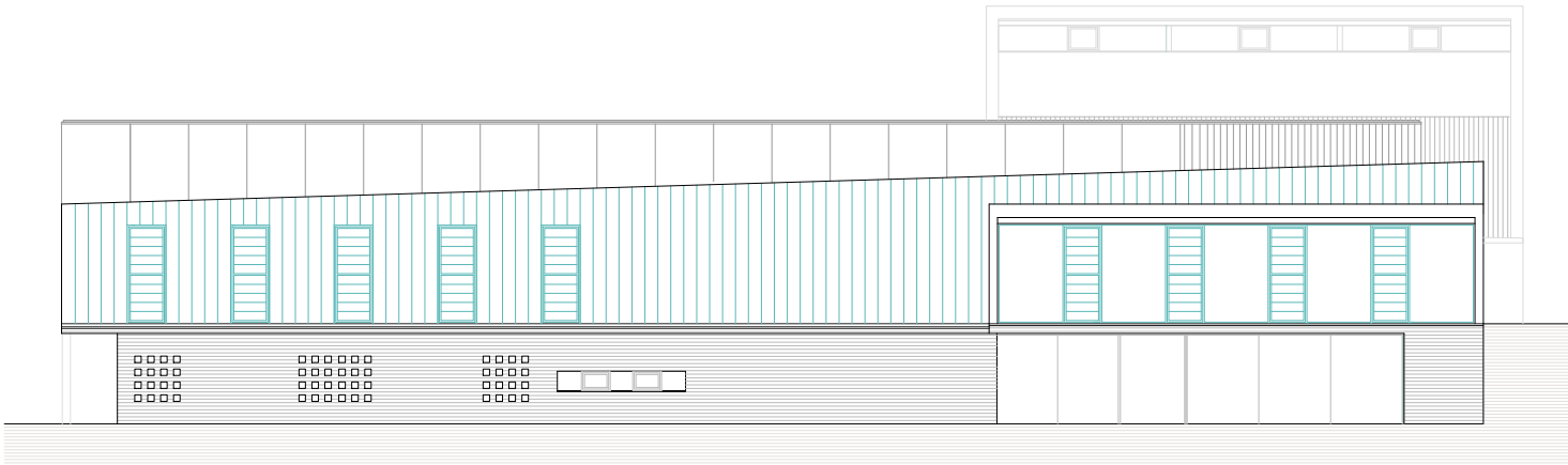
ALÇAT SUD
