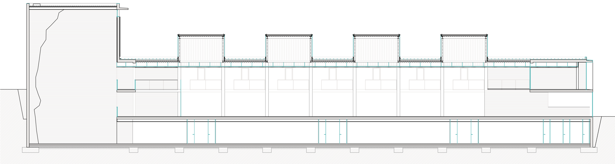
SECCIÓ LONGITUDINAL
