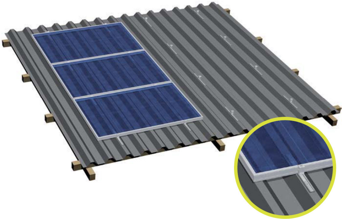
Fig. 6.3. Sistema de subjecció coplanar S-Flex.
