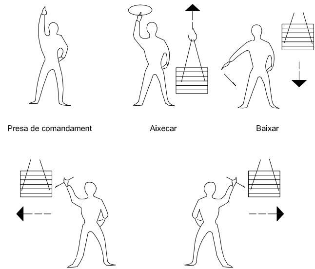
Desplaçaments laterals
