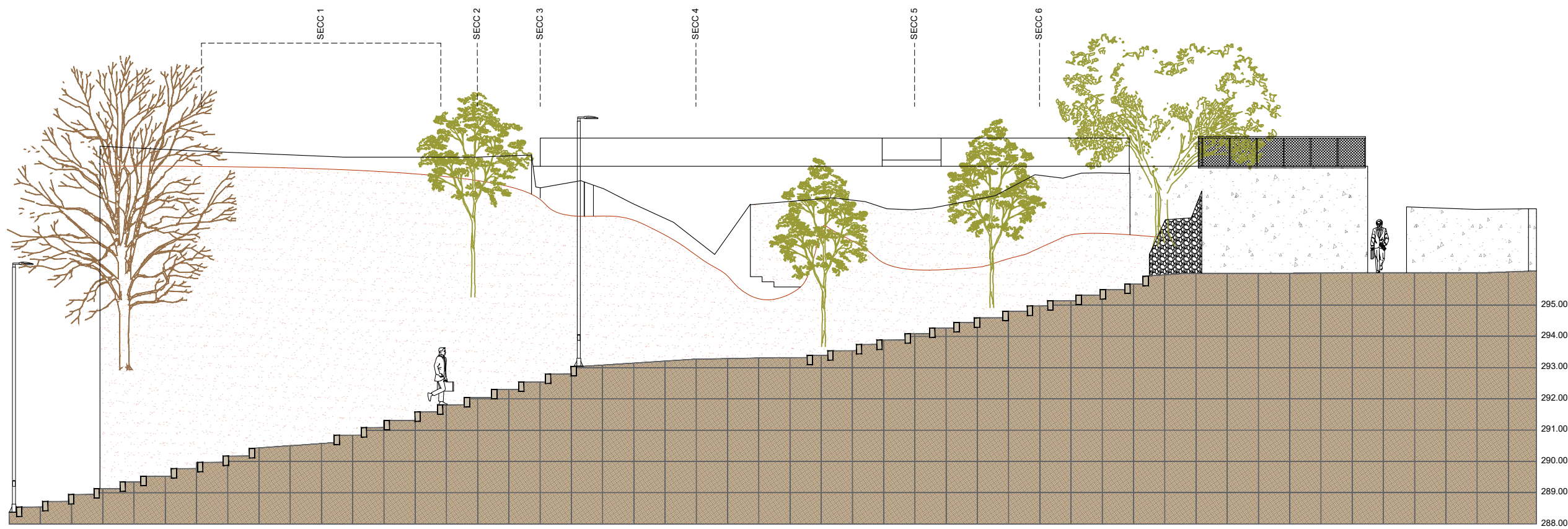
SECCIÓ LONGITUDINAL PLA EXTERIOR ESCALA
