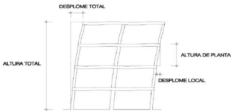
Figura 4.1 Desplomes
