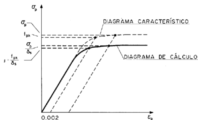
Diagrama tensió -deformació per a armadures actives
