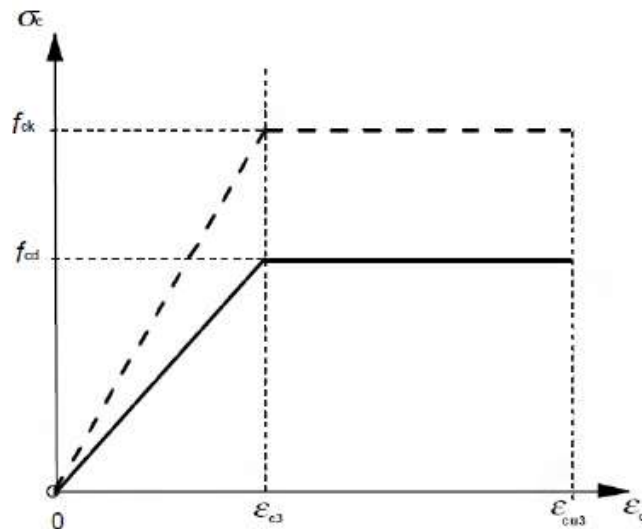
Figura A19.3.4 Diagrama tensió-deformación bilineal
