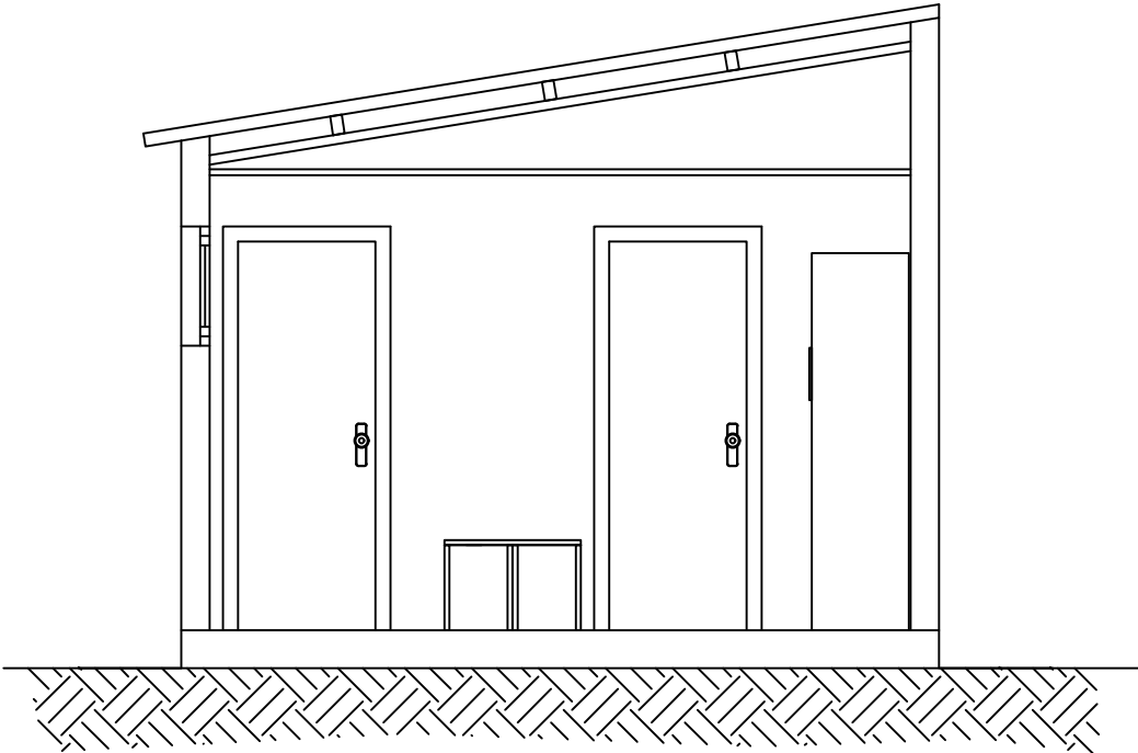
SECCIÓ A-B
