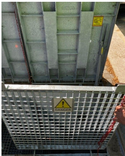
Fig. 1. Tapa d'accés a la sala d'equipaments, amb sistema de bloqueig a 90° i amb reixeta de seguretat.
