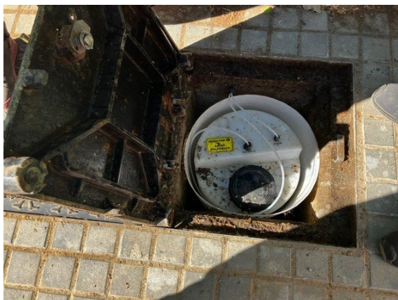
Fig. 4. Bidó amb sistema de recàrrega des de l'exterior de la sala de màquines (sempre que aquesta estigui soterrada a una profunditat superior als 1,5m), a través d'una arqueta antivandàlica.
