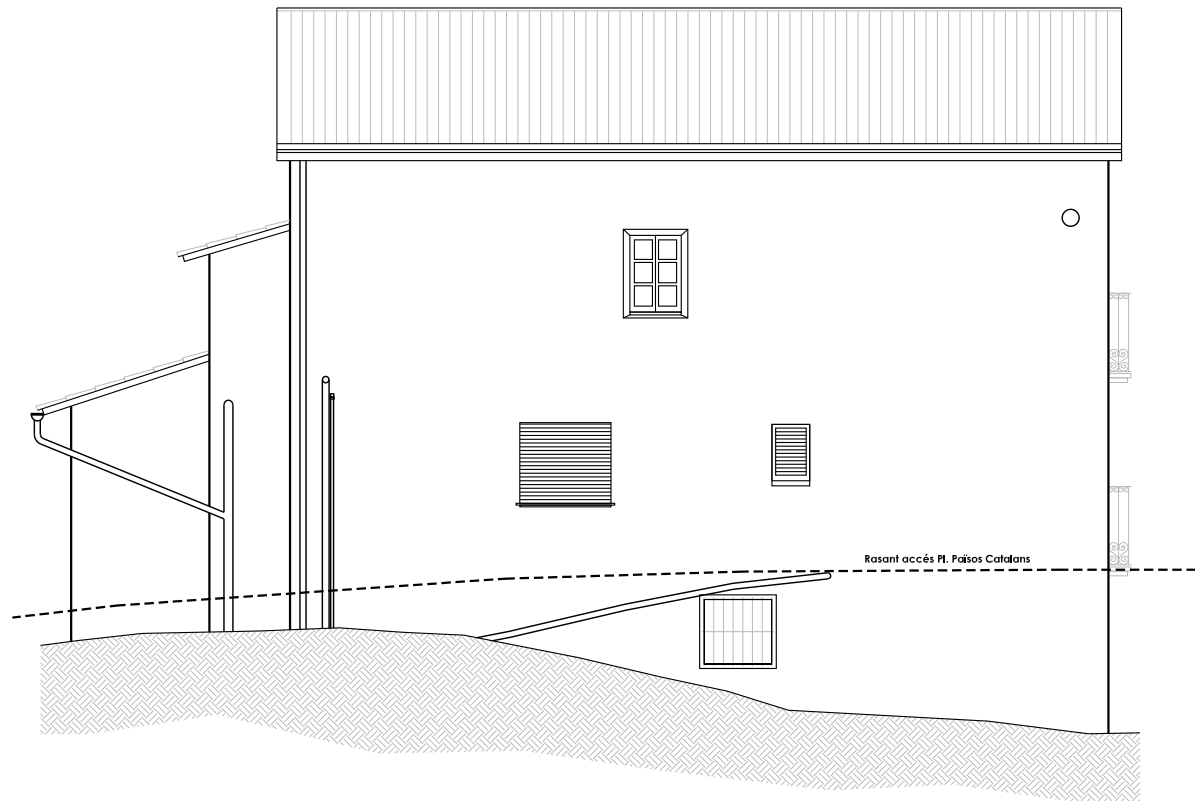
FAÇANA SUD OEST
