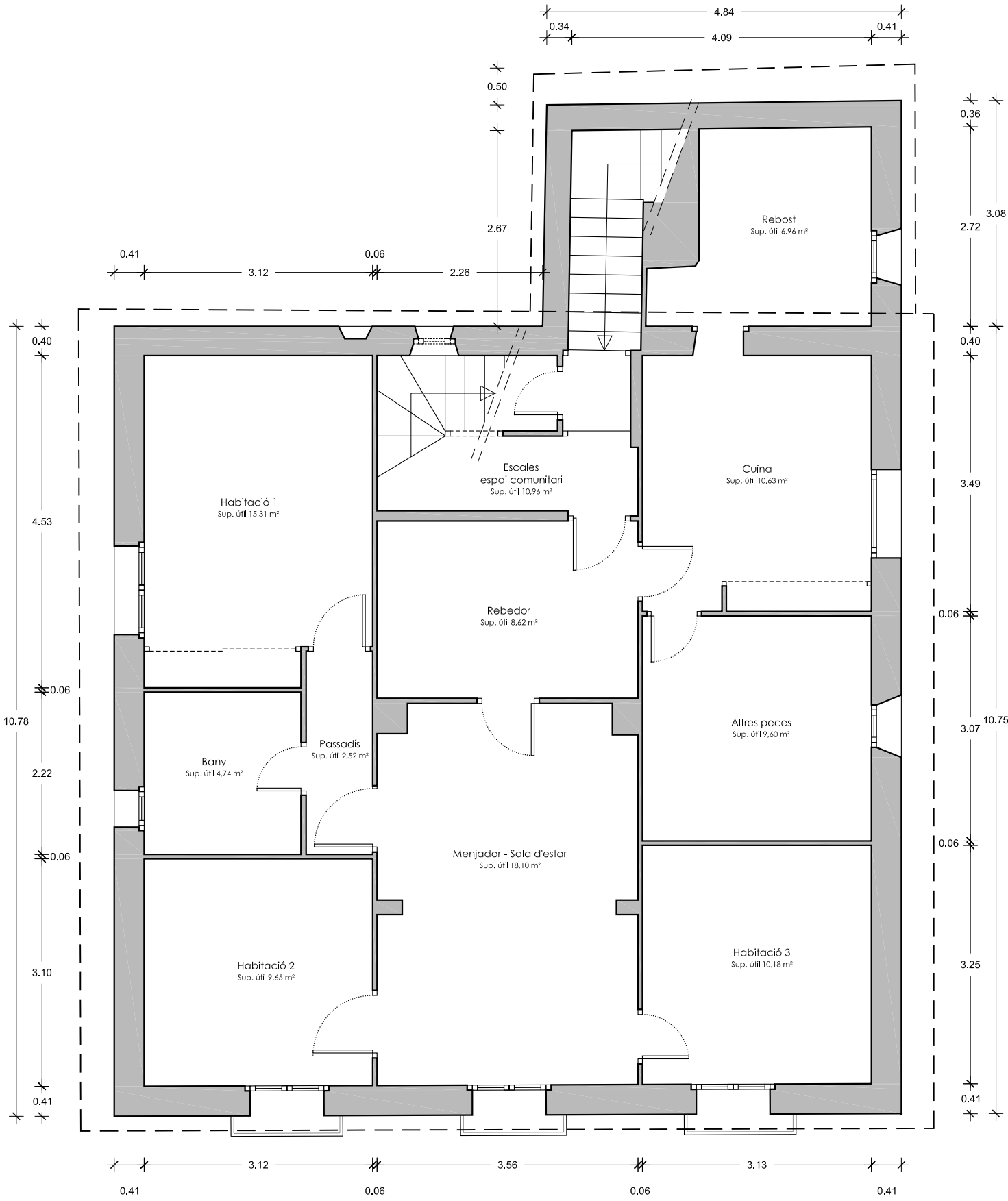
PLANTA SUPERIORS
