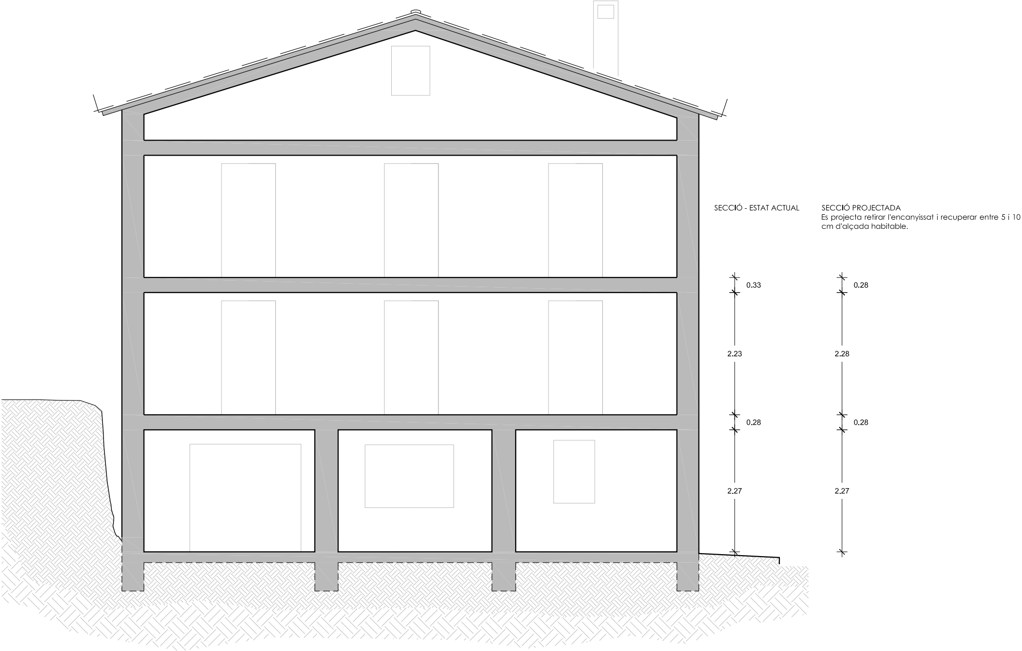
SECCIÓ ESTAT ACTUAL I PROJECTADA
