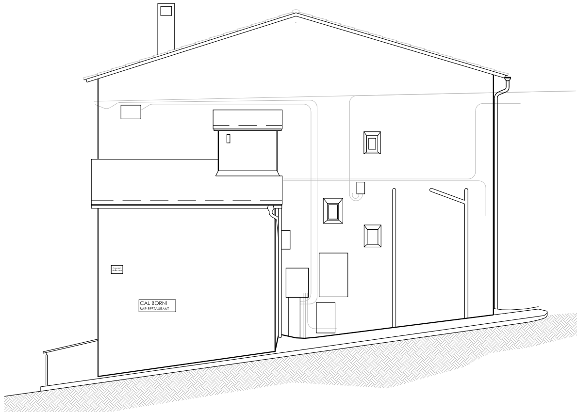
FAÇANA NORD OEST
