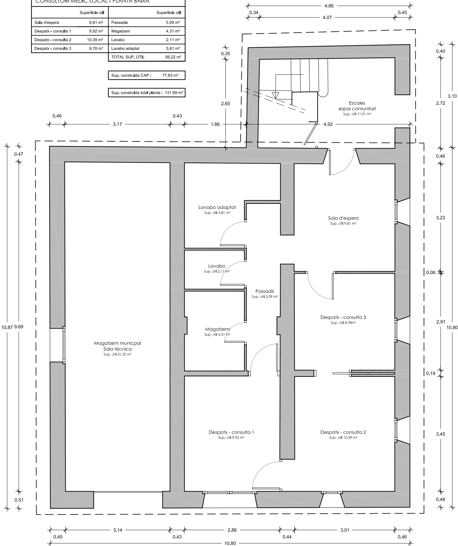
PLANTA BAIXA
