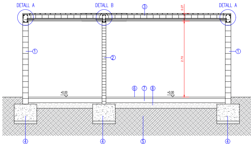
Secció A-A'
