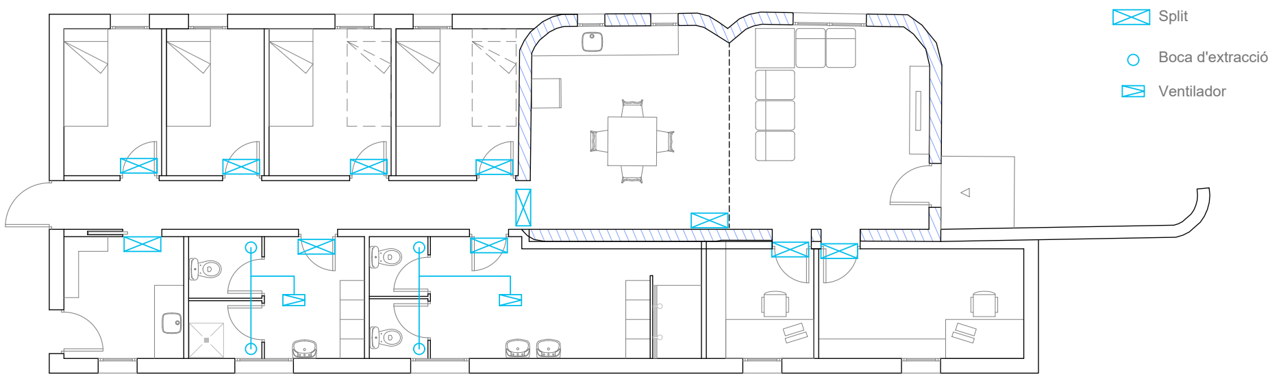
PLANTA CLIMA
