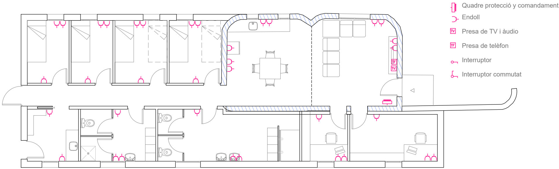
PLANTA ELECTRICITAT
