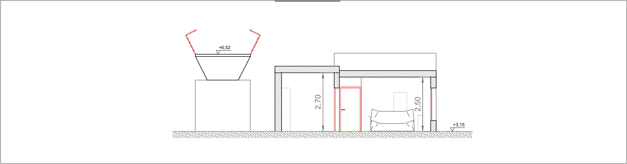
SECCIÓ C-C'
