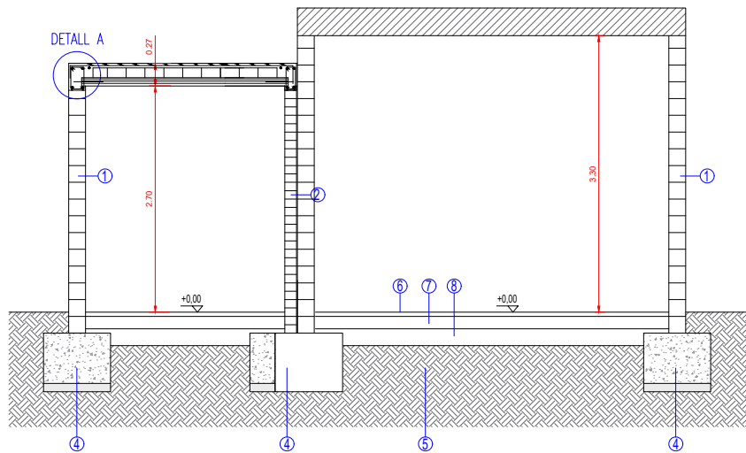
Secció B-B'
