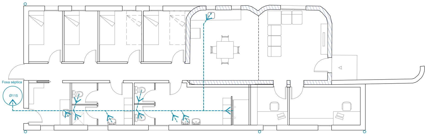
PLANTA SANEJAMENT
