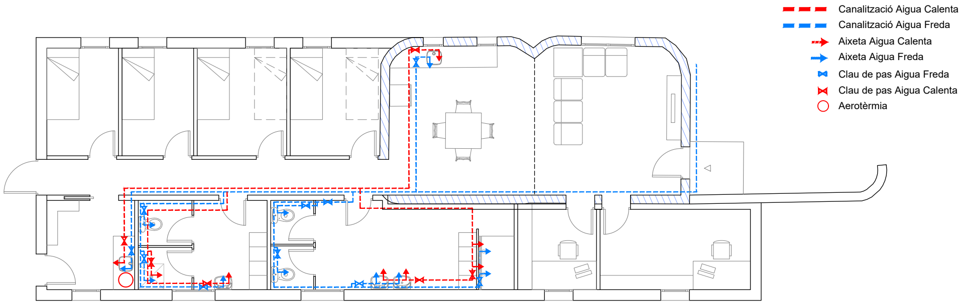
PLANTA FONTANERIA
