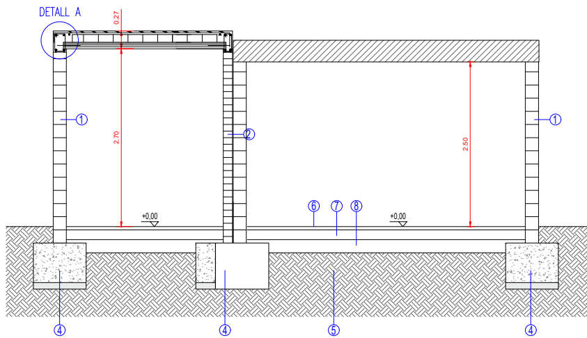
Secció C-C'
