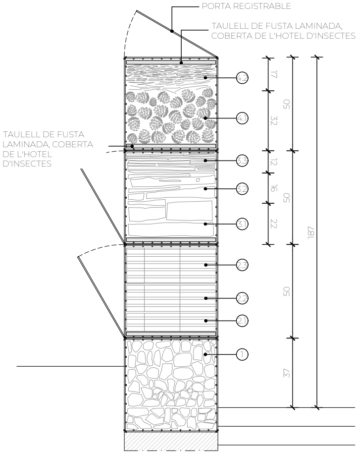
ST1 - DETALL MUR GABIÓ HOTEL D'INSECTES - E:1/20
