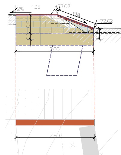
MUR 03.01
