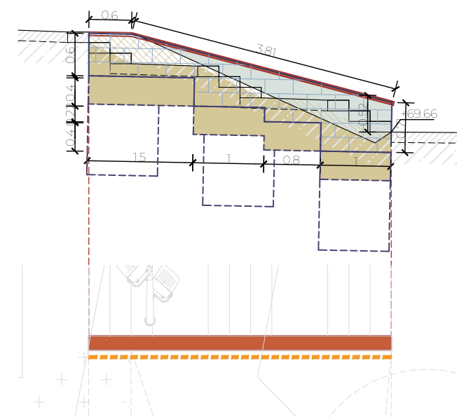
MUR 05.02
