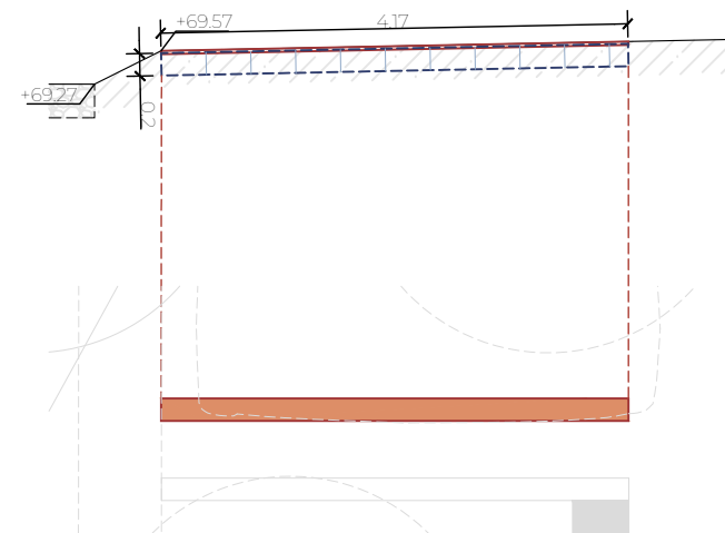
MUR 08.01
