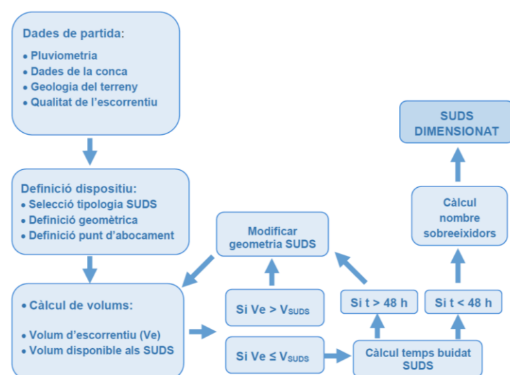
Figura 7. Passos a seguir pel dimensionament dels SUDS.
