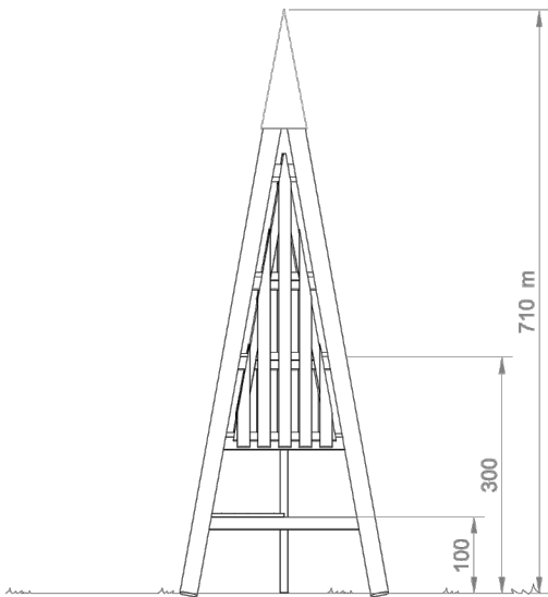
ALÇAT E:1/100
