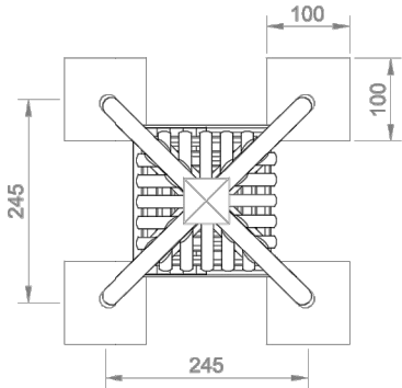
FONAMENTACIÓ E: 1/100
