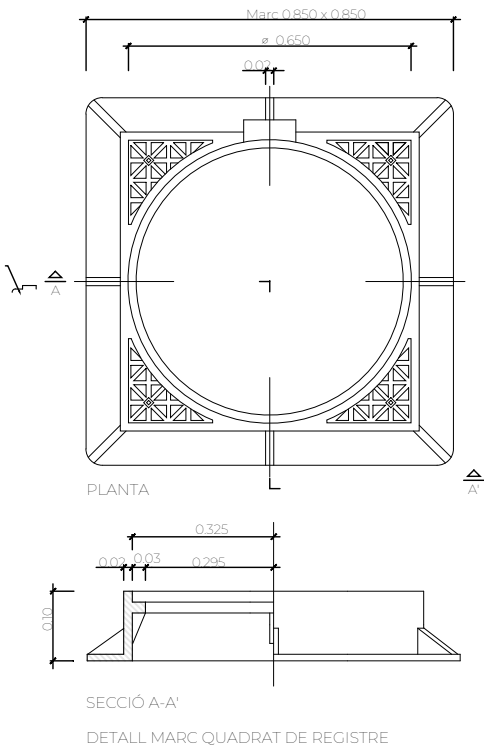
DETALL MARC QUADRAT DE REGISTRE
