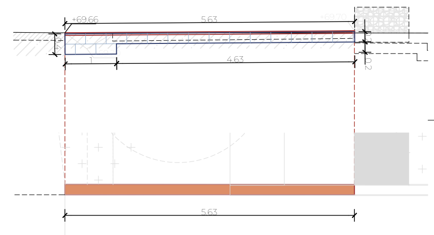
MUR 04.03
