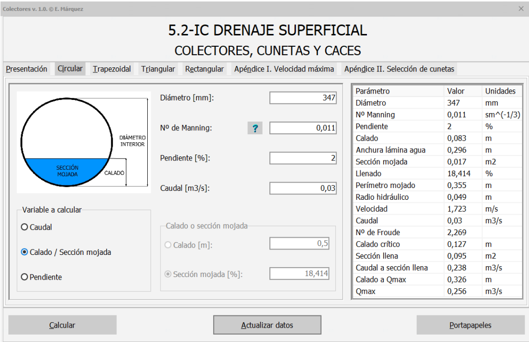
Figura 4. Resultats col·lector connexió av. d'en Piera
