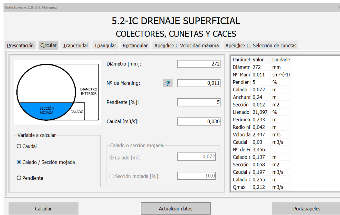
Figura 5. Resultats col·lector connexió travessa Carrancà
