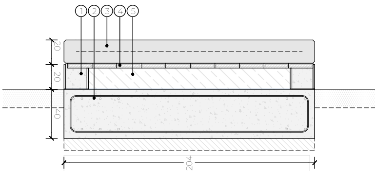
SECCIÓ TRANSVERSAL 2
