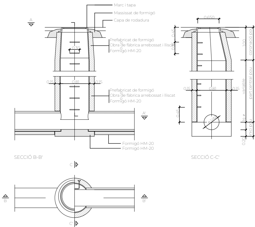
PLANTA, SECCIÓ A-A' NOTA: també poden ésser prefabricats
