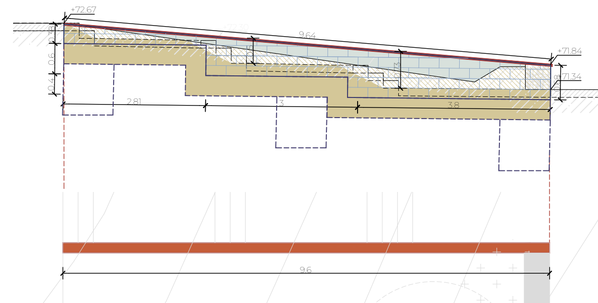
MUR 03.02
