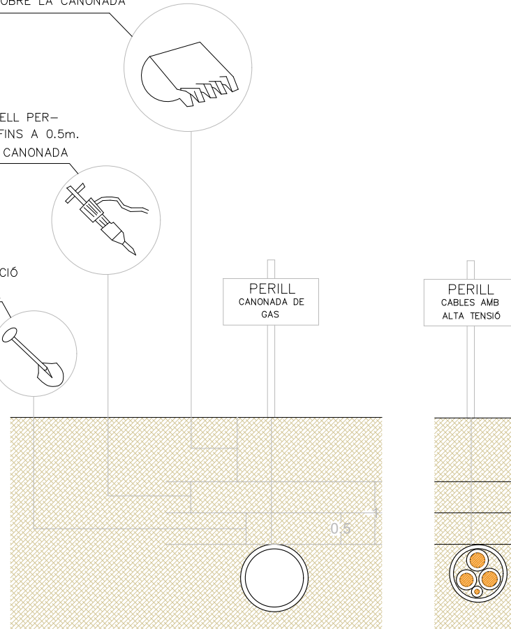
DISTÀNCIES DE SEGURITAT EN EXCAVACIÓ DE SERVEIS
