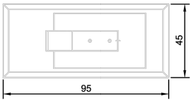
CIMENTACIÓN PREFABRICADA E:1/20
