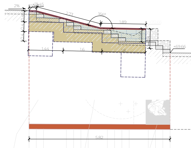
MUR 04.02
