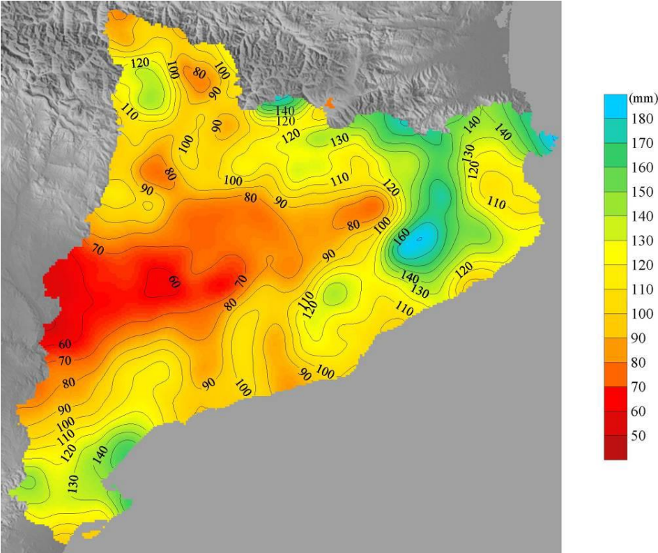
Figura 2. Precipitació màxima en un dia (en mm).
