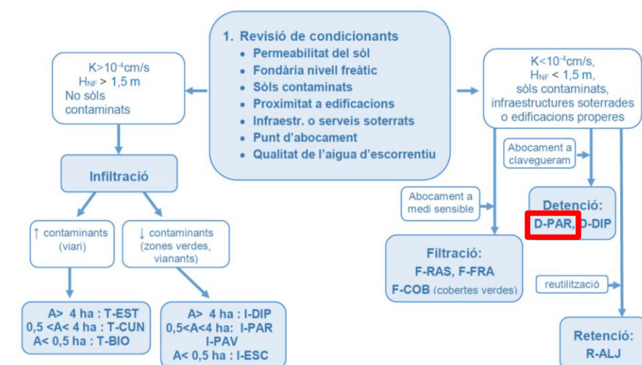
Figura 6. Diagrama de flux per la selecció de la tipologia de SUDS.
