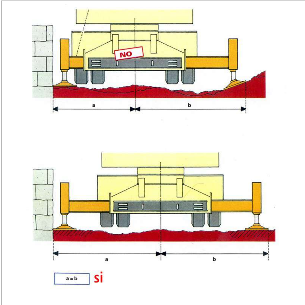
Col·locació estabilitzadors distàncies
