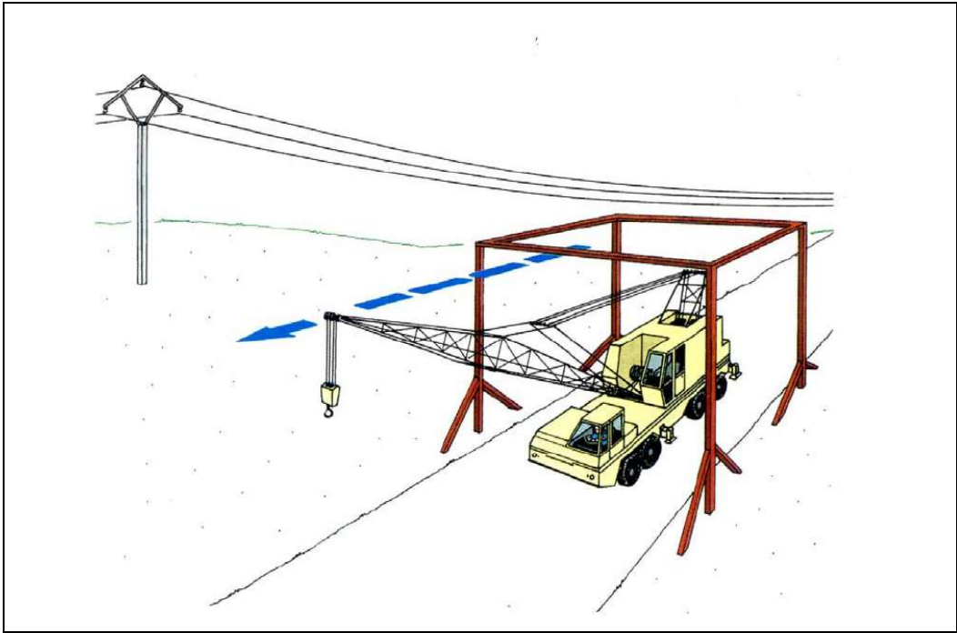
pas sota línies elèctriques perspectiva
