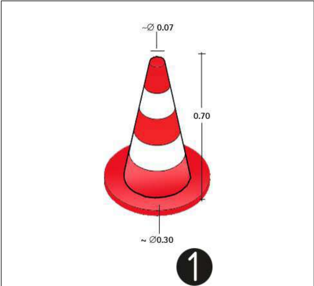
1.con de balissament
