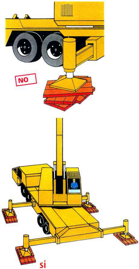
Col·locació estabilitzadors recolçaments
