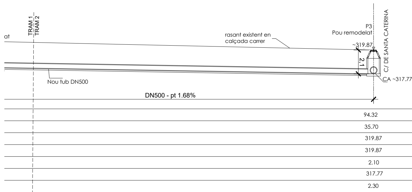
PERFIL LONGITUDINAL - TRAM 2 CARRER DE LA TORRE e. 1/200
