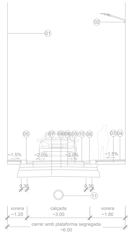
SECCIÓ TRANSVERSAL TIPUS e. 1/100
