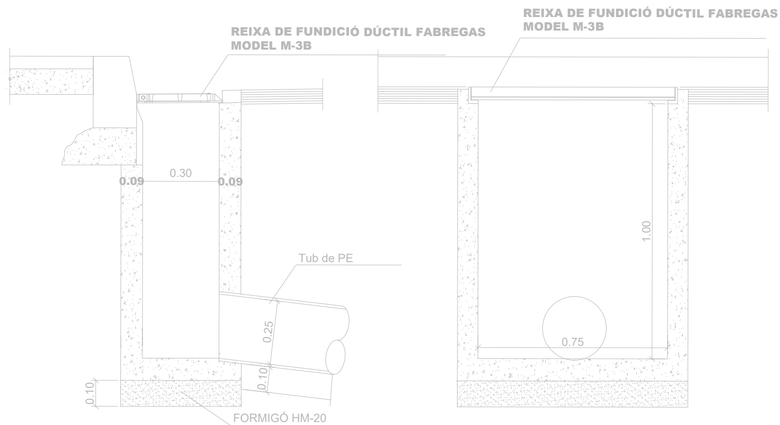
SECCIONS - DETALL EMBORNAL TIPUS e. 1/15
