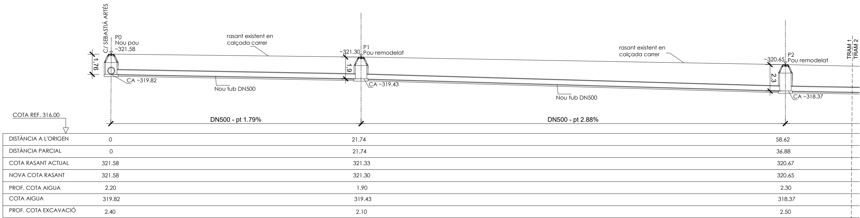
PERFIL LONGITUDINAL - TRAM 1 CARRER DE LA TORRE e. 1/200
