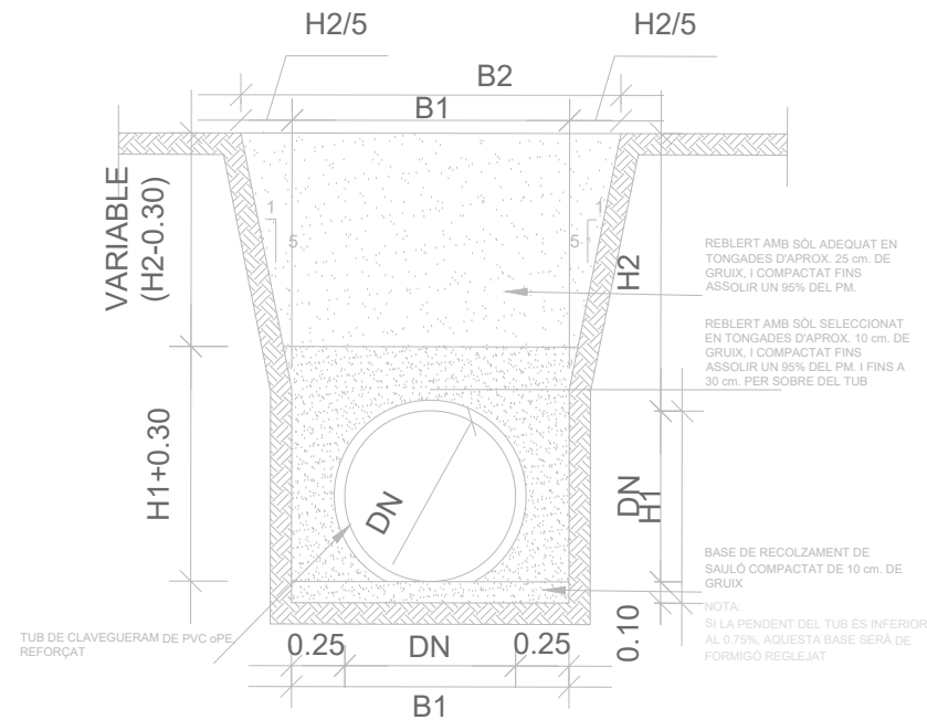
DETALL RASA TIPUS CLAVEGUERAM e. s/e
