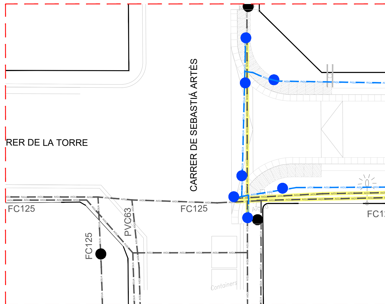
DETALL 1 AMPLIAT - ENCREUAMENT C/ TORRE AMB C/ DE SEBASTIÀ ARTÈS e. 1/100
