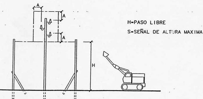
PORTICO DE BALIZAMIENTO DE LINEAS ELECTRICAS AEREAS
