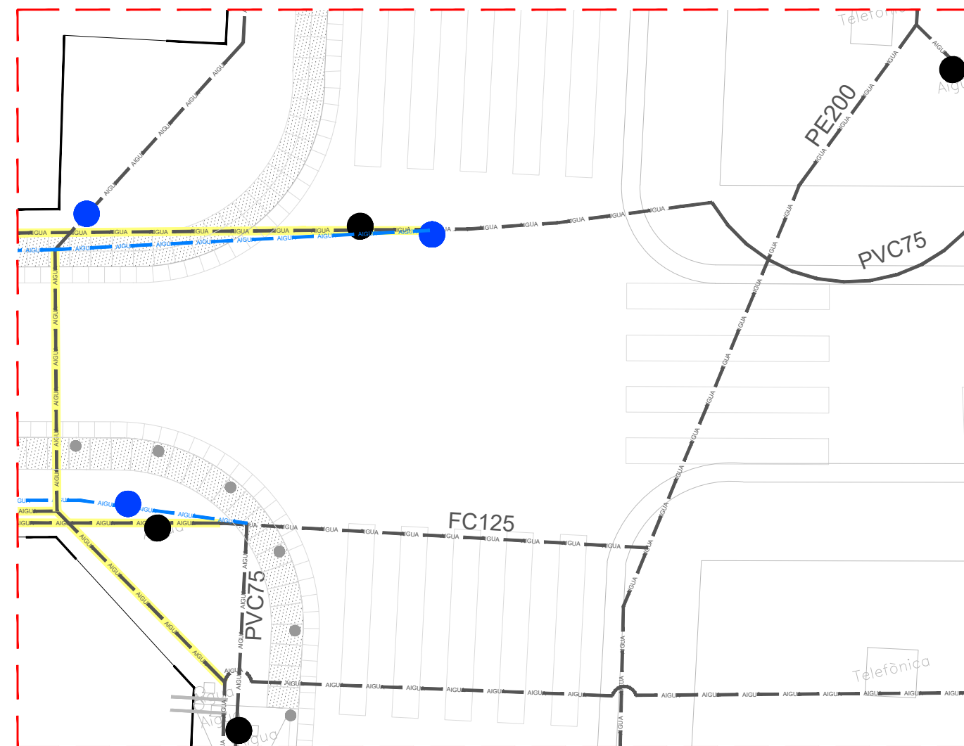
DETALL 2 AMPLIAT - ENCREUAMENT C/ TORRE AMB C/ SANT CATARINA e. 1/100
