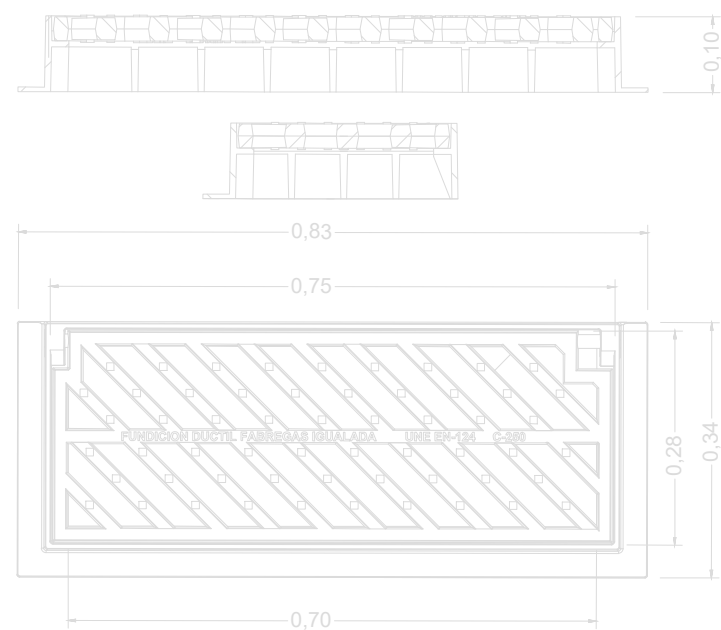
MARC I REIXA ABATIBLE TIPUS M-3B e. 1/10
