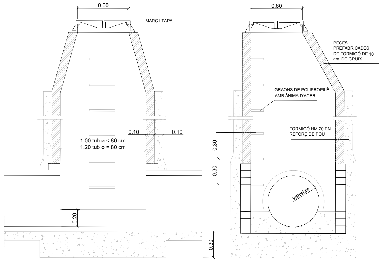
DETALLS POU DE REGISTRE TIPUS e. 1/25
