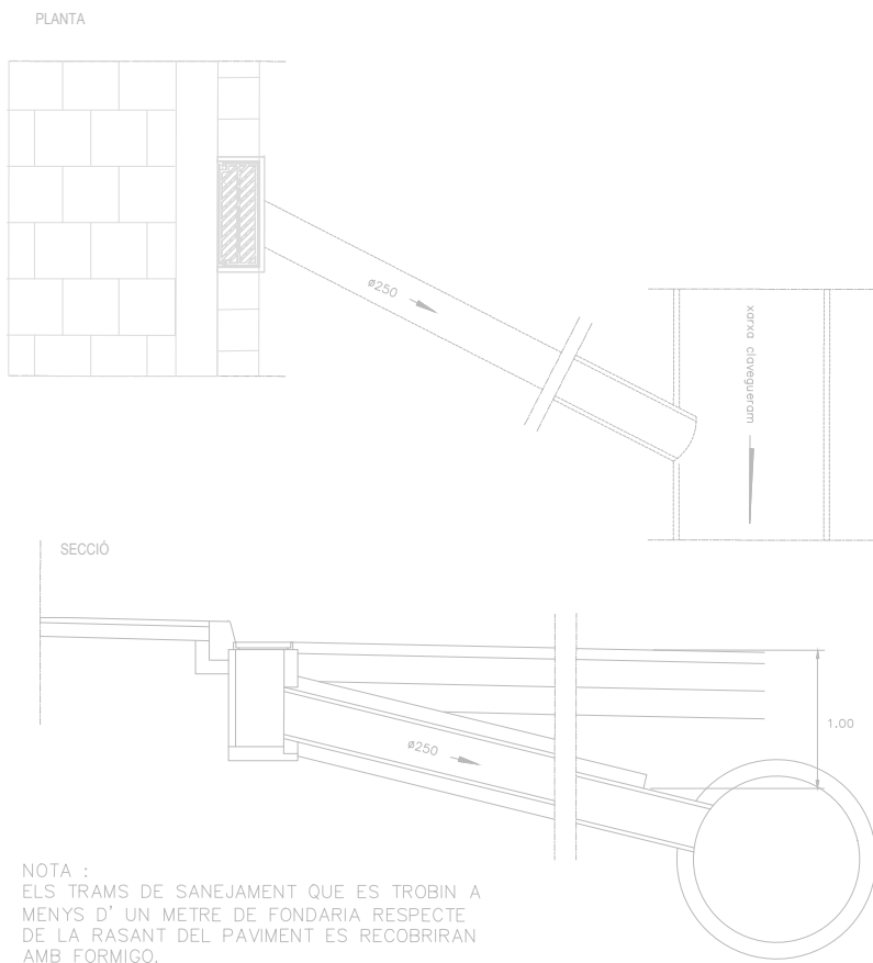
CONNEXIÓ EMBORNAL AL NOU COL·LECTOR e. s/e
