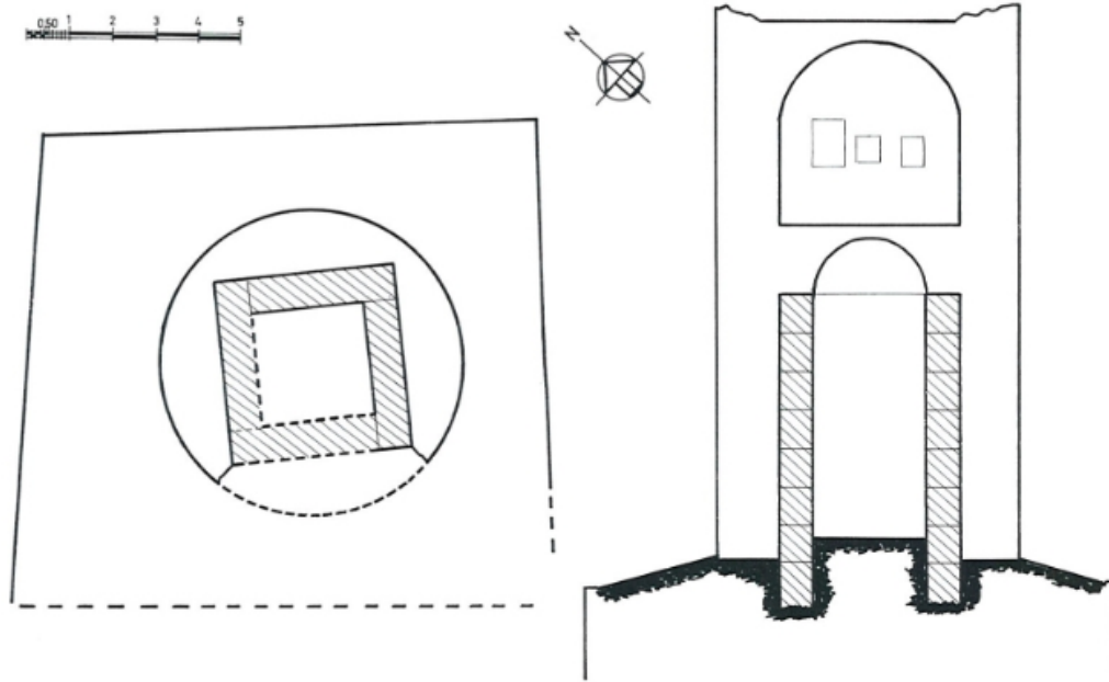
Planta i secció de la torre, amb la reconstrucció de la seva estructura
