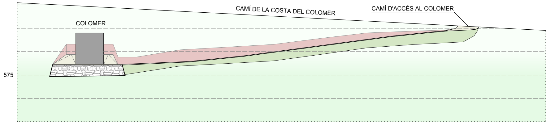
ALÇAT SUD CAMÍ D'ACCÉS AL COLOMER
