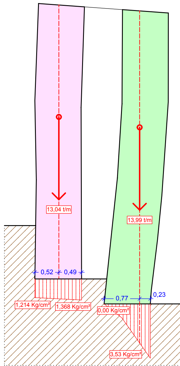
SECCIÓ A-A'
