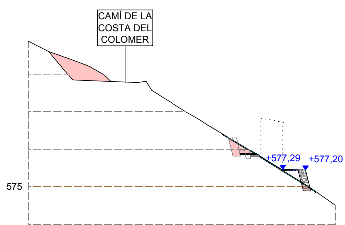
SECCIÓ 3
