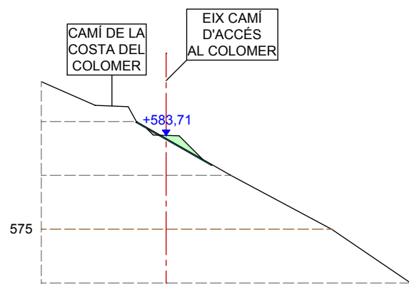
SECCIÓ 10
