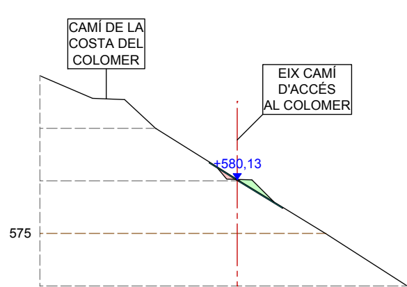
SECCIÓ 7
