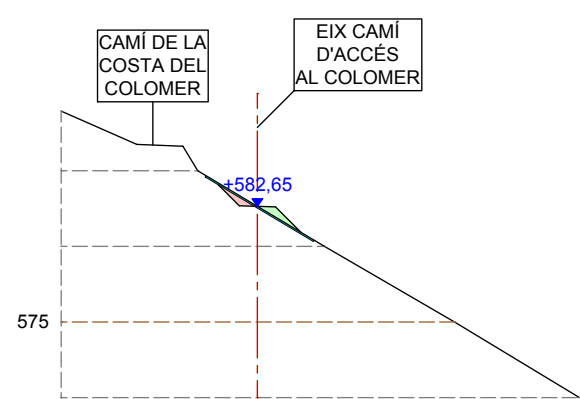
SECCIÓ 9
