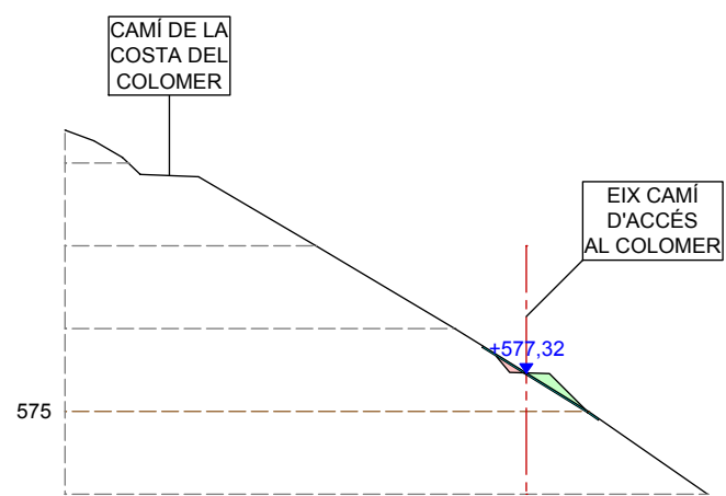
SECCIÓ 4
