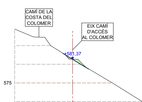
SECCIÓ 8
