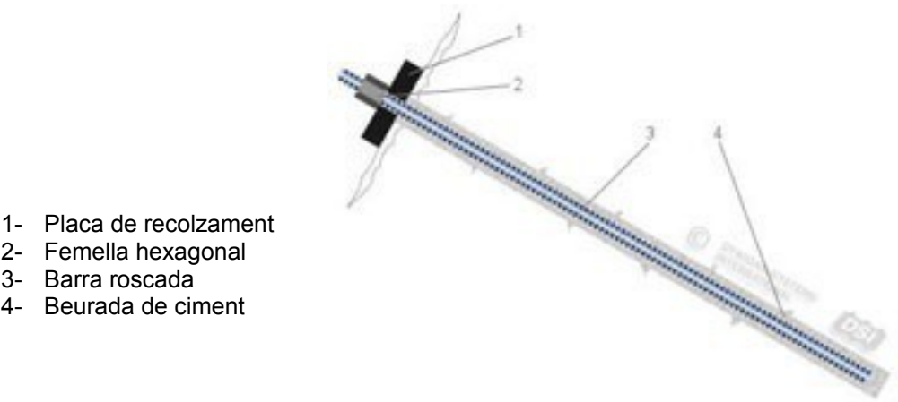
Figura 1: Esquema d'ancoratge Gewi tipus SN
