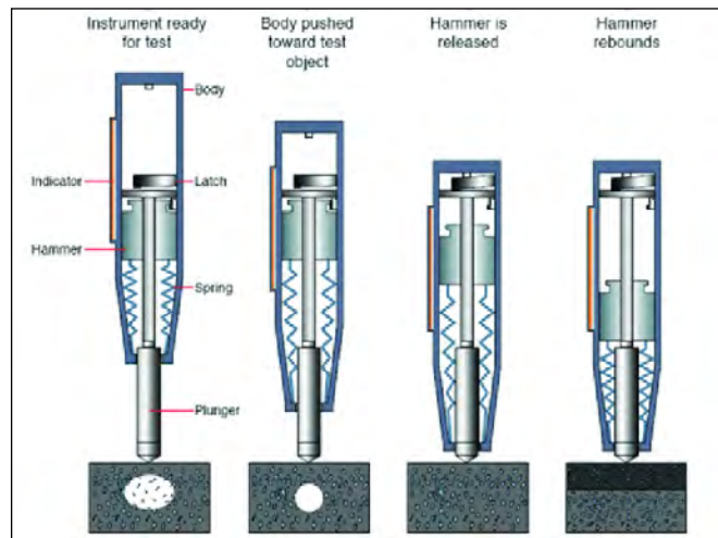
Figura 4. Esquema del funcionament del martell de Schmidt.
