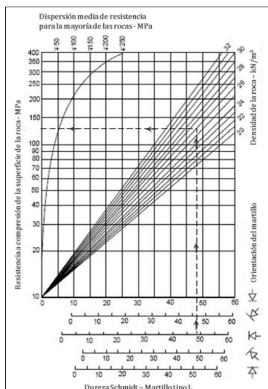
Figura 5. Gràfic de correlació pel martell de Schmidt entre resistència a la compressió, densitat de la roca i el rebot (Miller, 1965).
