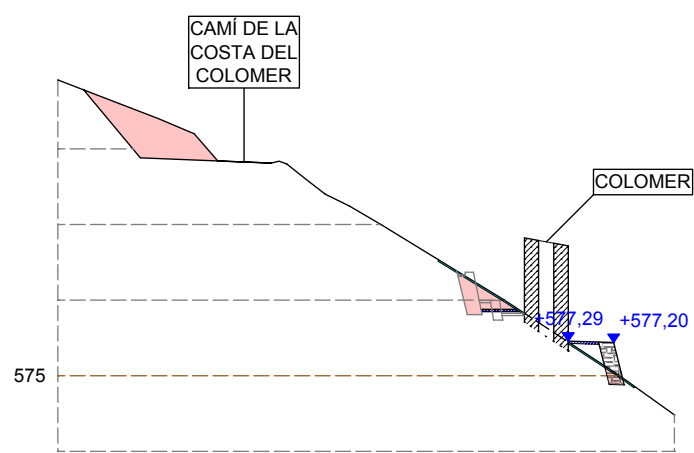
SECCIÓ 2
