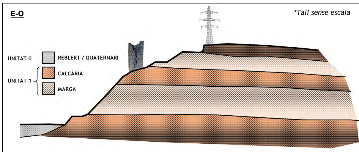
Figura 8. Tall interpretatiu dels materials que afloren en la zona d'estudi
