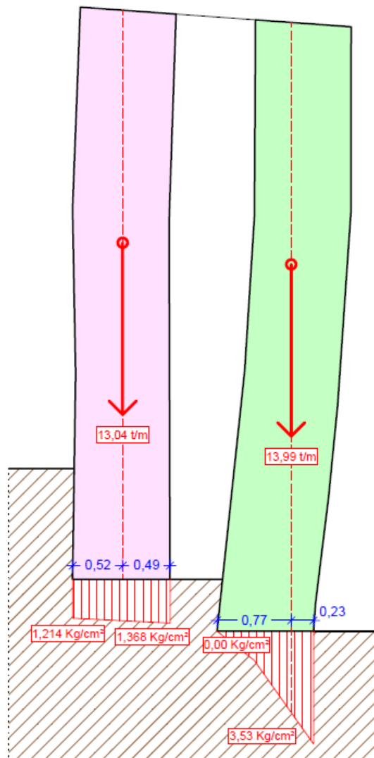
SECCIÓ A-A'
