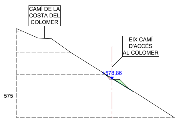
SECCIÓ 6
