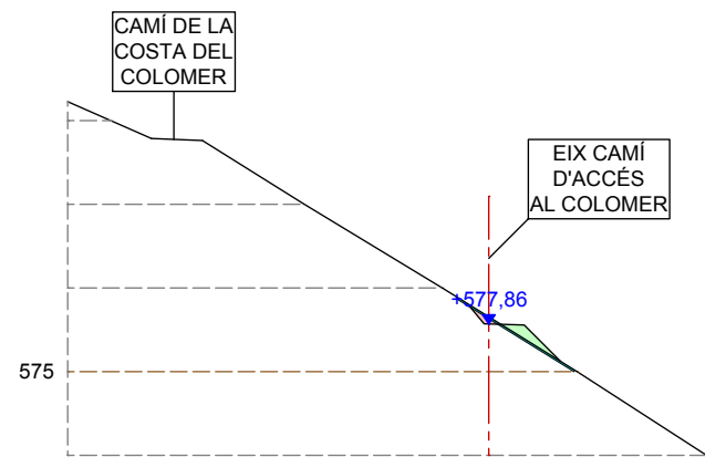
SECCIÓ 5
