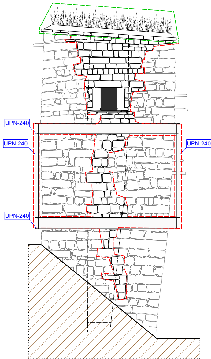
ALÇAT OEST
