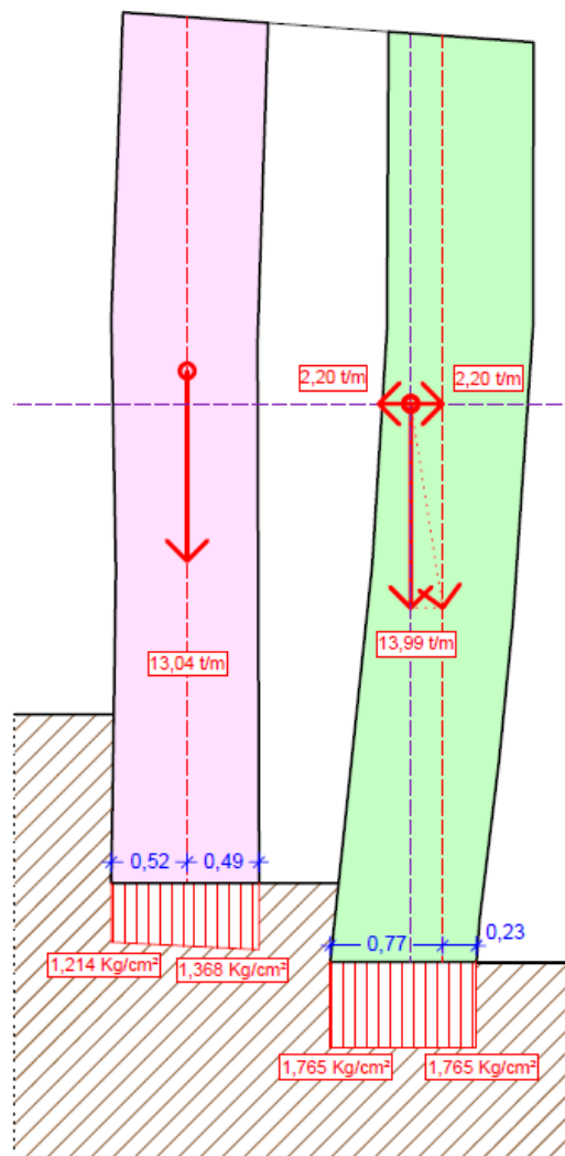
Secció A-A Descens de càrregues amb compensació del component horitzontal per corregir vinclament.
