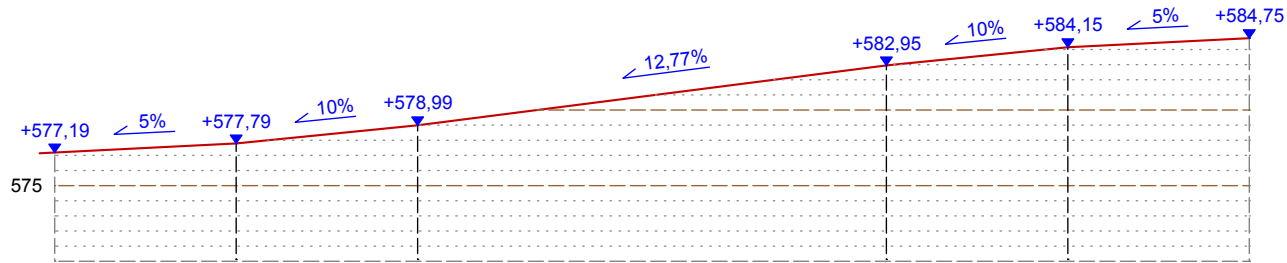
SECCIÓ LONGITUDINAL DEL CAMÍ D'ACCÉS
