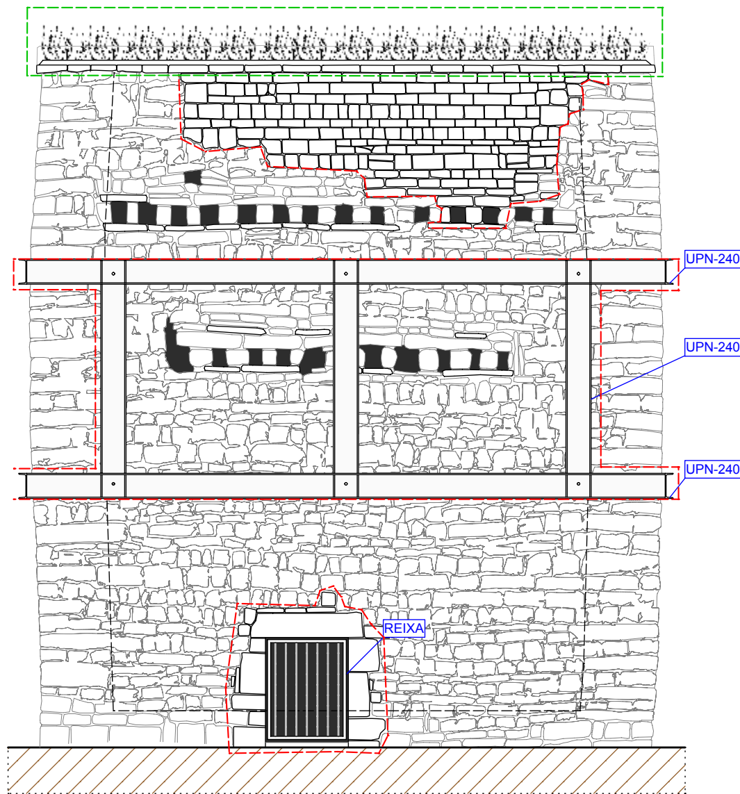
ALÇAT SUD
