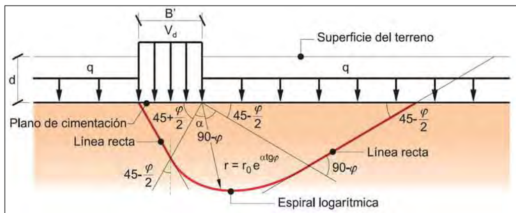
Figura 10. Distribució d'esforços en les formulacions principals considerades
