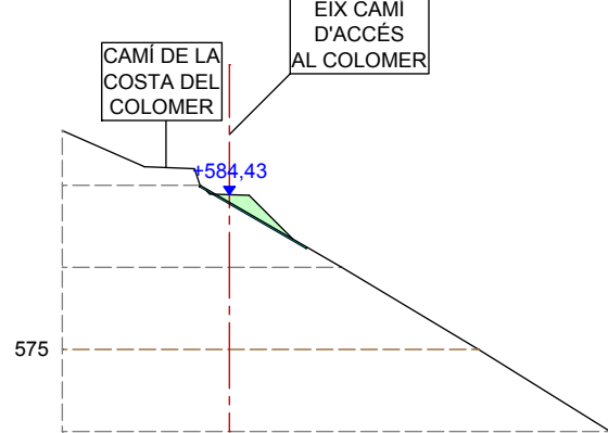
SECCIÓ 11
