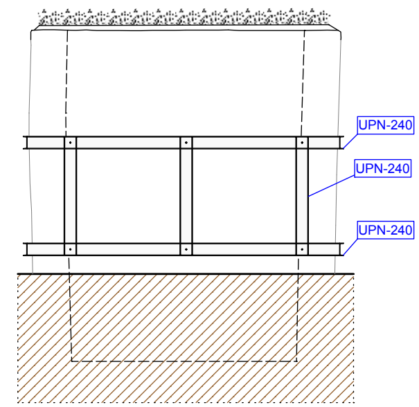
ALÇAT NORD (E: 1/100)
