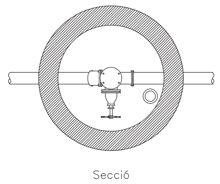
ARQUETA AMB VENTOSA
