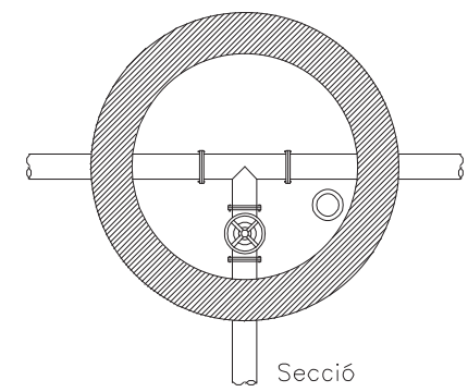
ARQUETA AMB VÀLVULA DE DESGUÀS
