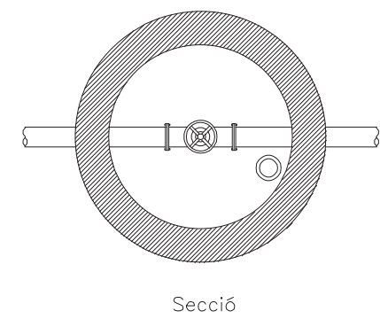
ARQUETA AMB CLAU DE PAS
