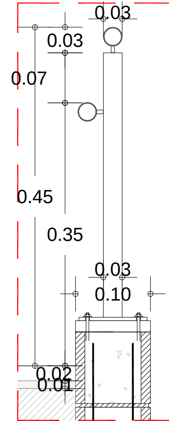
DETALL BARANA AMB PASSAMA E:1/10
