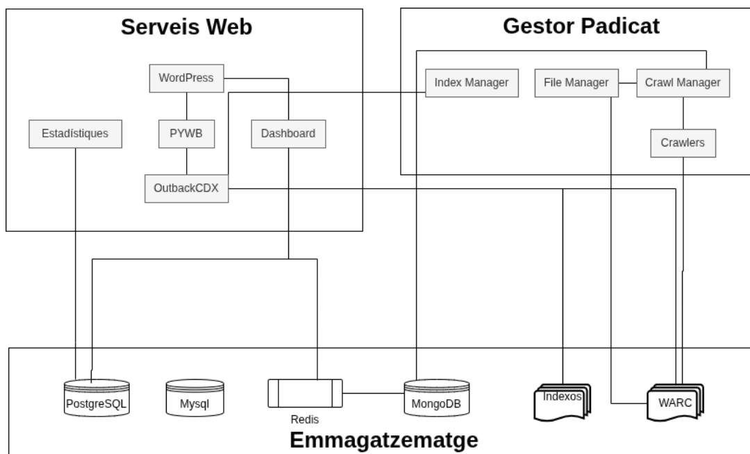
Fig.1 Esquema de l'arquitectura
