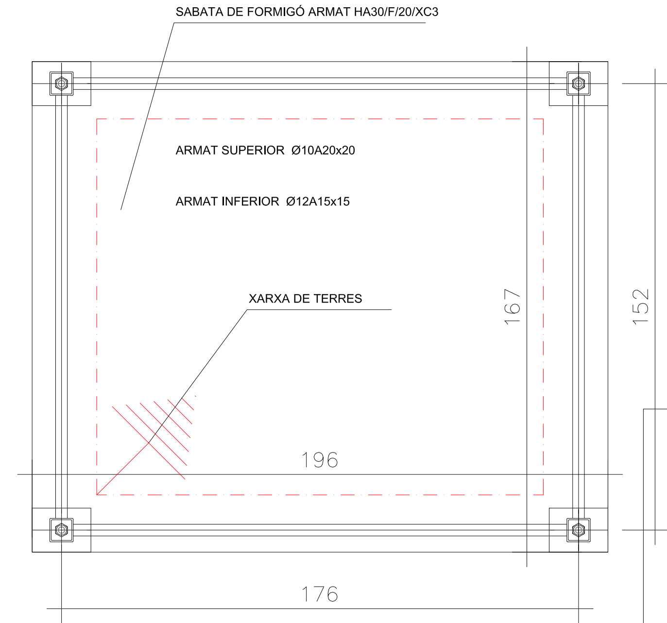
ESTRUCTURA CAIXA ASCENSOR - PLANTA
