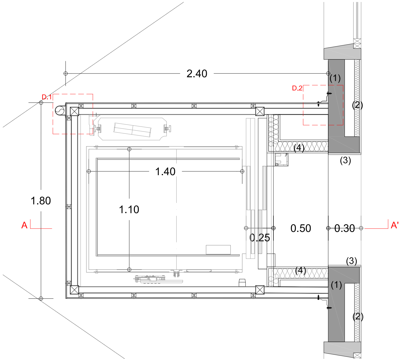
PLANTA PRIMERA: ASCENSOR e 1/20
