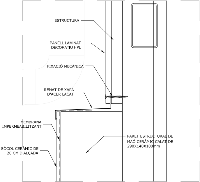
Detall 4: Sòcol panell HPL - Secció e.1/5
