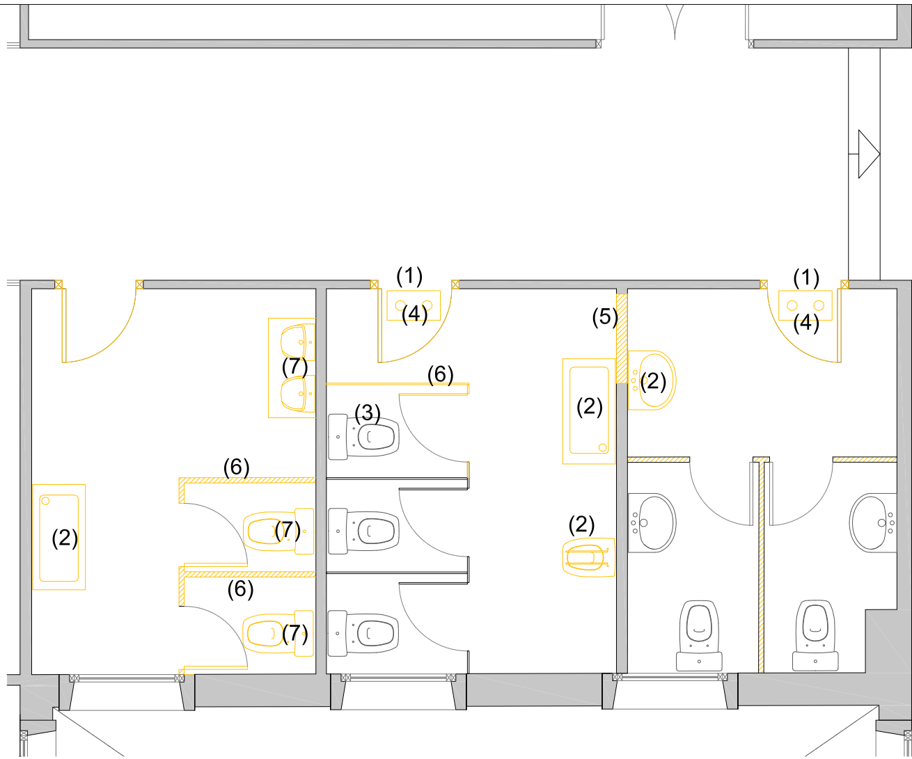
PLANTA PRIMERA - ESTAT ACTUAL
