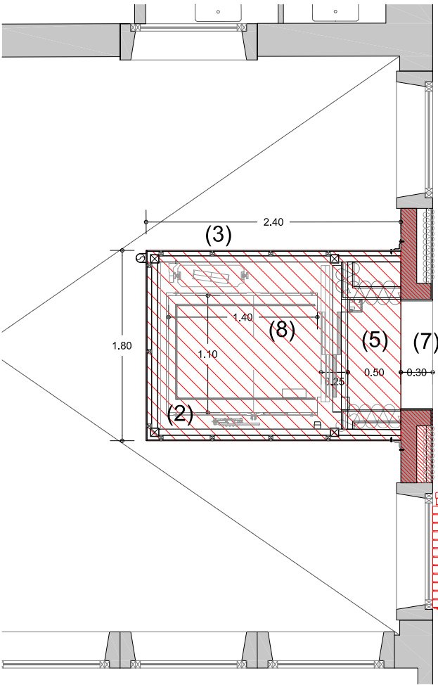
PLANTA PRIMERA PROPOSTA
