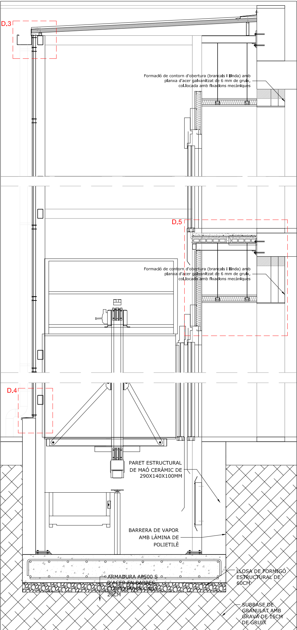
SECCIÓ A-A' e.1/25
