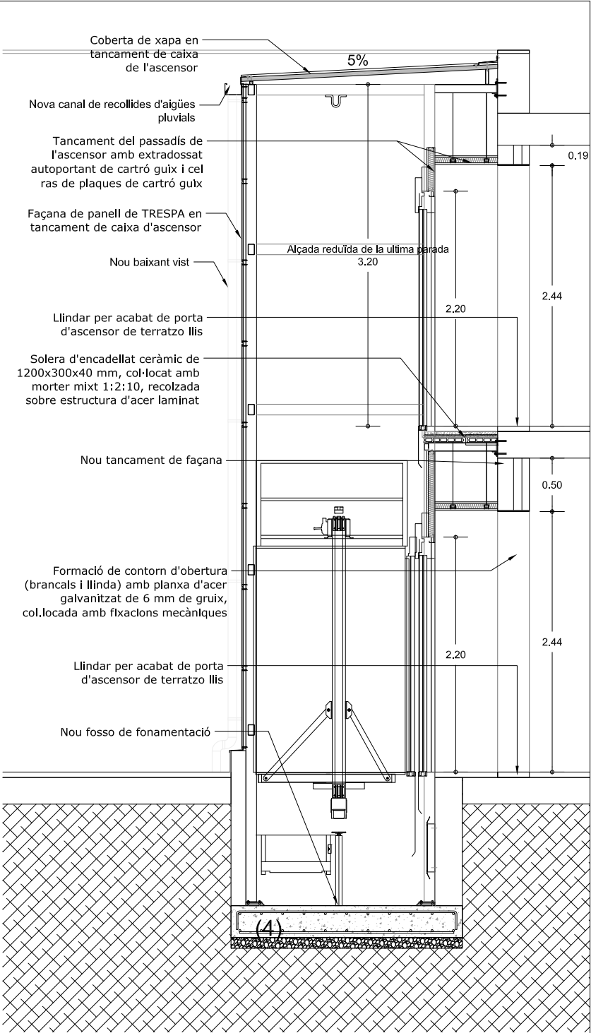
SECCIÓ A-A'
