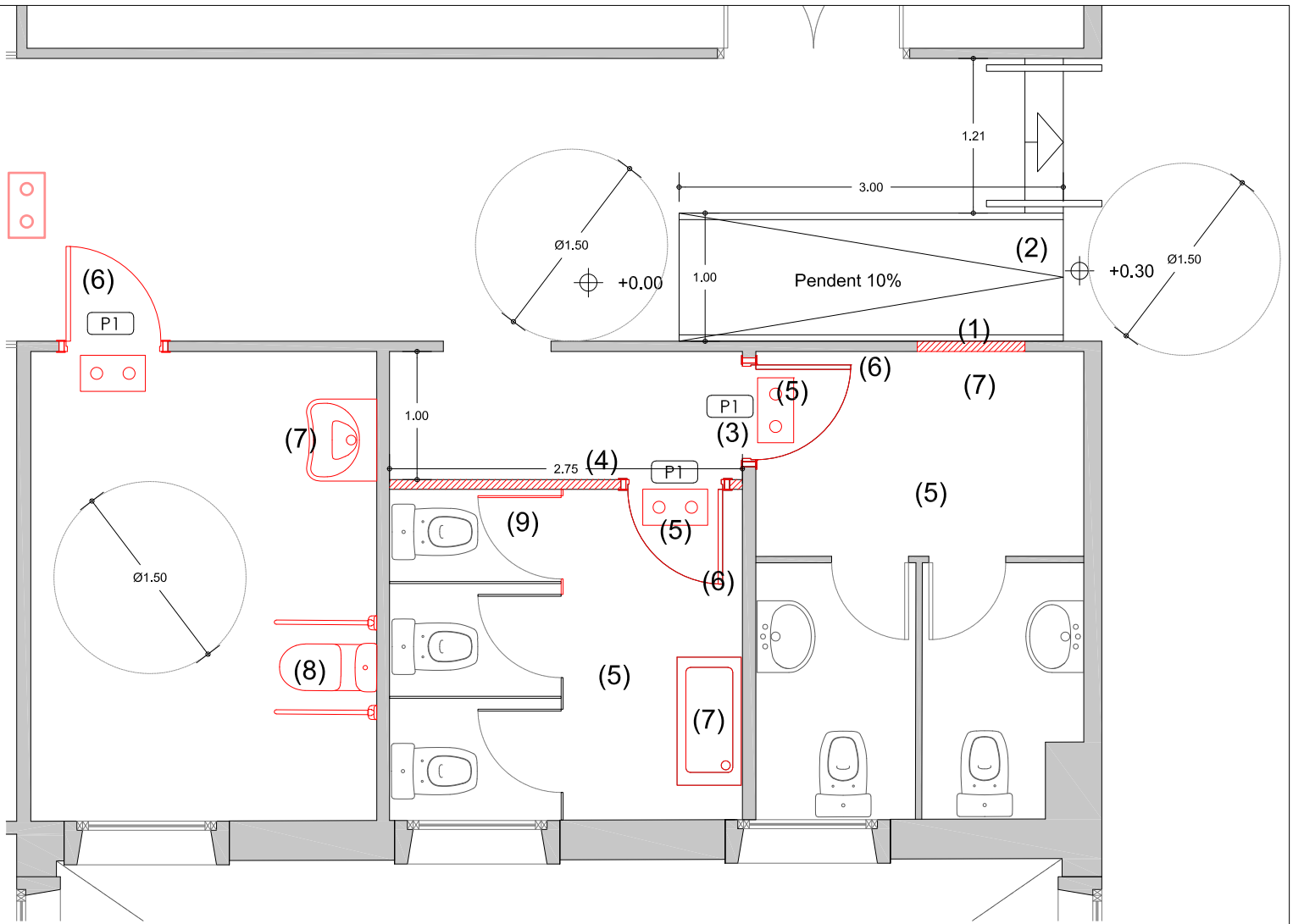
PLANTA PRIMERA - PROPOSTA
