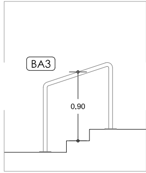
SECCIÓ C-C'
