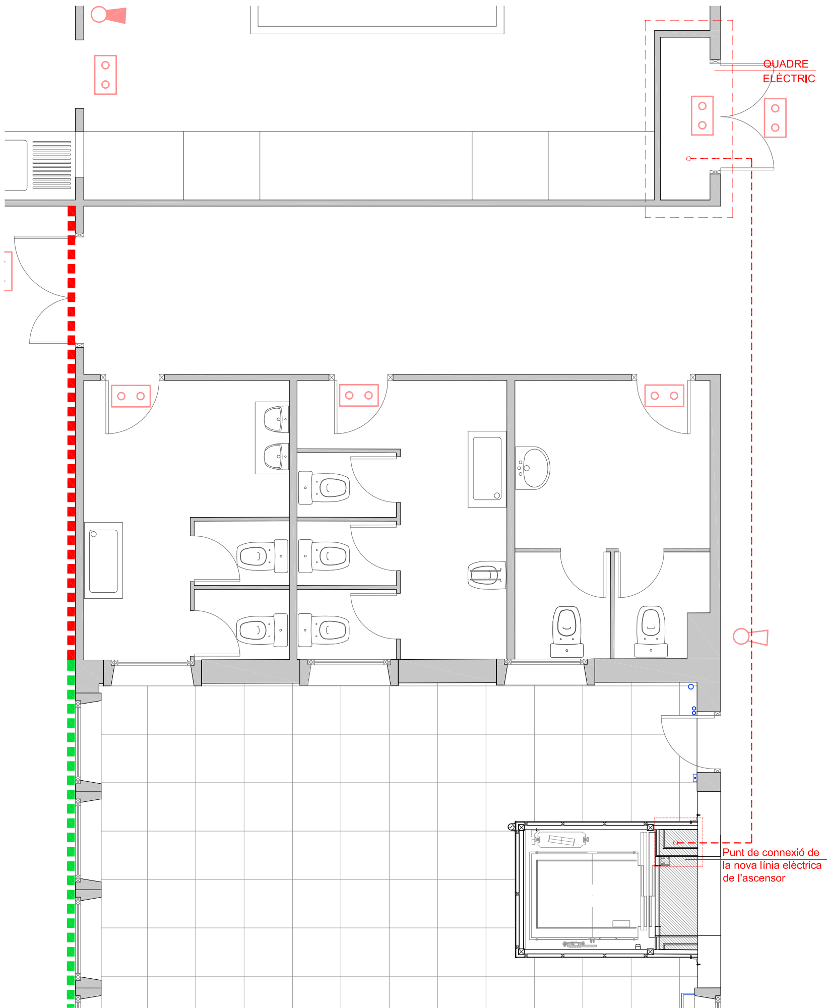
Planta Baixa - Connexió de l'ascensor amb el quadre elèctric general
