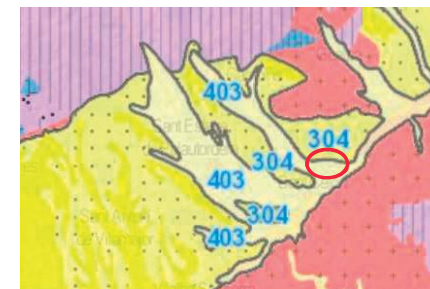
Mapa àrees hidrogeològiques publicat per l'IGCC.
