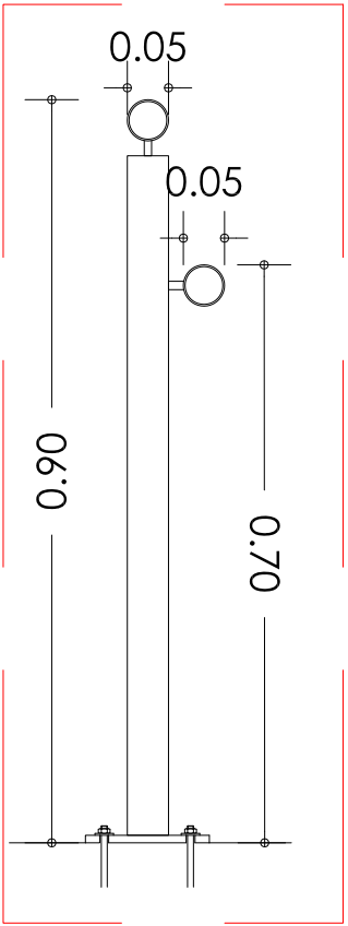
DETALL SECCIÓ 2 e.1/10
