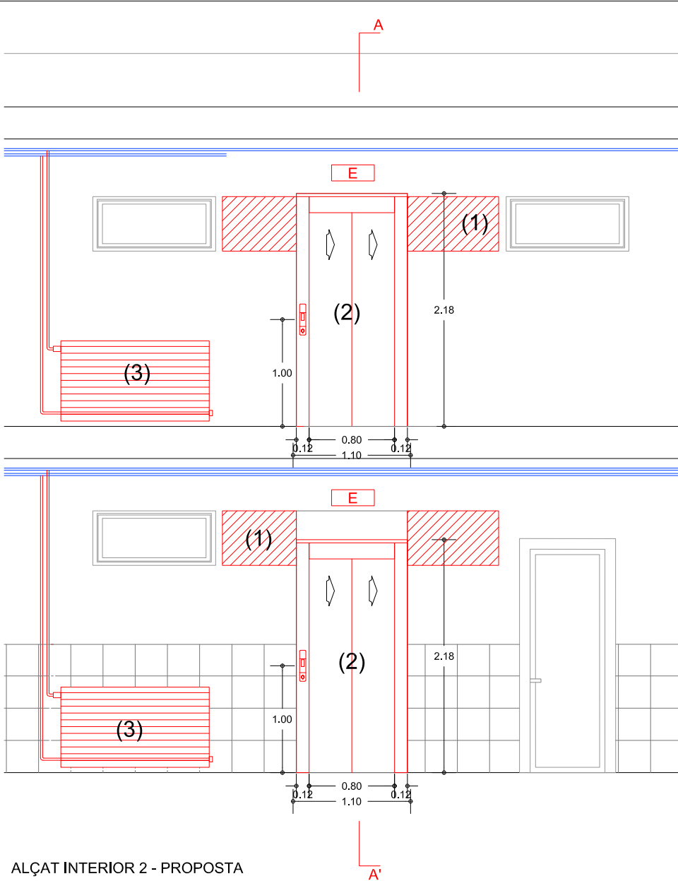
ALÇAT INTERIOR 2 - PROPOSTA
