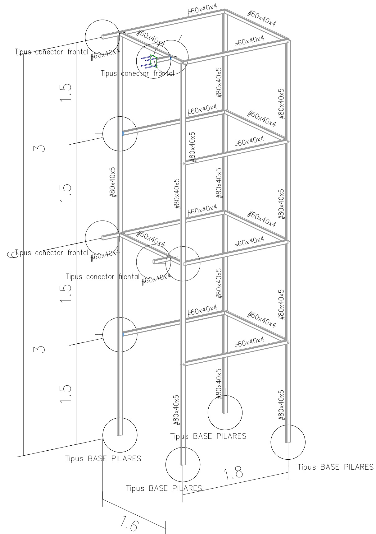
ESTRUCTURA CAIXA ASCENSOR - AXONOMÈTRIC
