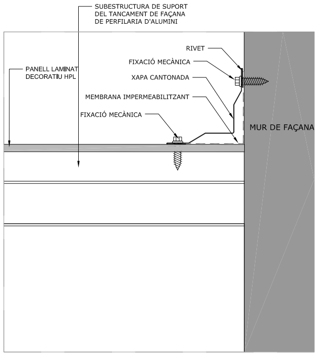
Detall 2: Racó exterior - Planta e.1/5
