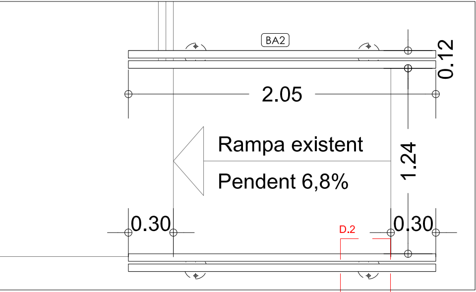
PLANTA RAMPA - ZONA D'ACTUACIÓ 3
