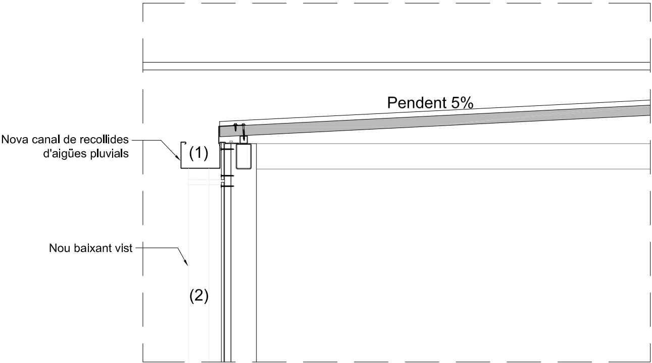
Detall: Secció Coberta de l'ascensor e 1/15
