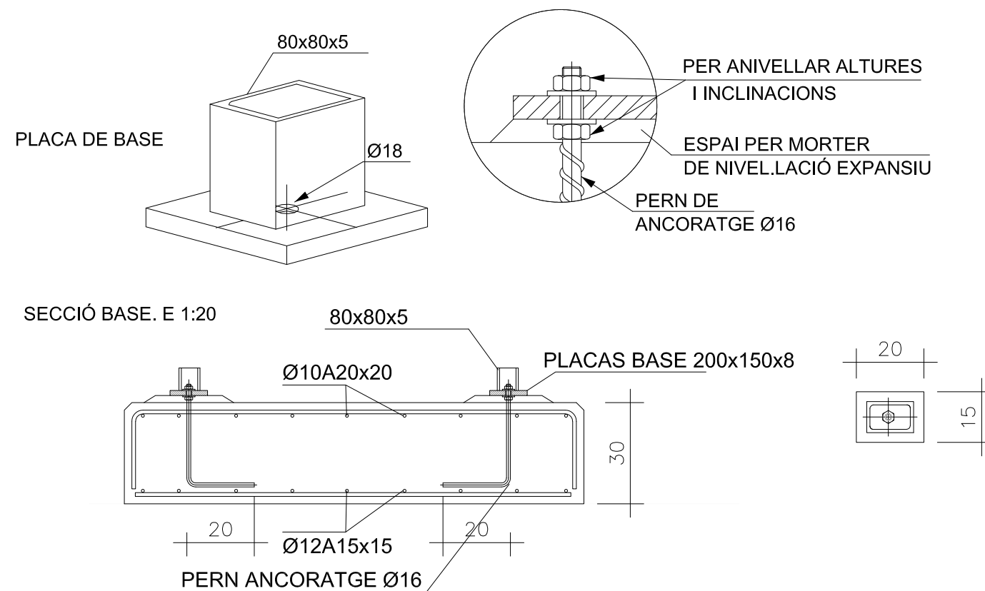
CIMENTACIÓ - DETALLS
