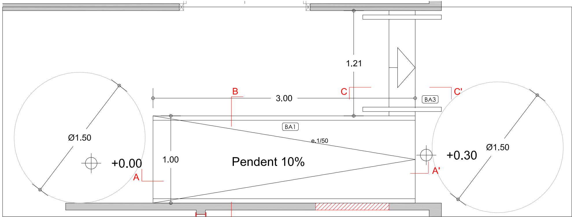
PLANTA RAMPA - ZONA D'ACTUACIÓ 2
