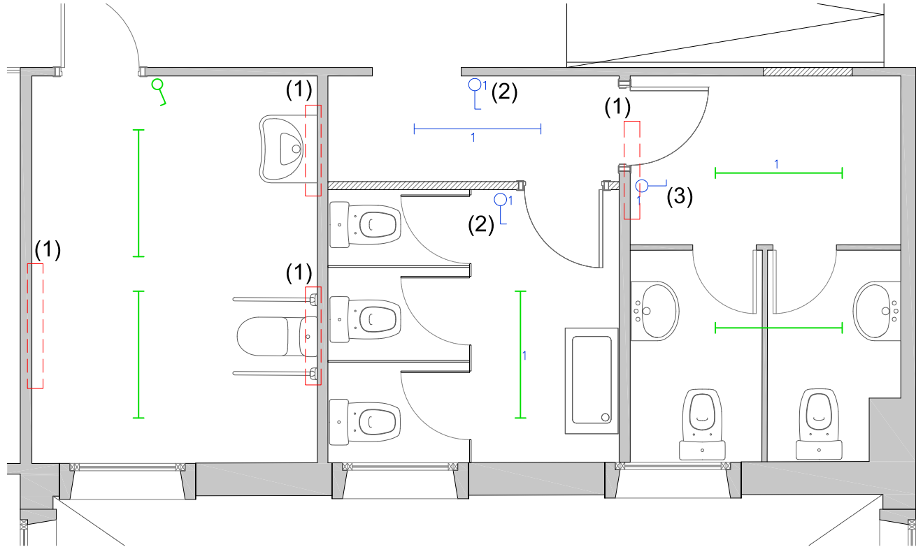
PLANTA PRIMERA - PROPOSTA
