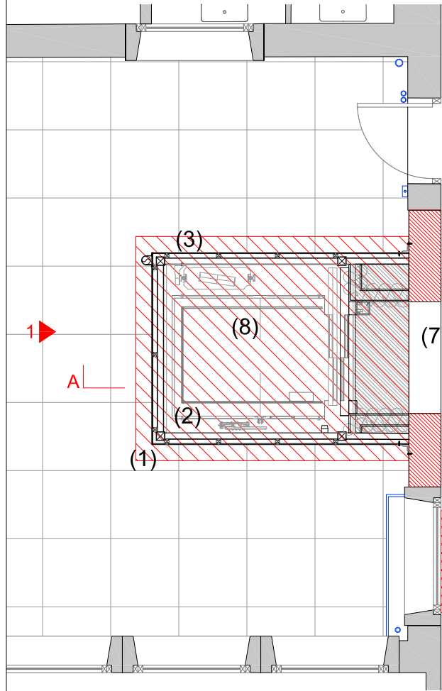
PLANTA BAIXA PROPOSTA
