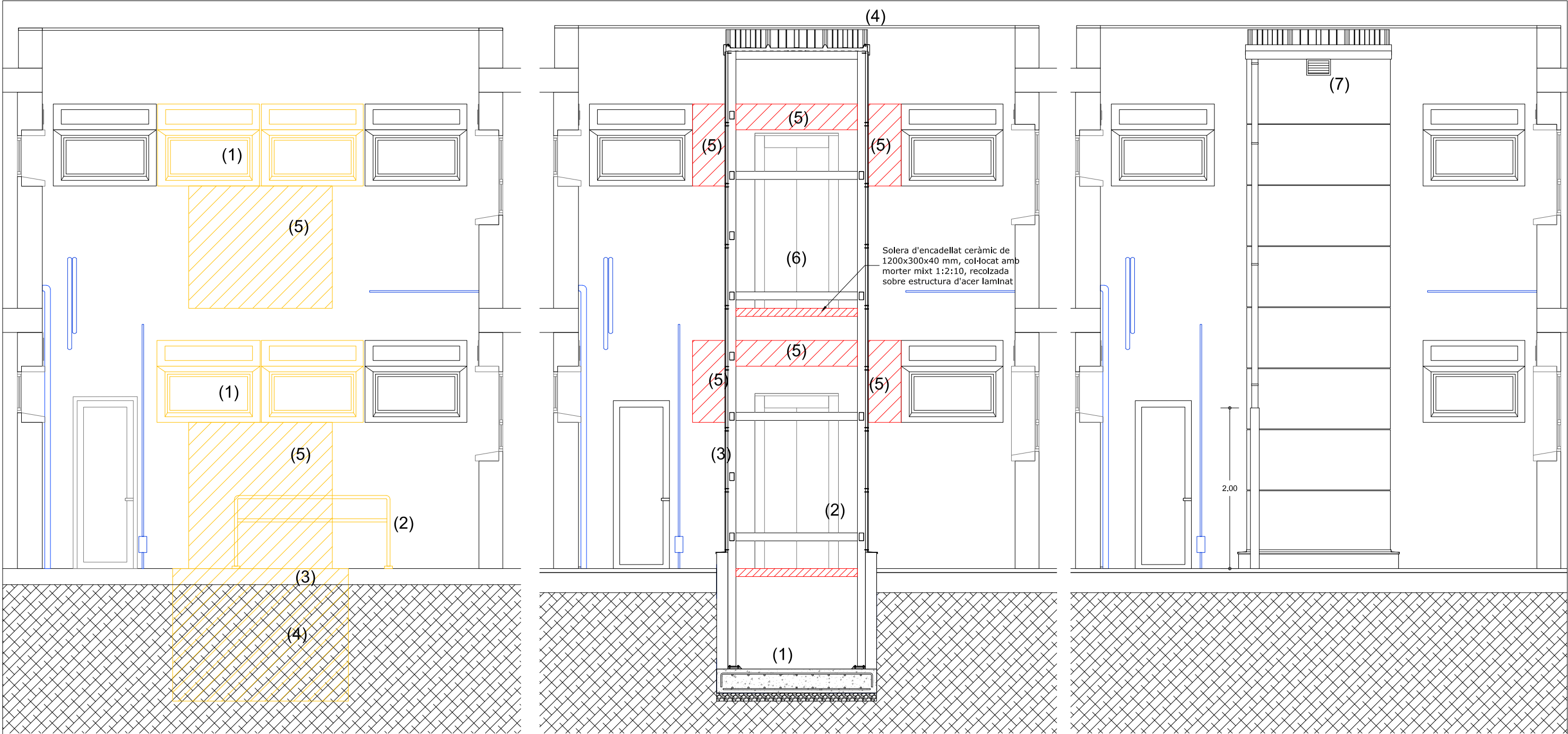
ALÇAT / SECCIÓ PATI - ESTAT ACTUAL
