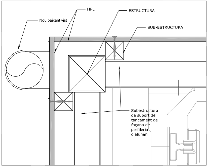
Detall 1: Cantonada exterior - Planta e.1/5
