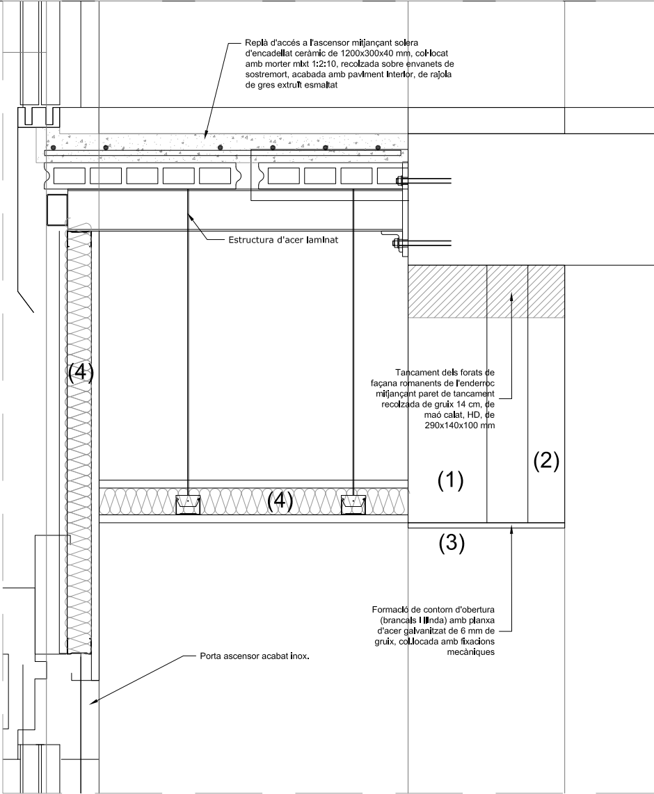
Detall 5: Replà d'accés en ascensor e.1/10
