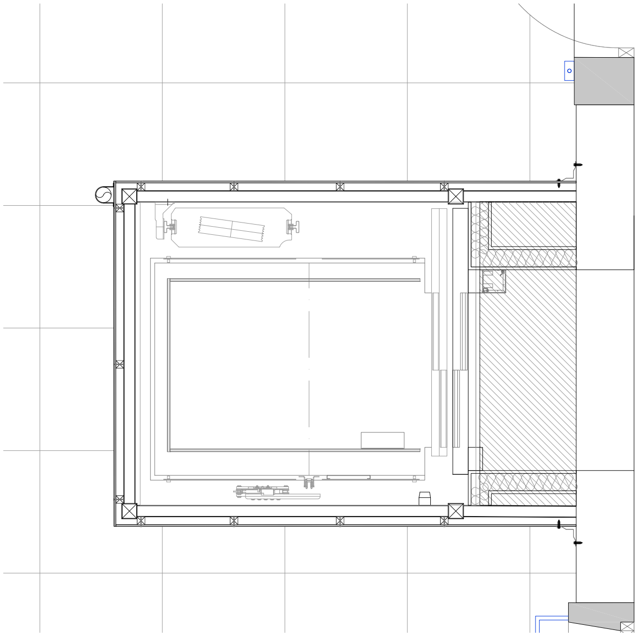
PLANTA BAIXA: ASCENSOR e 1/20
