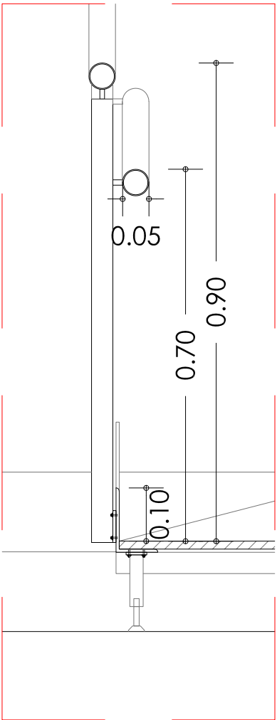
DETALL SECCIÓ 1 e.1/10
