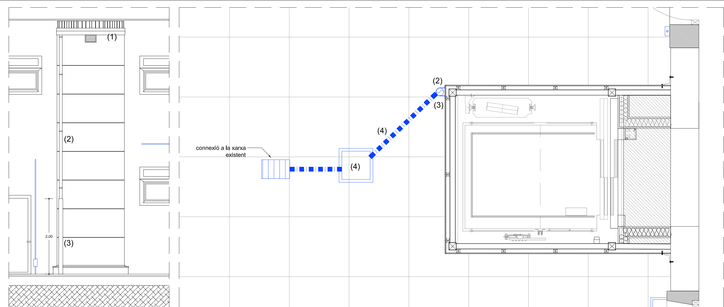
PLANTA BAIXA: ASCENSOR e 1/20
