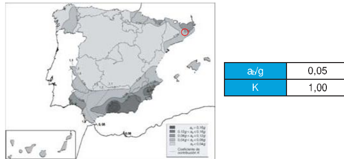
Figura 3: Mapa de risc sísmic d'Espanya
