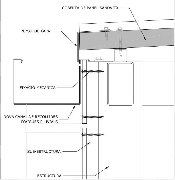
Detall 3: Trobada entre façana i la coberta de l'ascensor
