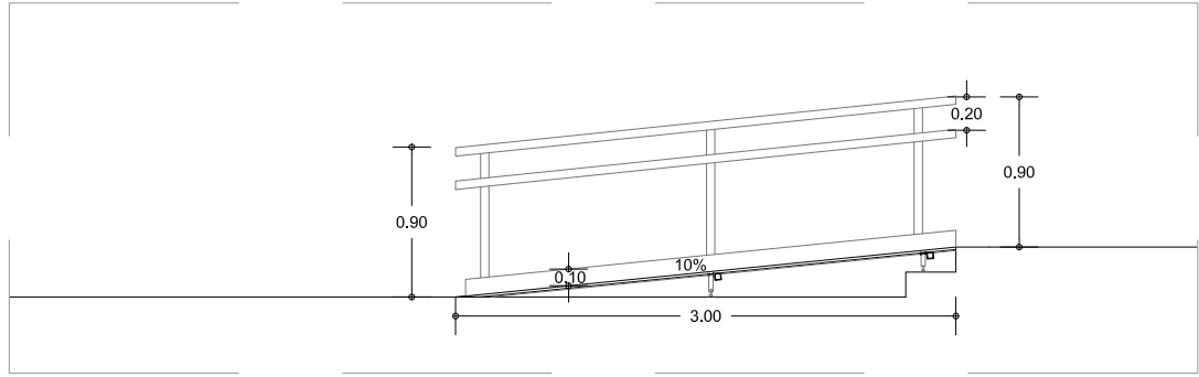
SECCIÓ RAMPA A-A'
