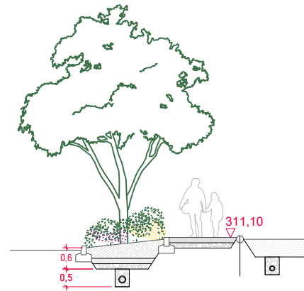
SECCIÓ 6 S6-S6'
