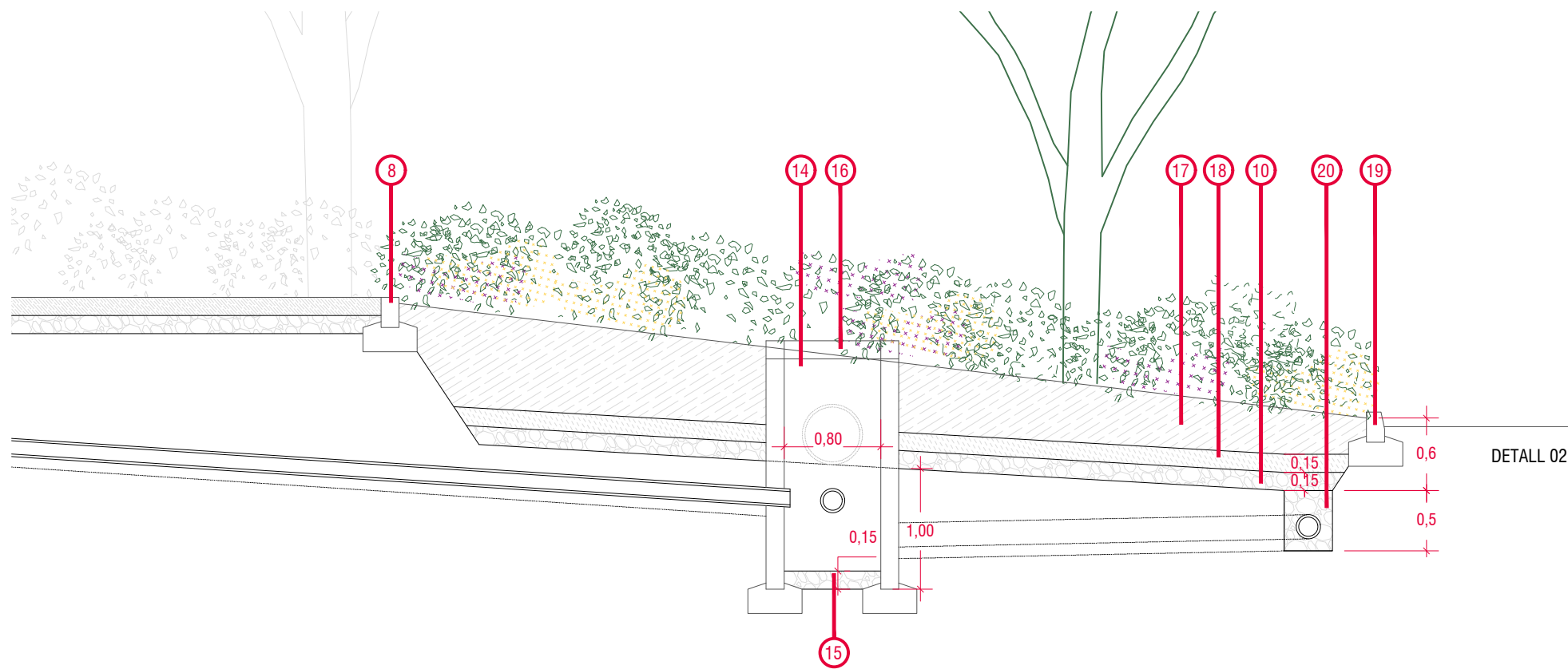
DETALL 01
