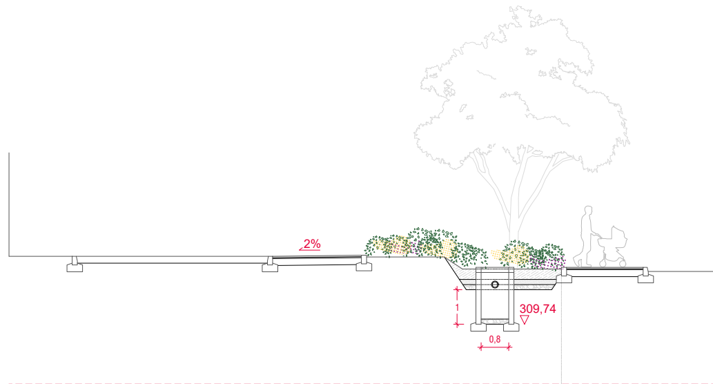
SECCIÓ 5 S5-S5'
