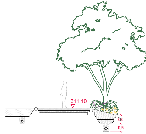
SECCIÓ 4 S4-S4'
