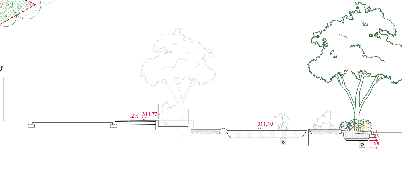
SECCIÓ 3 S3-S3'
