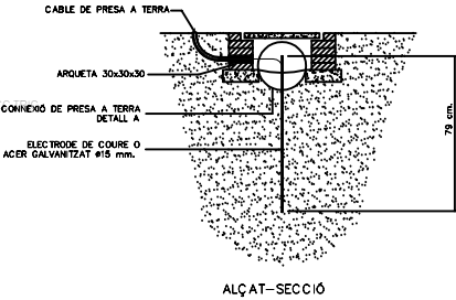
PRESA A TERRA NORMALITZADA GENERAL DE L' OBRA RESISTÈNCIA 80 OHMS, RESISTIVITAT 50 M. OHMS
