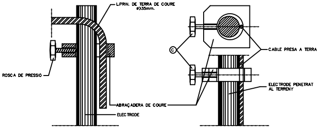
DETALL A
