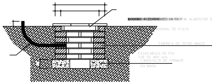
ALÇAT
