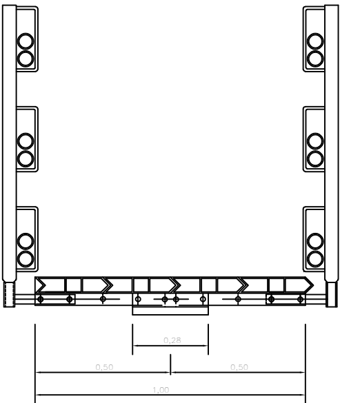
SECCIÓ ESCALA 1/10
