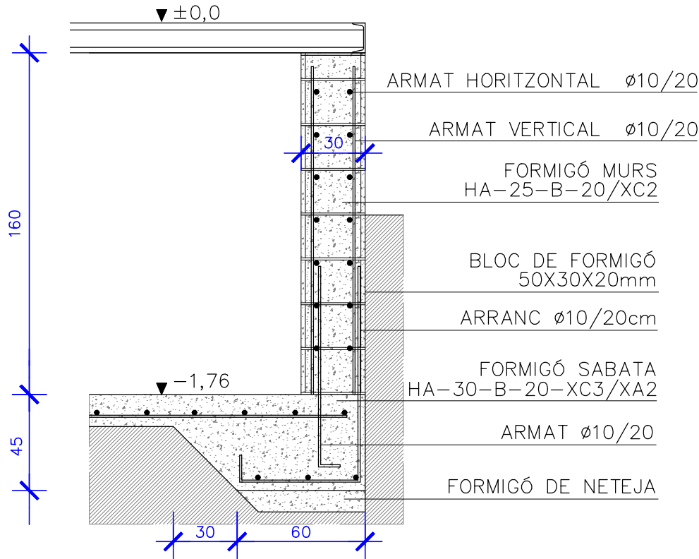
MB1. MUR BLOC DE FORMIGÓ – 30 cm
