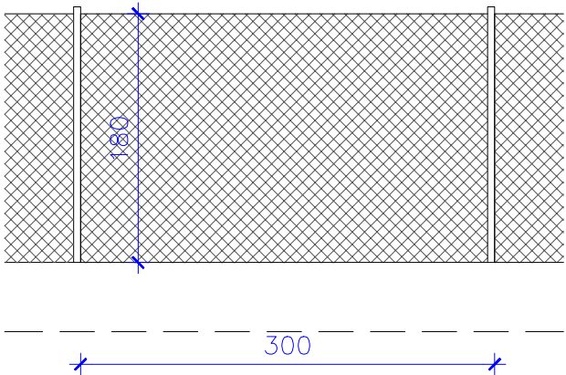
T1 62,33 ML REIXAT D'ACER AMB TELA METÀL·LICA DE TORSIÓ SIMPLE AMB ACABAT GALVANITZAT. PALS DE TUB GALVANITZAT Ø 50mm COL·LOCATS CADA 3m SOBRE MUR DE FORMIGÓ
