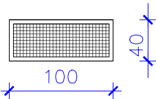
R3 4 UT REIXA AMB BASTIMENT PERIMETRAL PERFILS L 30.30mm ENTRAMAT METÀL·LIC TIPUS TRAMEX ACABAT GALVANITZAT
