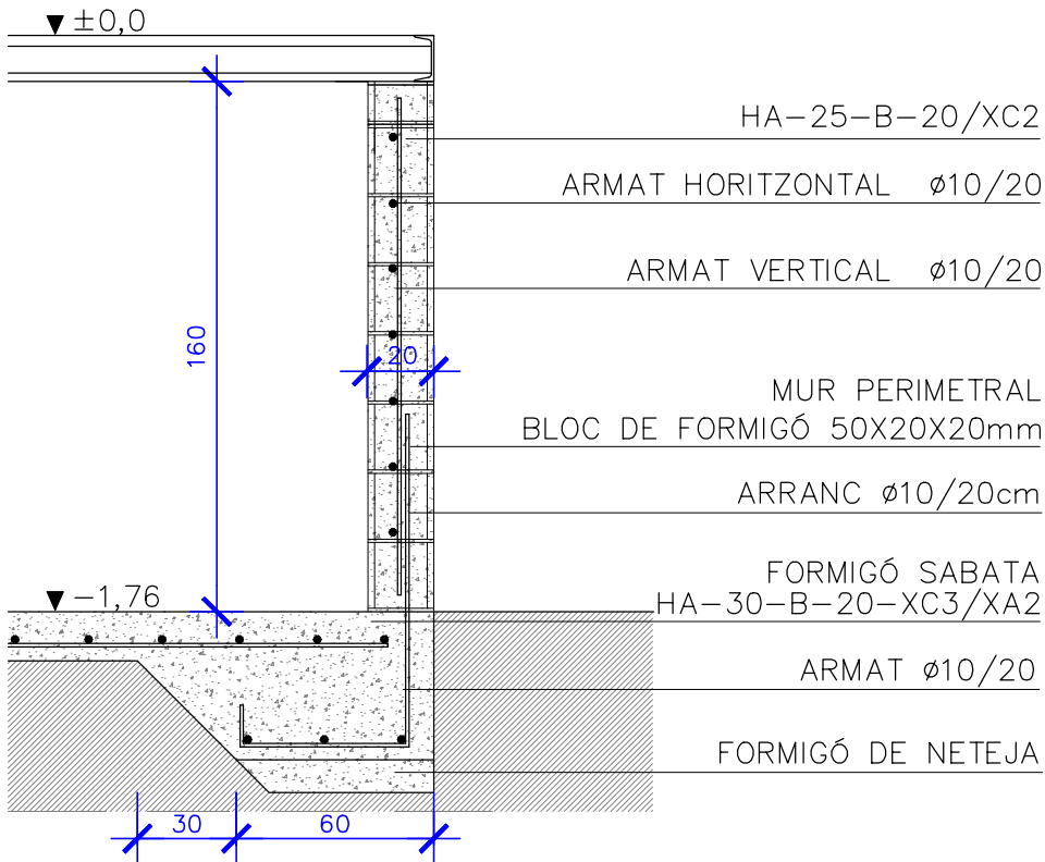
MB2. MUR BLOC DE FORMIGÓ – 20 cm
