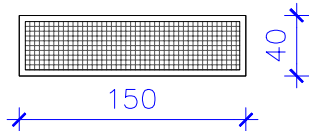
R2 3 UT REIXA AMB BASTIMENT PERIMETRAL PERFILS L 30.30mm ENTRAMAT METÀL·LIC TIPUS TRAMEX ACABAT GALVANITZAT
