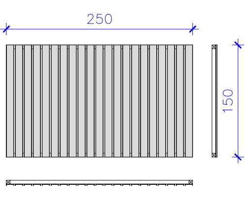
T2 1 UT TANCA FIXA SOBRE MURET DE BLOC DE FORMIGÓ ESTRUCTURA TUB ACER GALVANITZAT 50.50.2mm LAMES VERTICALS DE XAPA PLEGADA 3mm ACABAT GALVANITZAT FIXACIONS MECÀNIQUES
