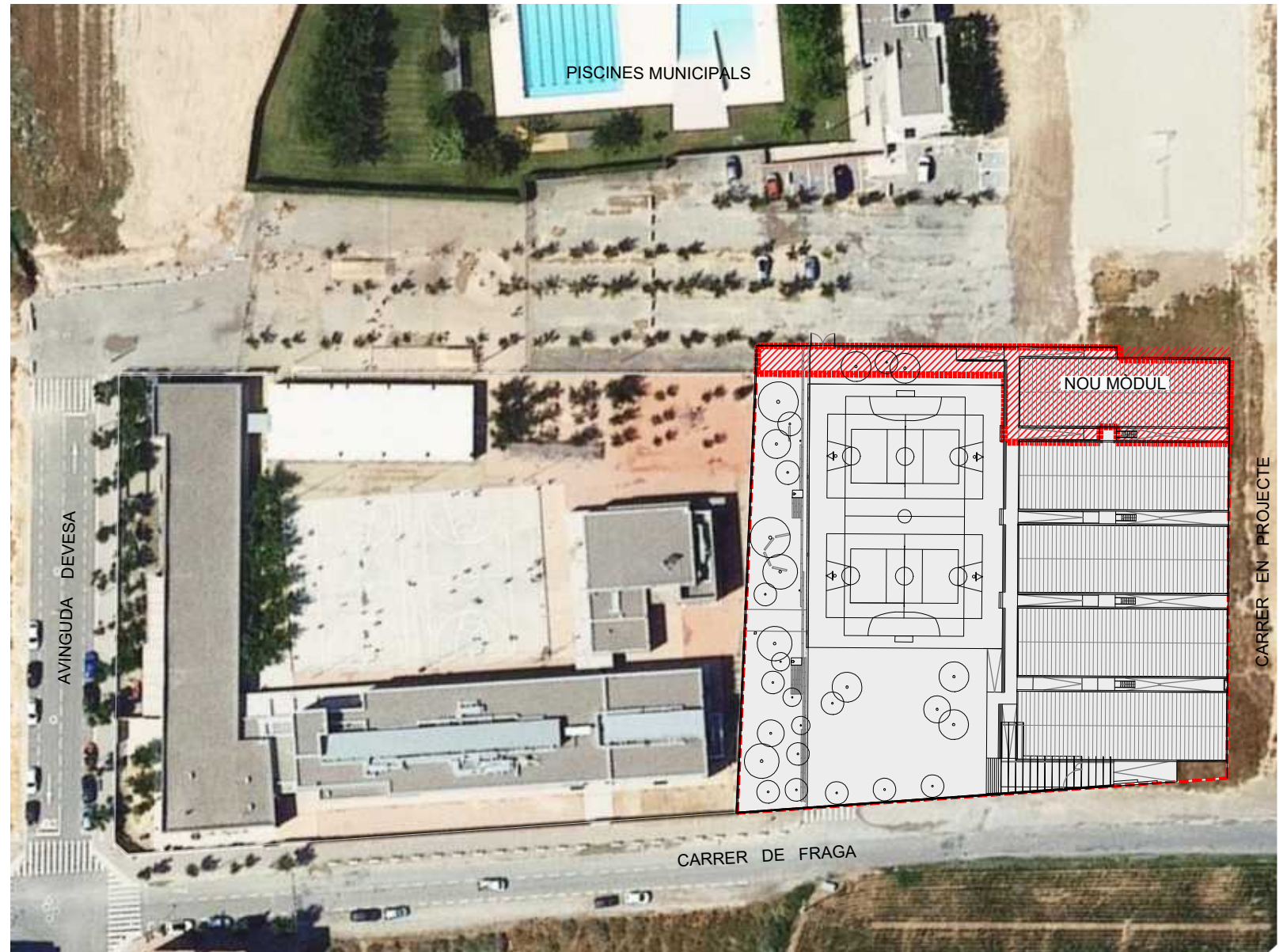
EMPLAÇAMENT 1/1000
