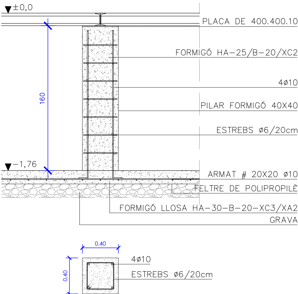
PILARS DE FORMIGÓ
