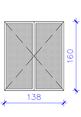
R1 1 UT PORTA DE PERFILS D'ACER LAMINAT PER A VENTILACIÓ BATENT DE 2 FULLES AMB PANY DE COP I CLAU PERFILS L 30.30mm ENTRAMAT METÀL·LIC TIPUS TRAMEX ACABAT GALVANITZAT
