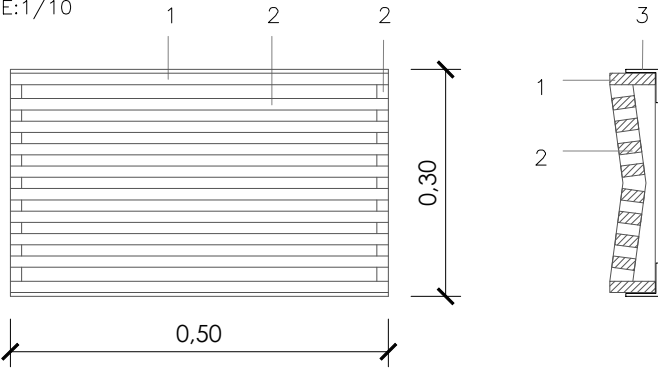
1 PASSAMA D'ACER GALVANITZAT DE 60X15 MM 2 PASSAMA D'ACER GALVANITZAT DE 30X15 MM 3 LPN 40.4 MM
