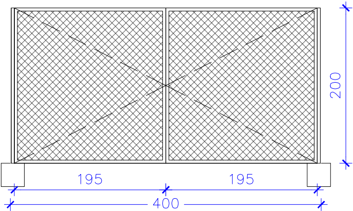
P1 1 UT PORTES BATENTS DE MARC D'ACER GALVANITZAT REIXAT D'ACER AMB TELA METÀL·LICA DE TORSIÓ SIMPLE ANCORATGE A PALS DE TUB GALVANITZAT Ø 50mm COL·LOCATS SOBRE DAUS DE FORMIGÓ
