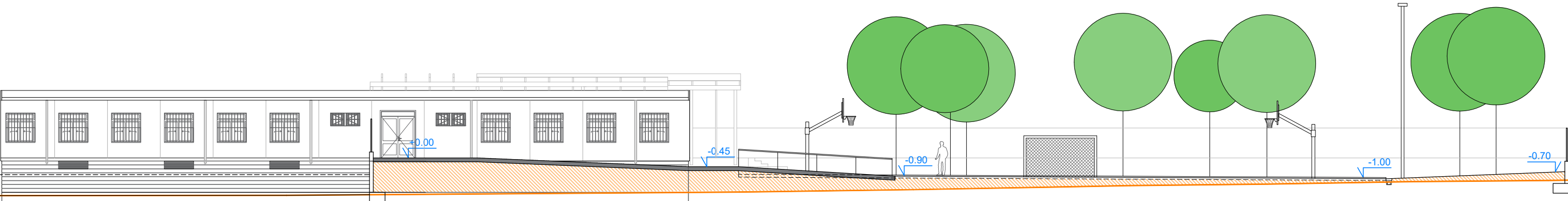
SECCIÓ 7-7
