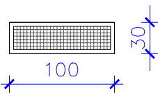
R4 4 UT REIXA AMB BASTIMENT PERIMETRAL PERFILS L 30.30mm ENTRAMAT METÀL·LIC TIPUS TRAMEX ACABAT GALVANITZAT
