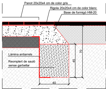
DETALL 2: FRANJA ANTIARRELS - NOVA CAIXA
