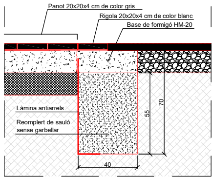
DETALL 1: FRANJA ANTIARRELS - CAIXA EXISTENT
