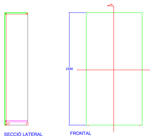
SECCIÓ LATERAL
