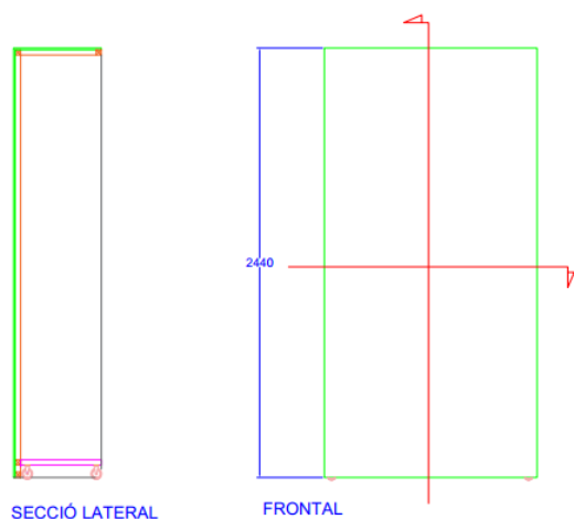
SECCIÓ LATERAL
