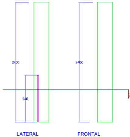
COLUMNA C2/C8
