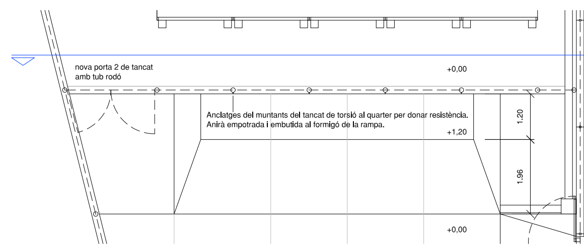
ALÇAT 2
