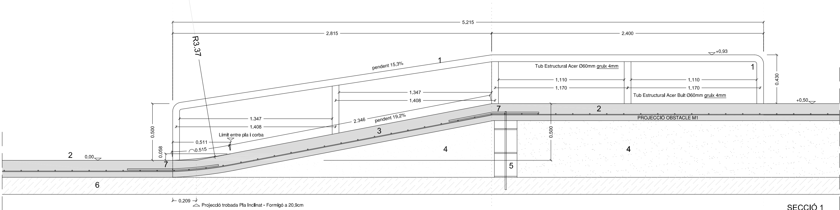
SECCIÓ 1
