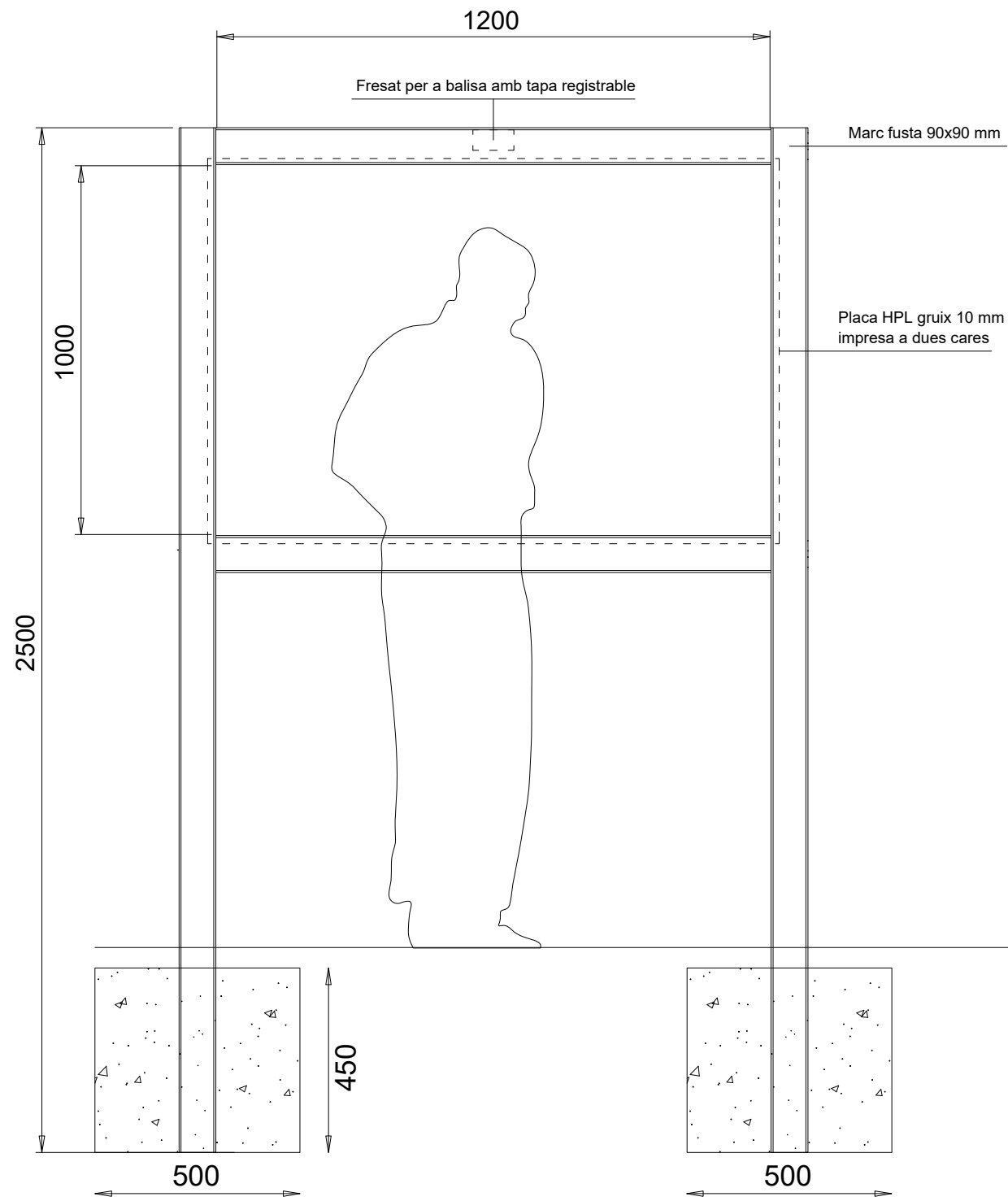
ALÇAT FRONTAL
