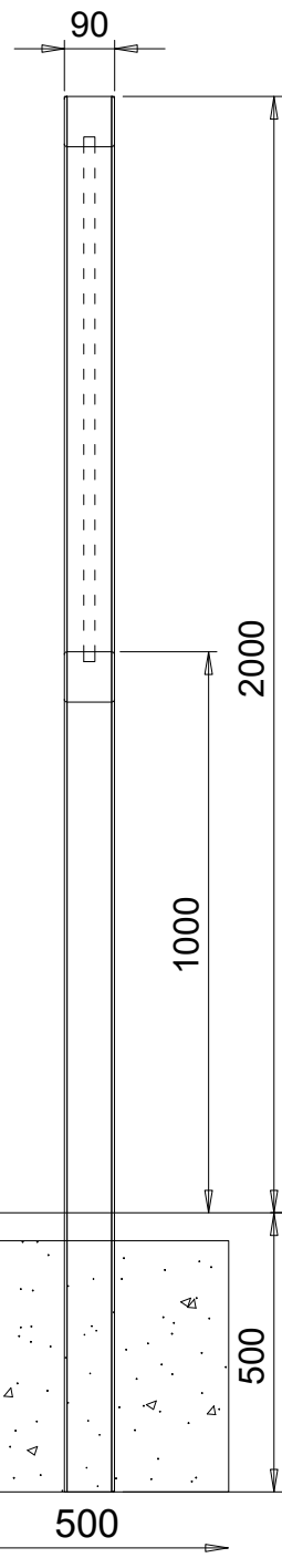
ALÇAT LATERAL
