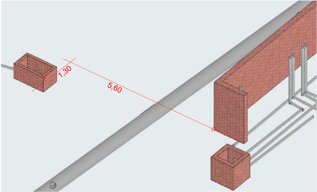
Ubicació Arqueta 3
