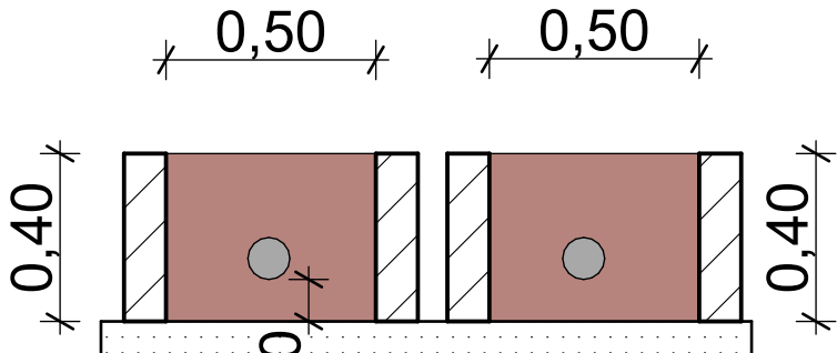
Secció C
