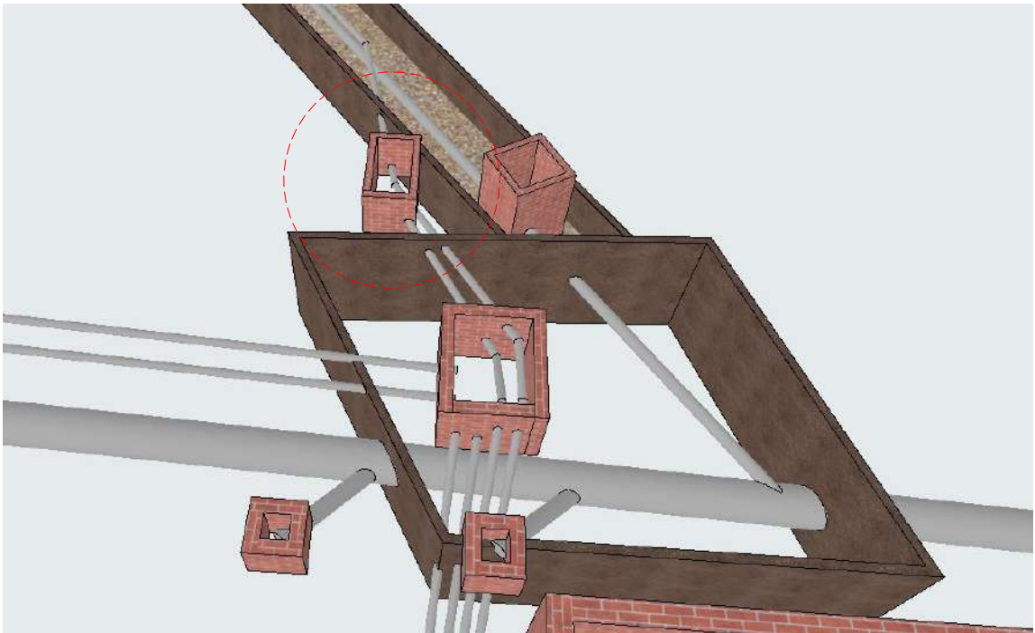
Vista Arqueta 3
