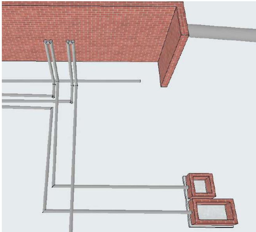
Vista arquetes 1 i 2 Aigua
