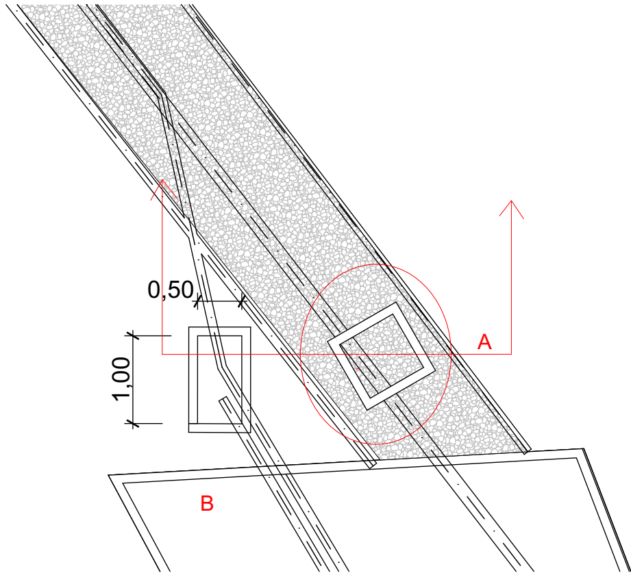
Planta cotes Arqueta 1 S.
