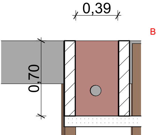
Secció arqueta
