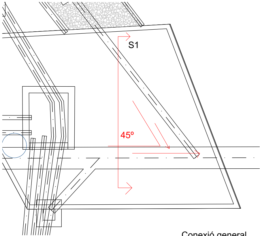
Conexió general
