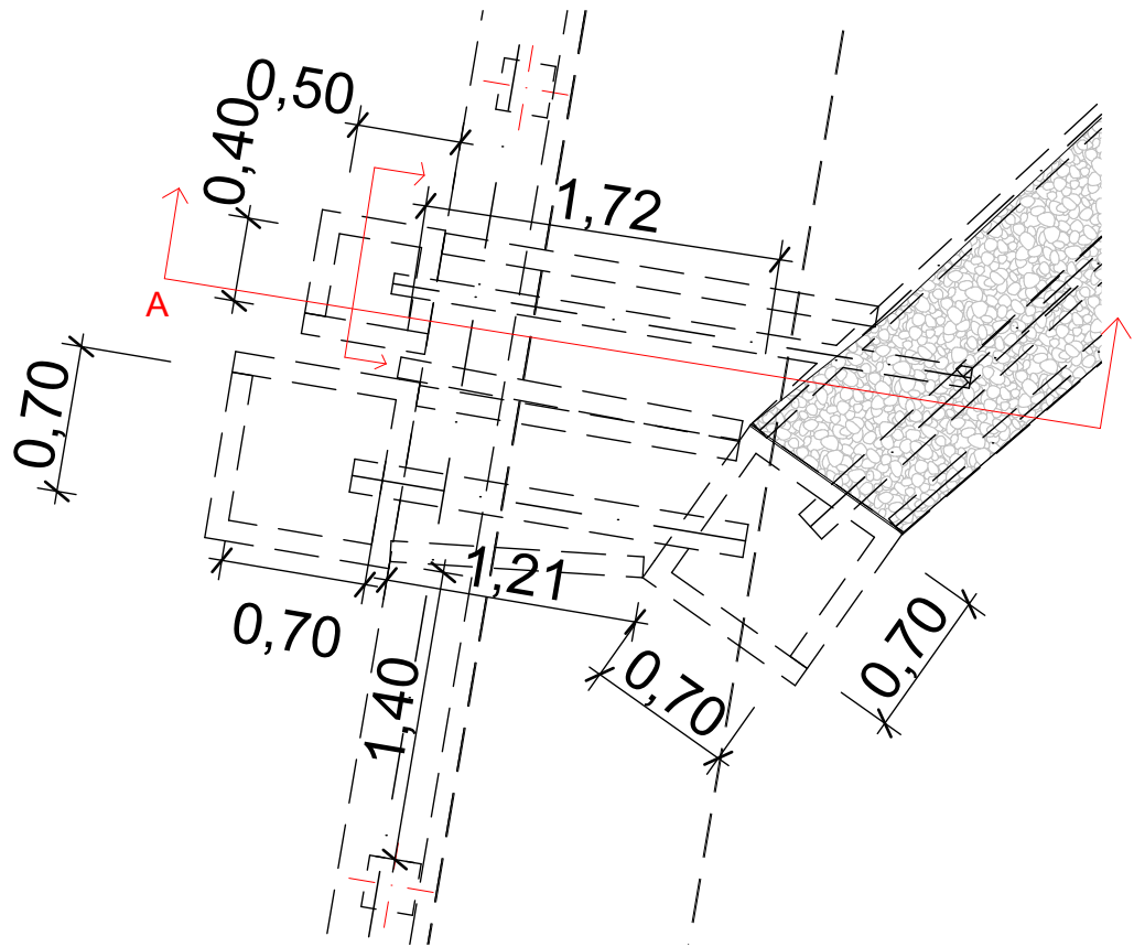
Planta cotes arquetes
