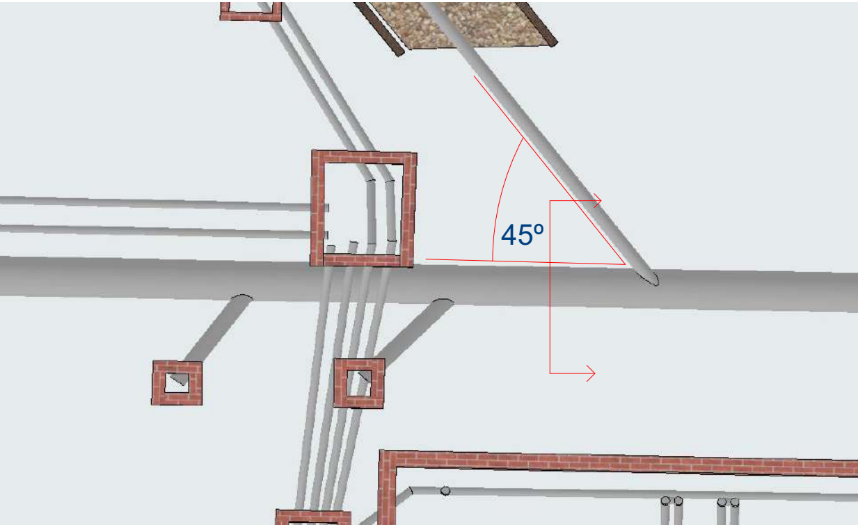
Angle Conexió
