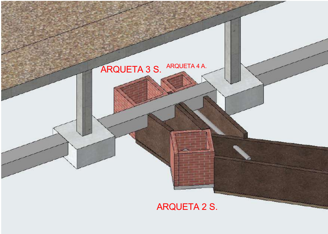
Vista arquetes 2 i 3 Sanejament i Arqueta 4 Agua
