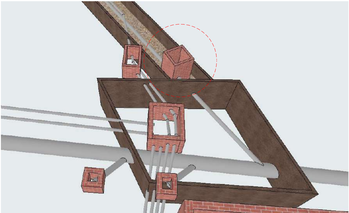
Vista Arqueta 1 S.
