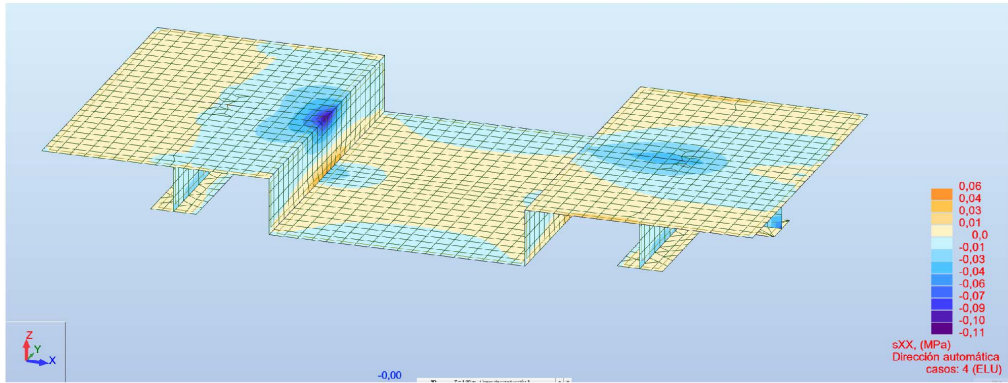
Sxx
