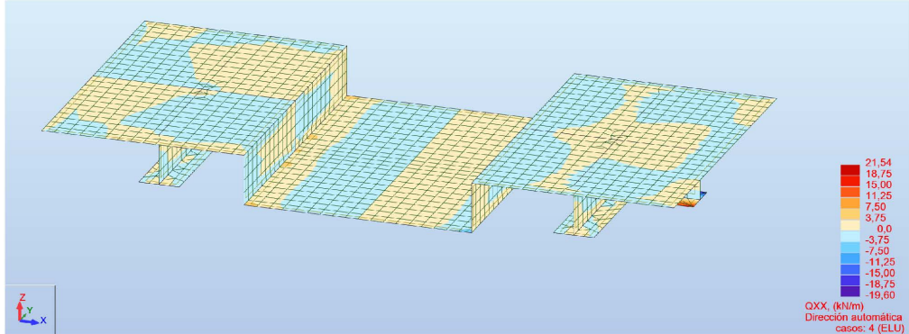
Cortante Qx
