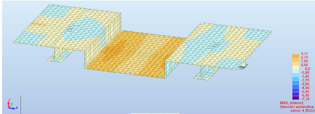
Momentos Mxx
