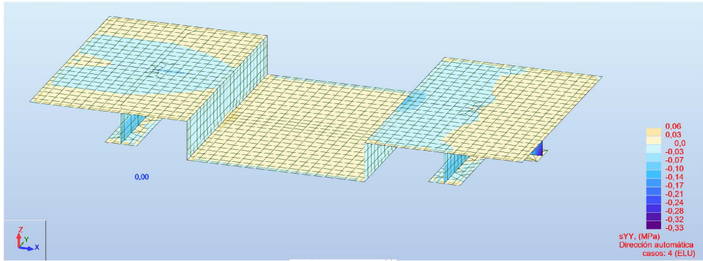
Syy
