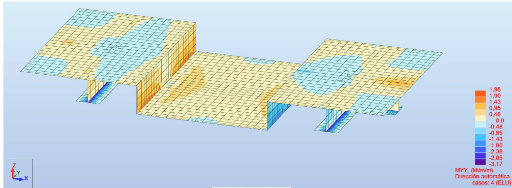
Momentos Myy
