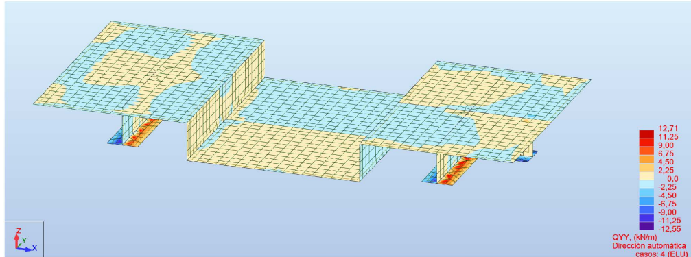
Cortante Qy
