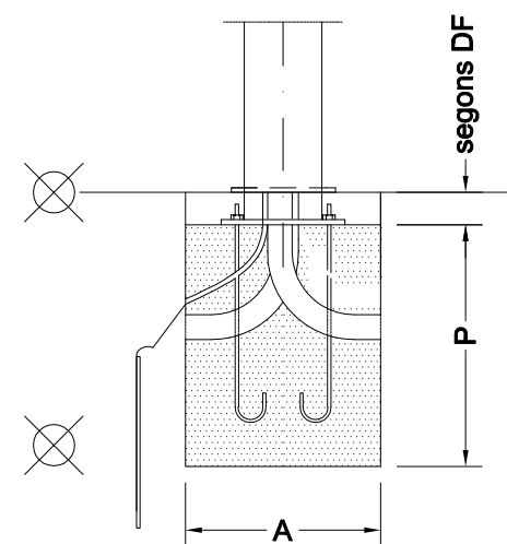
DETALL PAS DE CORRUGATS PEL DAU DE FORMIGÓ
