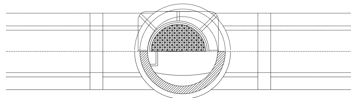
DETALL DEL POU DE PLUVIALS -PLANTA-
