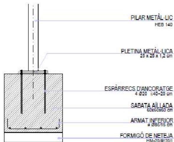
DETALL ANCLATGE DE COLUMNA D'ENLLUMENAT
