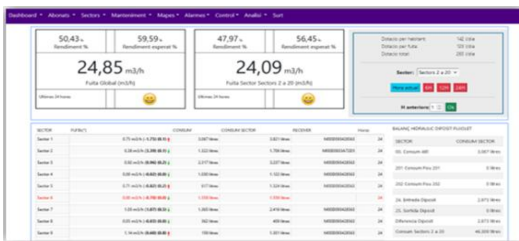
Pantalla de control del cabal mínim per sectors
