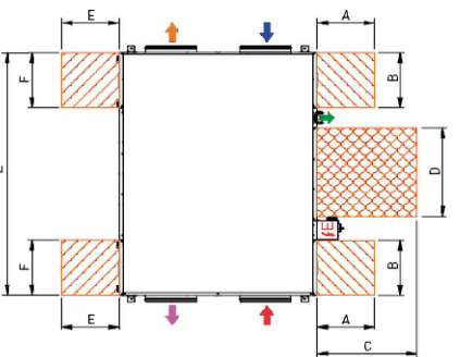
VISTA SUPERIOR POR DEFECTO DE DISEÑO DE FÁBRICA
