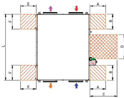
VISTA SUPERIOR CONFIGURACION RESULTADO DE SIMPLE MODIFICACION EN OBRA
