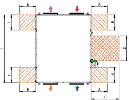
VISTA SUPERIOR CONFIGURACIÓN RESULTADO DE SIMPLE MODIFICACIÓN EN OBRA
