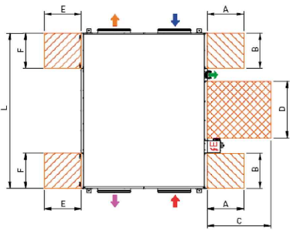
VISTA SUPERIOR POR DEFECTO (SUMINISTRO DE FABRICA)
