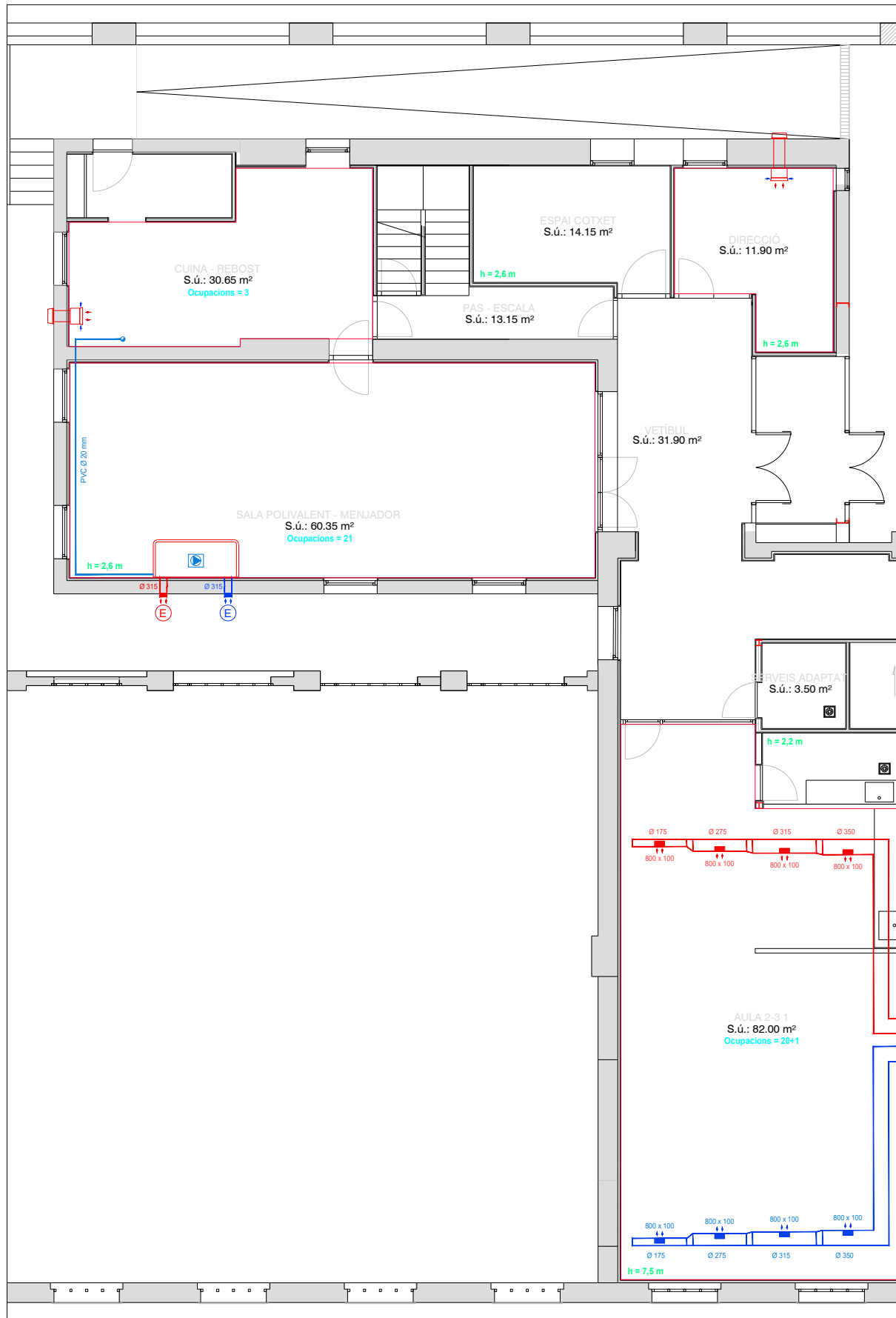
PLANTA BAIXA
