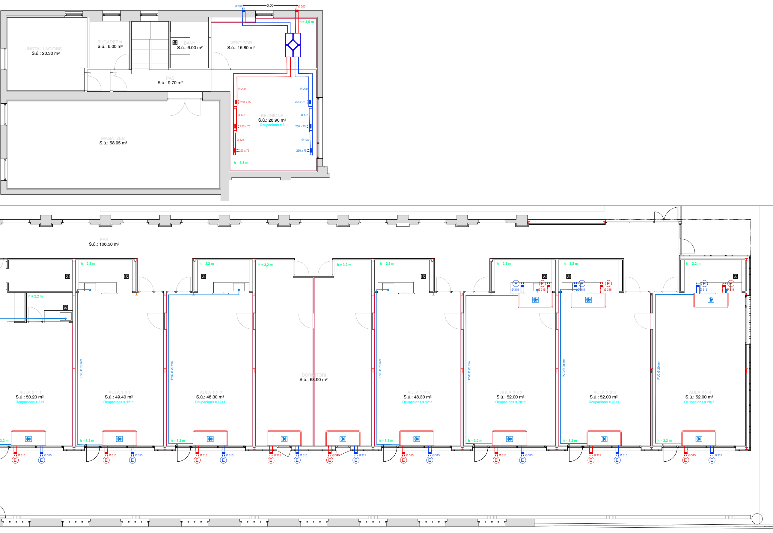
PLANTA PIS
