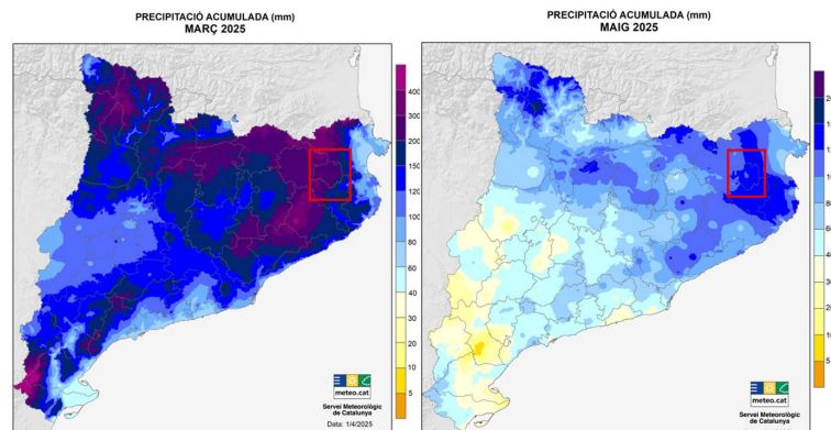
Mapes de precipitació del mes de març i de maig a la comara del Pla de l'Estant (Font: Meteocat)
