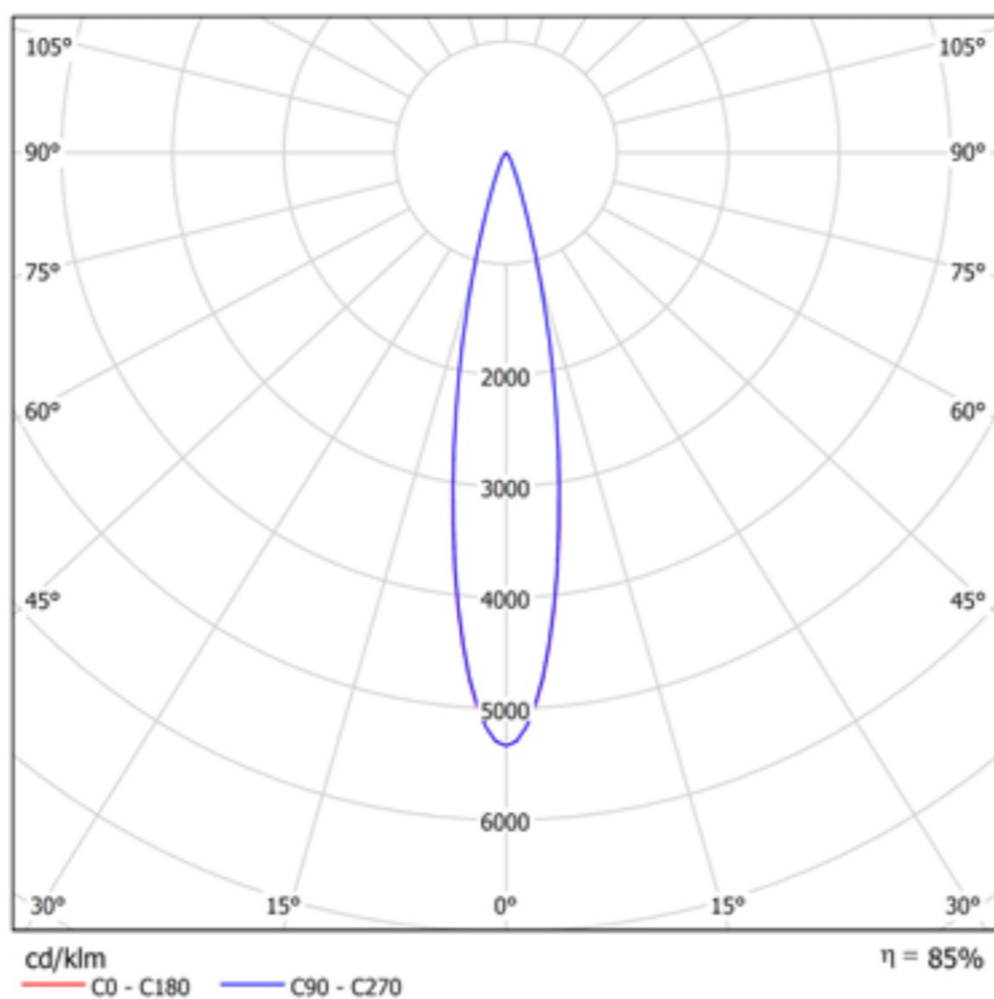
Diagrama polar
