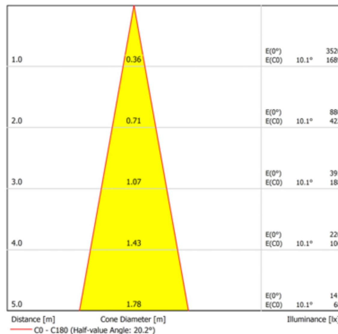
Diagrama cónico
