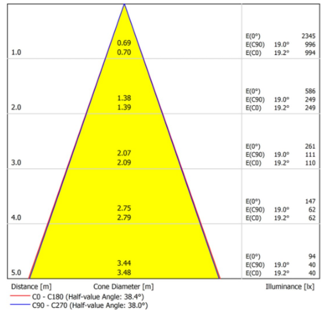
Diagrama cónico
