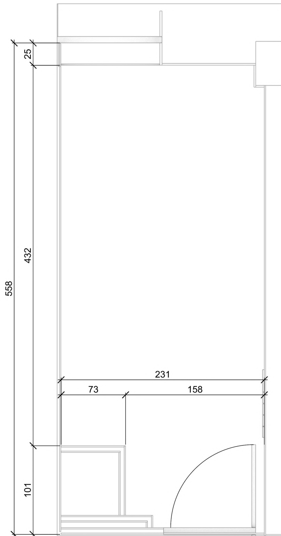
PLANTA 3
