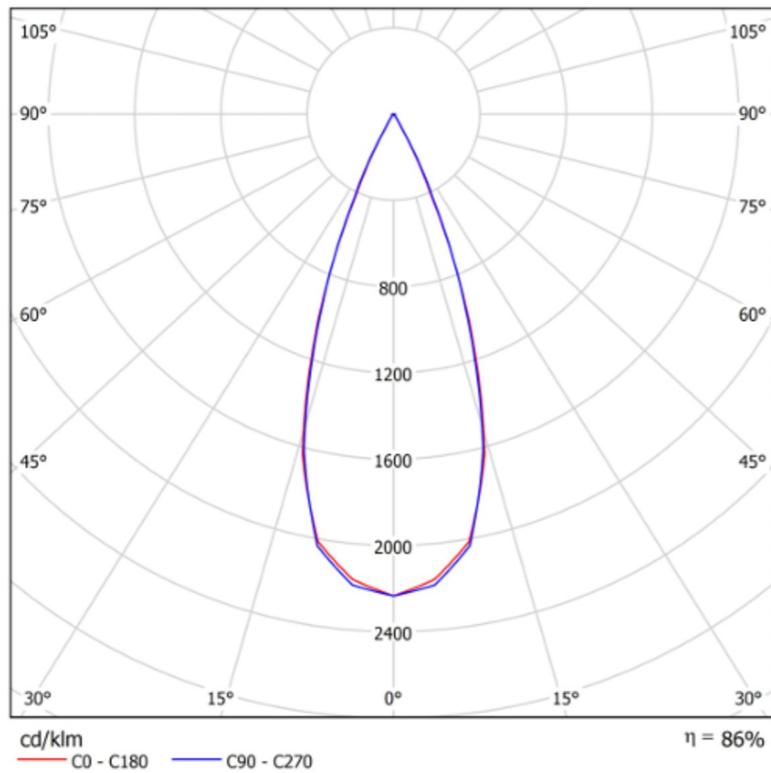
Diagrama polar
