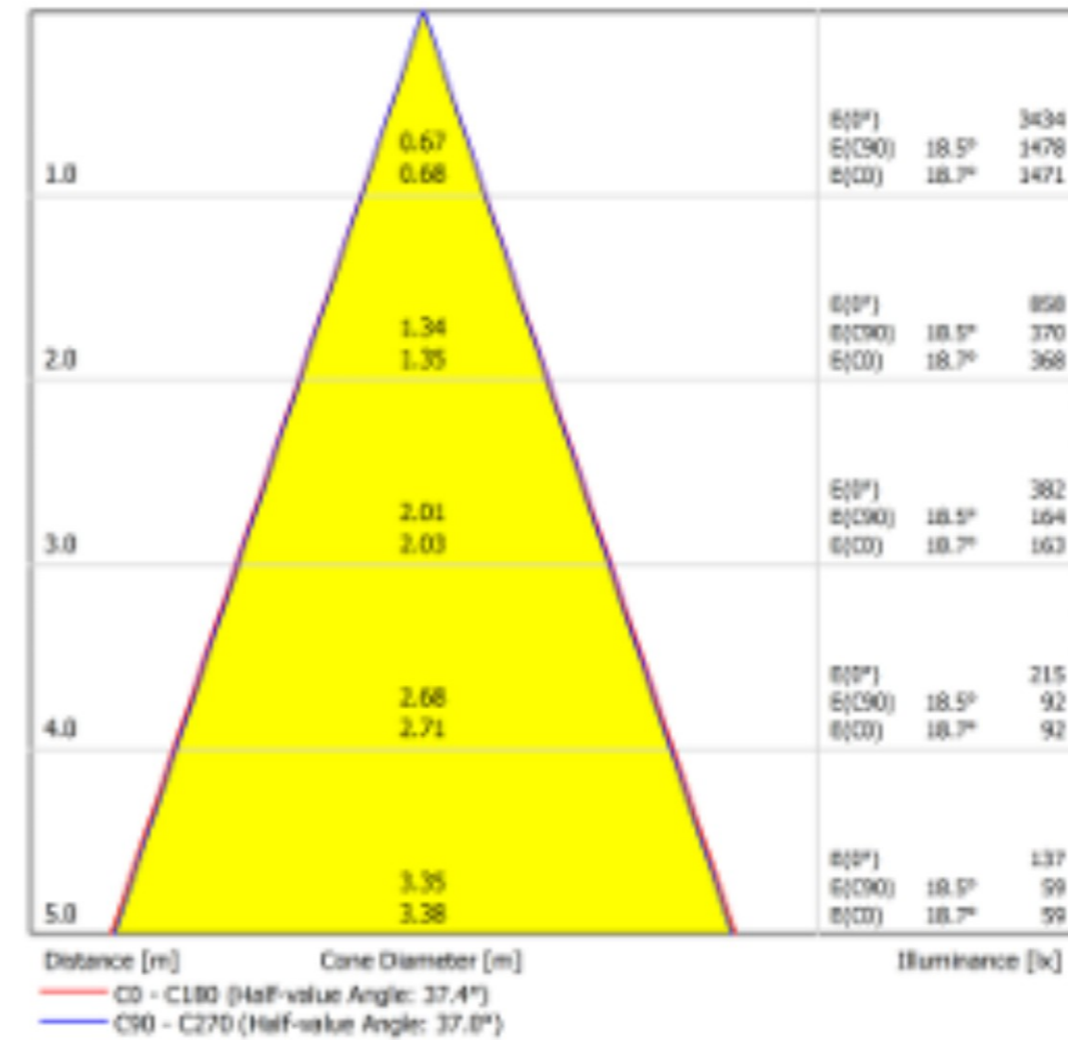
Diagrama cónico
