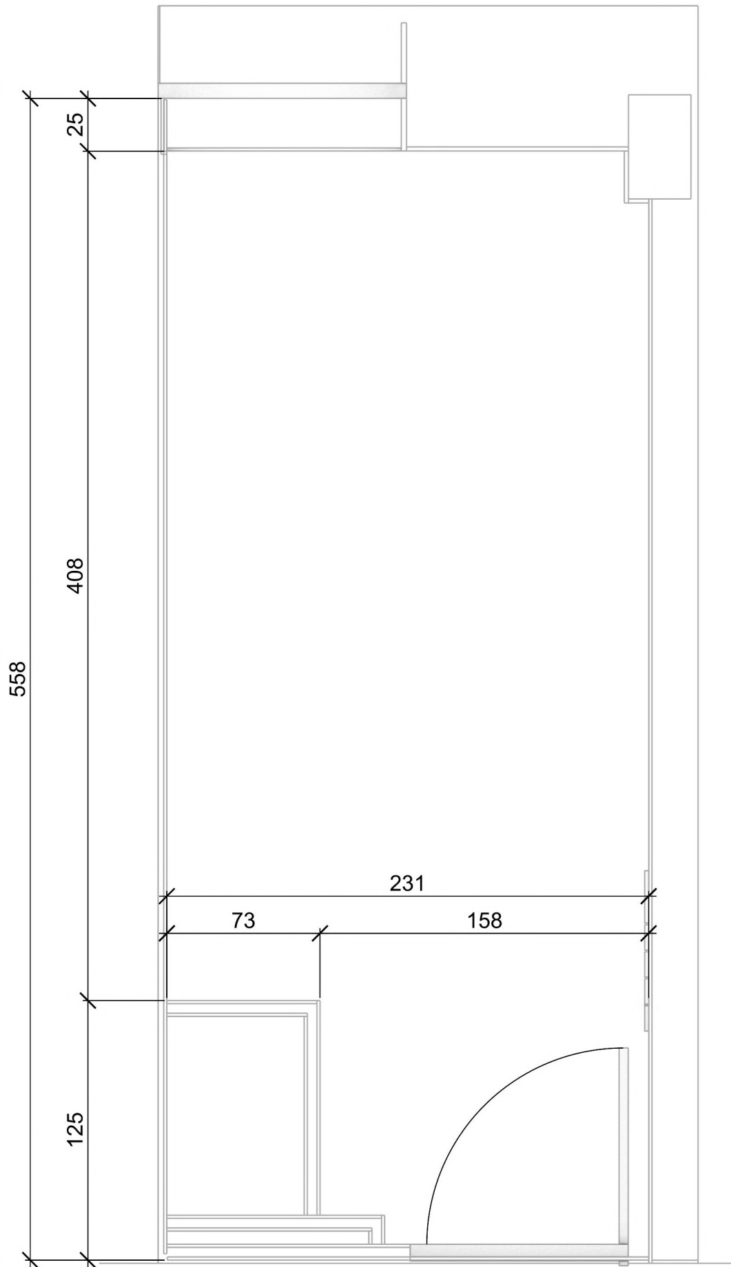
PLANTA 2
