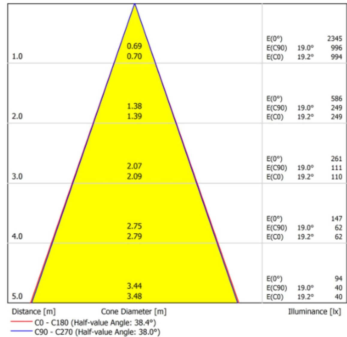
Diagrama cónico
