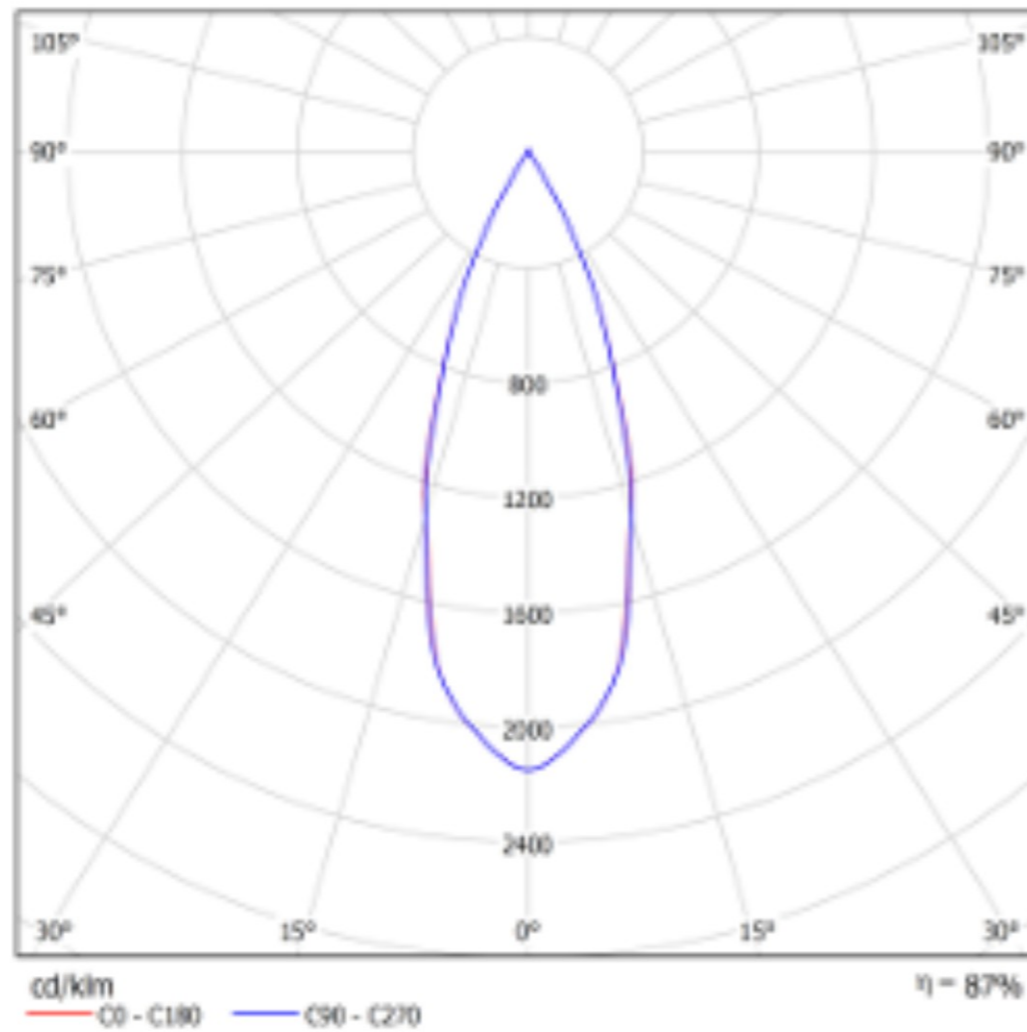
Diagrama polar
