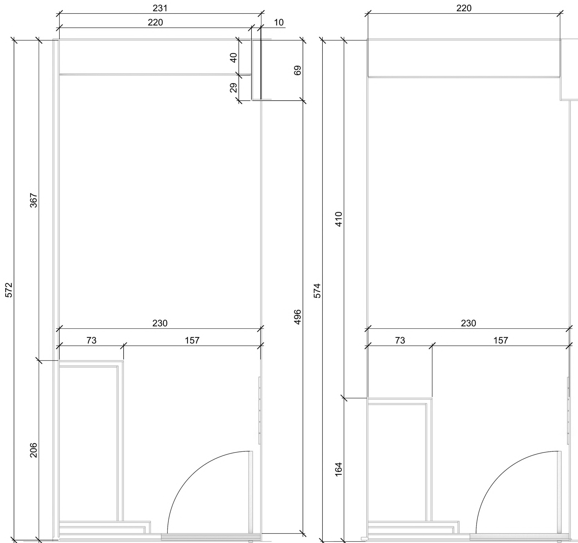
PLANTA 0
