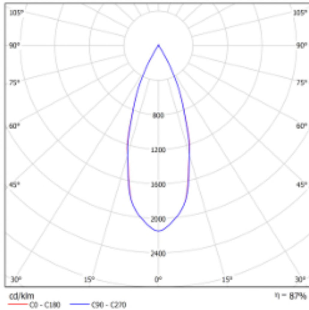
Diagrama polar
