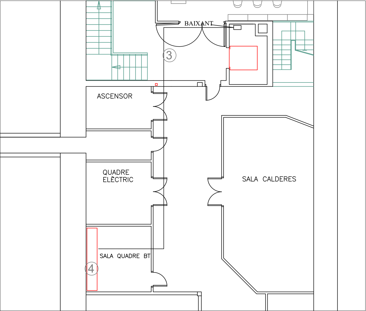
ESTAT ACTUAL PLANTA SOTERRANI. ESCALA 1:100
