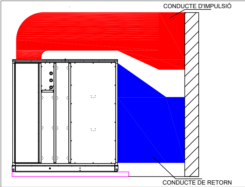
DETALL A-A': CONNEXIÓ CONDUCTE IMPULSIÓ I RETORN. ESCALA 1:50
