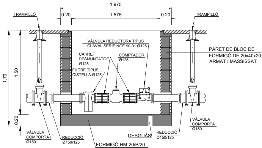
SECCIÓ A-A'
