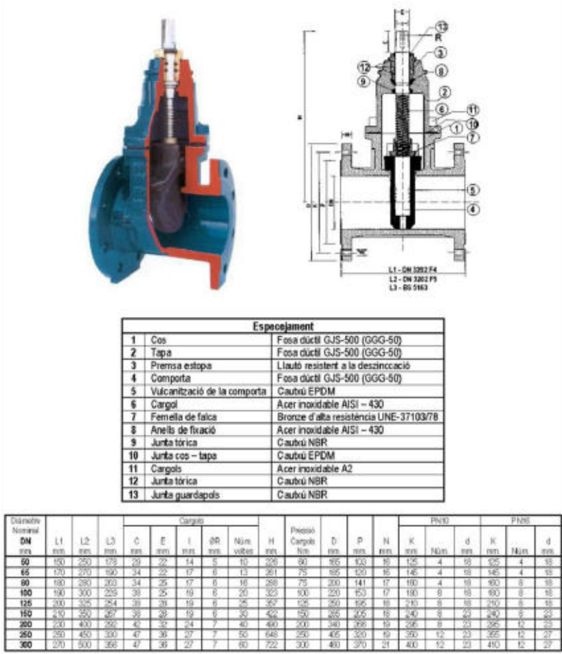
VÀLVULA COMPORTA AMB BRIDES
