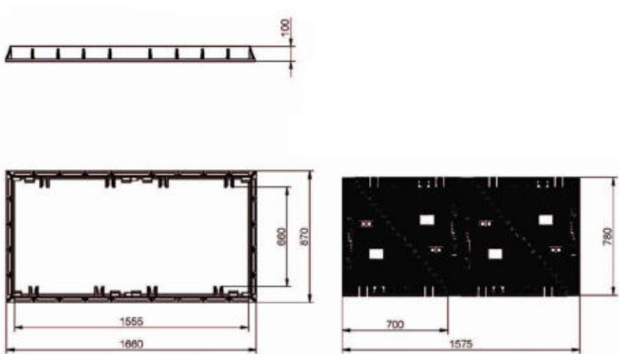
PLANTES I ALÇAT TAPA DE FOSA DÚCTIL
