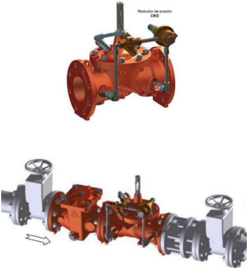
VÀLVULA REGULADORA DE PRESSIÓ
