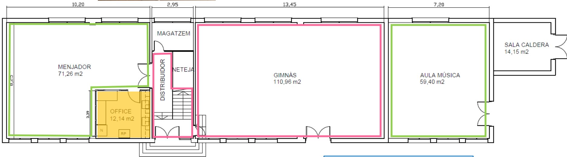
PLANTA BAIXA
