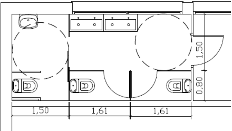
EDIFICI 2: Planta baixa i planta pis
