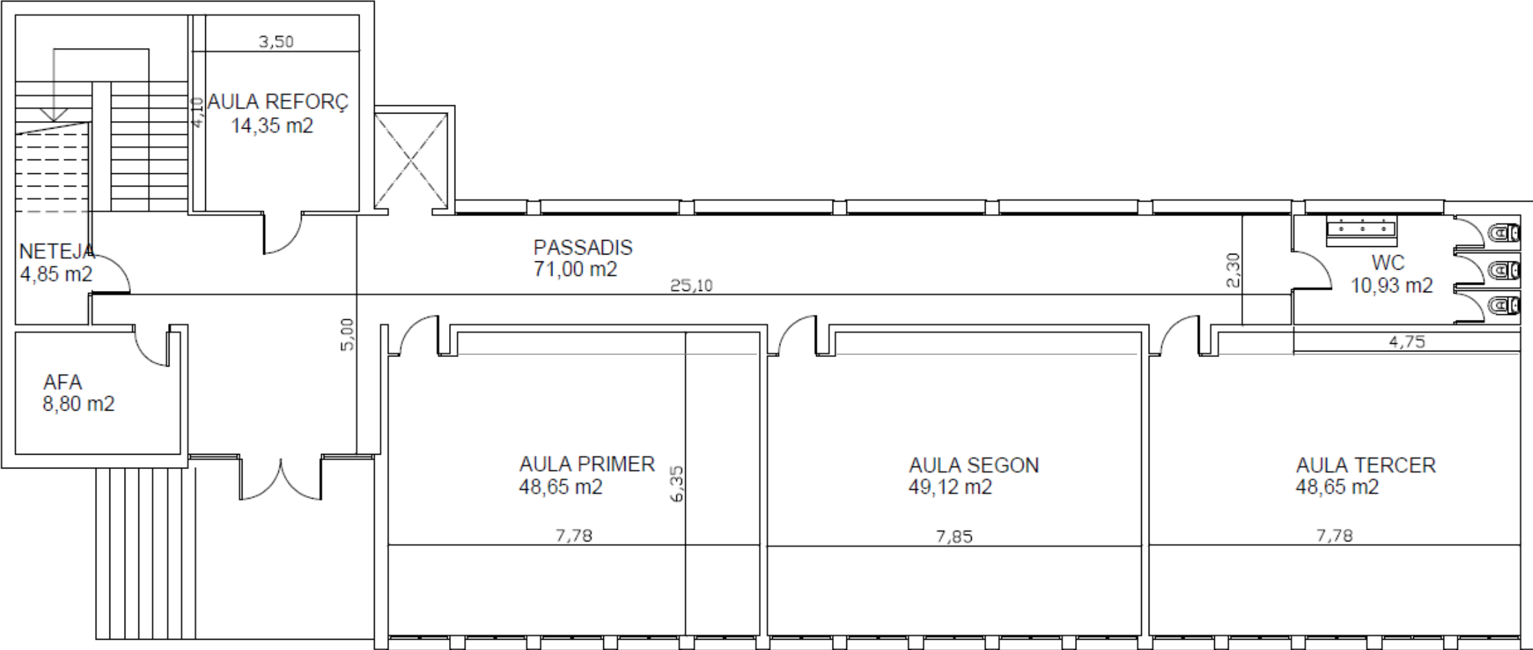
PLANTA BAIXA
