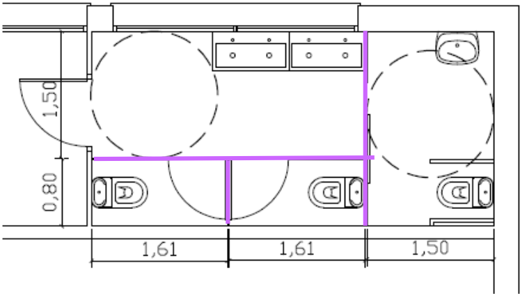
EDIFICI 1: Planta baixa i planta pis
