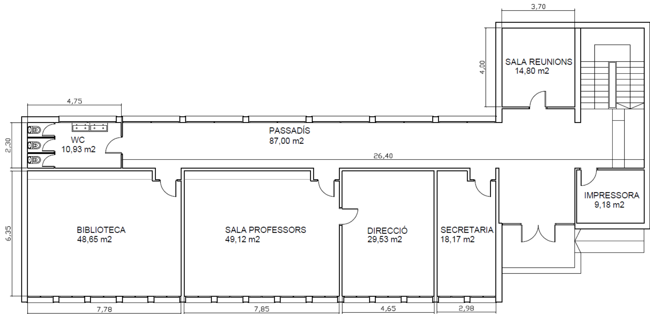
PLANTA BAIXA
