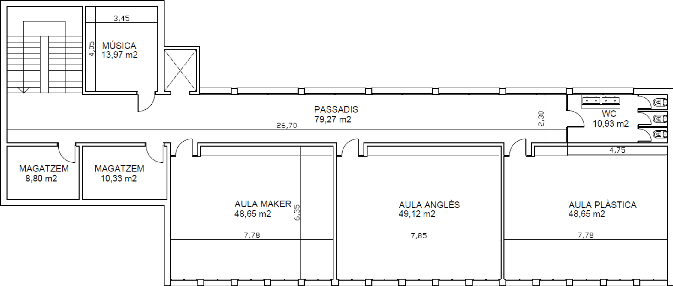
PLANTA PIS
