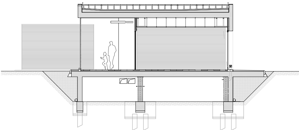
Secció f-f' 1:150
