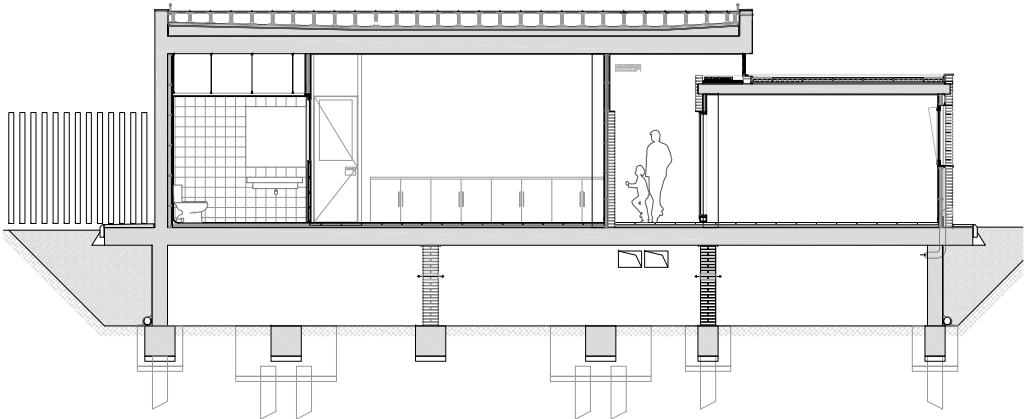
Secció c-c' 1:150
