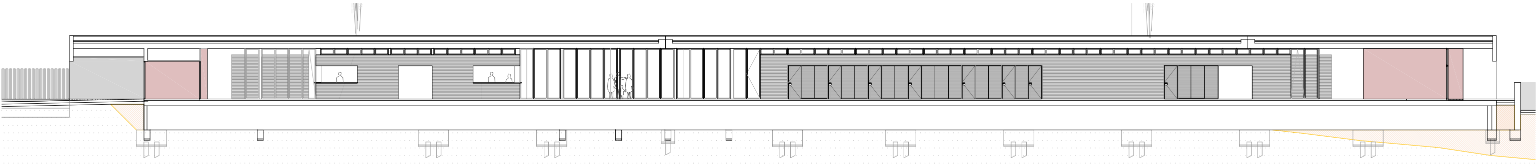
Secció a-a' 1:250
