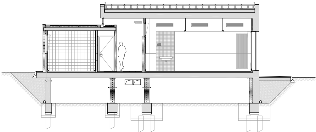
Secció e-e' 1:150
