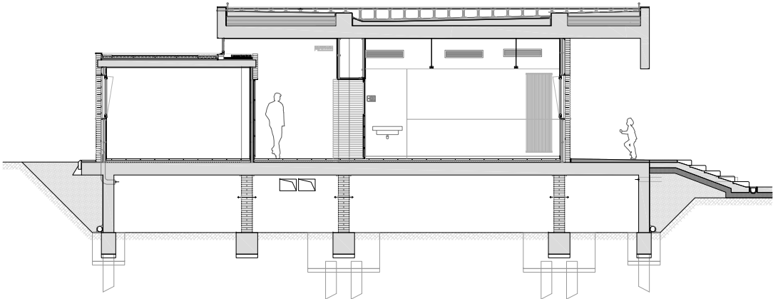
Secció d-d' 1:150
