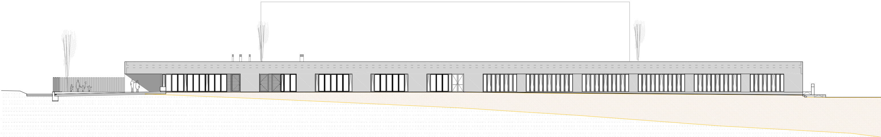
Alçats C-C'
