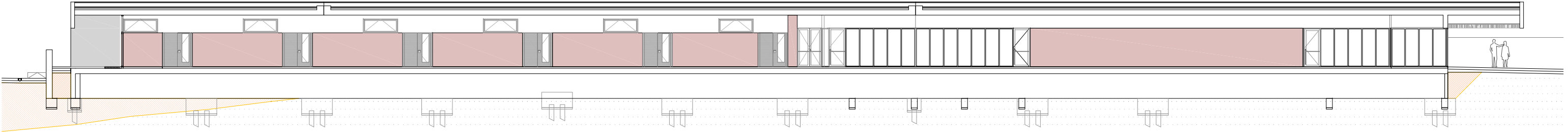
Secció b-b' 1:250
