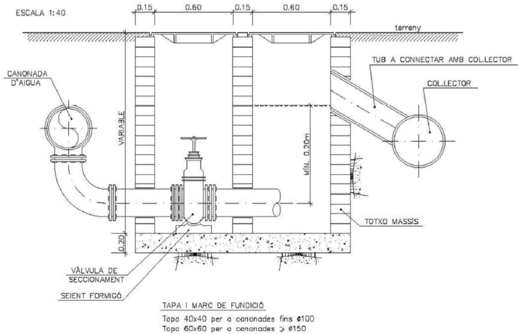
Fig. Arqueta tipus per descàrrega sobre canonada
