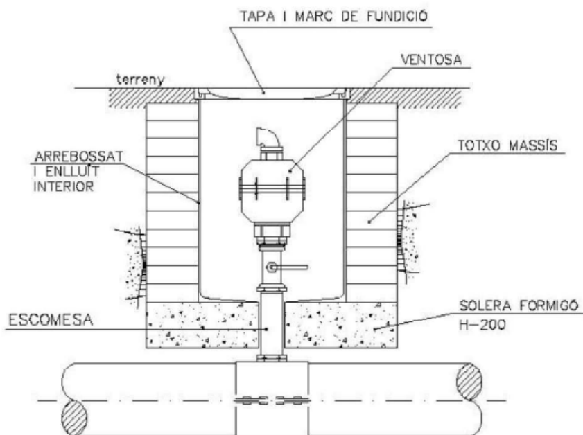
Fig. Arqueta tipus per ventosa
