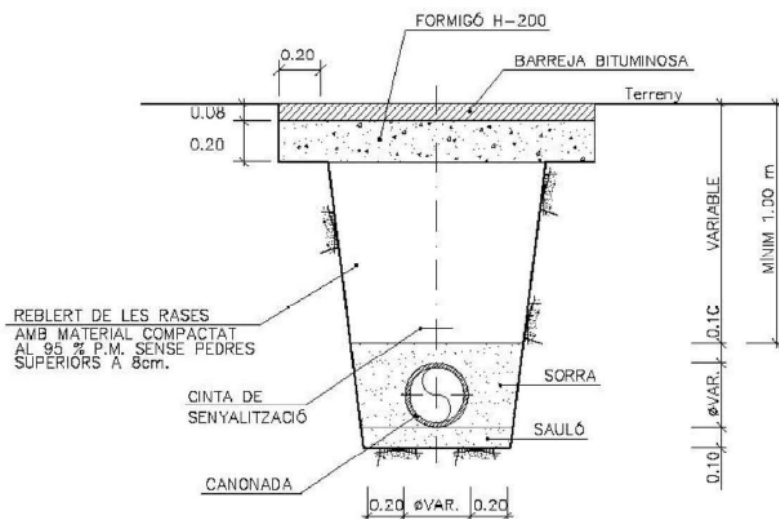
Fig. Rasa tipus sota calçada
