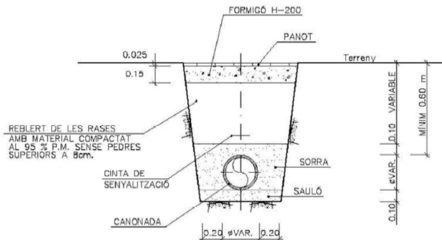
Fig. Rasa tipus sota vorera
