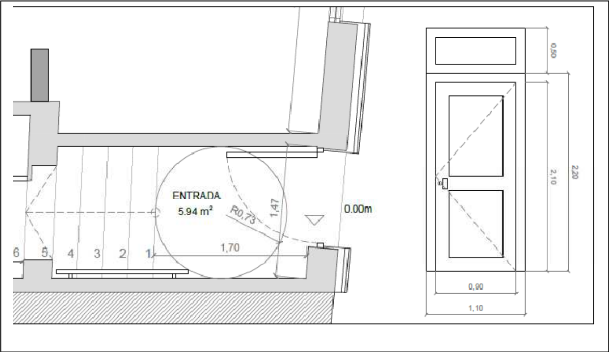
Foto del graó actual i dibuix de la nova porta (baix)
