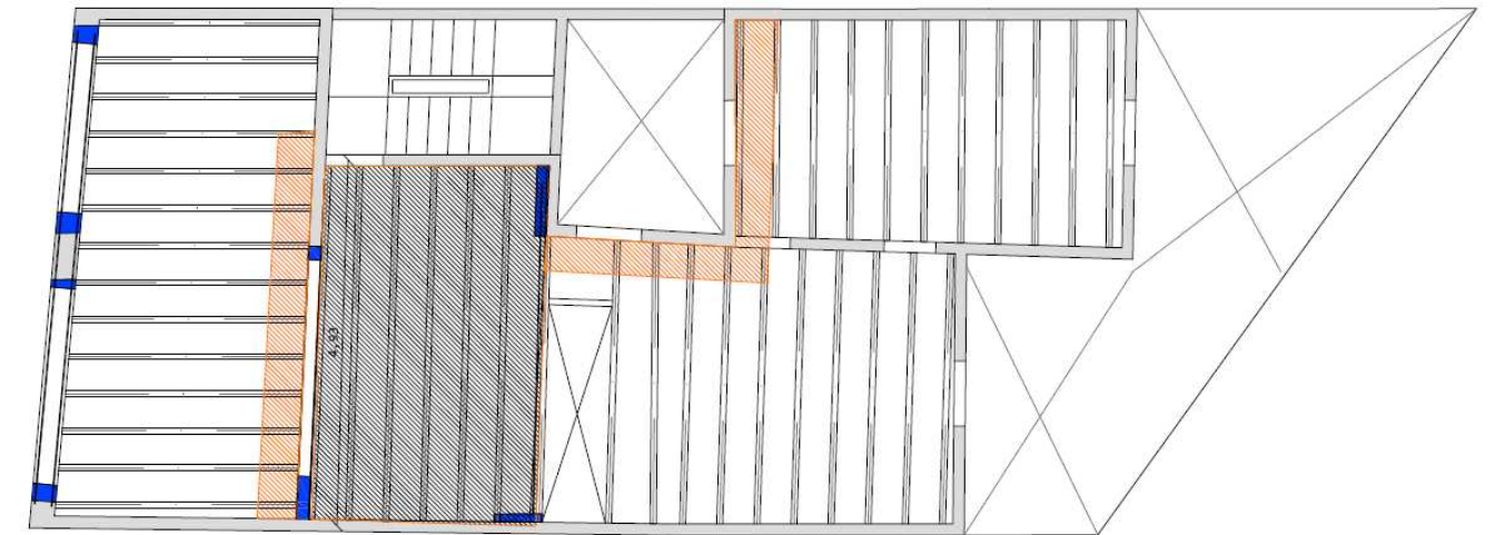
Planol d'estructura planta 3ª en gris zona de reforç de biguetes En Blau nous reforços verticals de Maó per nous perfils d'Acer als envans. En taronja zones a revisar i fer tractament preventiu.
