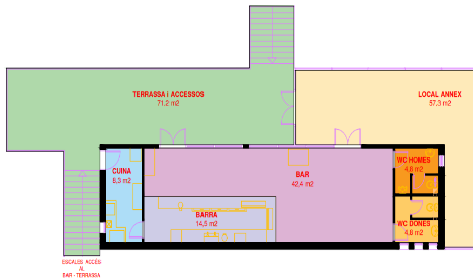
ANNEX NÚMERO 1 PLÀNOL DE LES INSTAL·LACIONS
