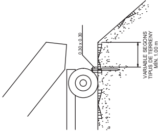
TOPALL PER A VEHICLES AUTOMÒBILS
