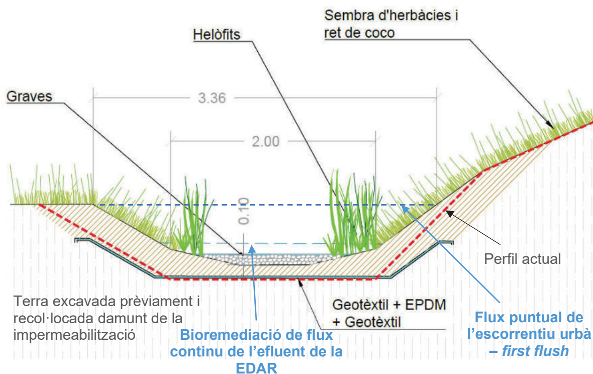
Figura 21 Secció del canal
