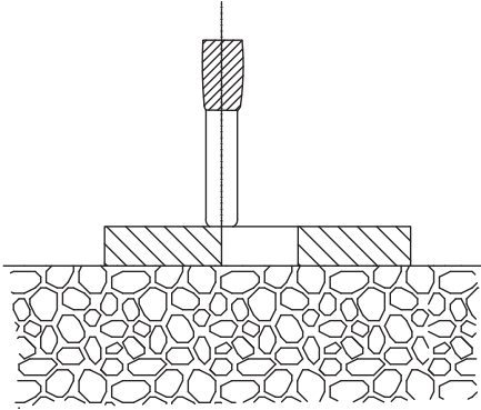
PERILL DE TIR A TRAVÉS DE FORAT
