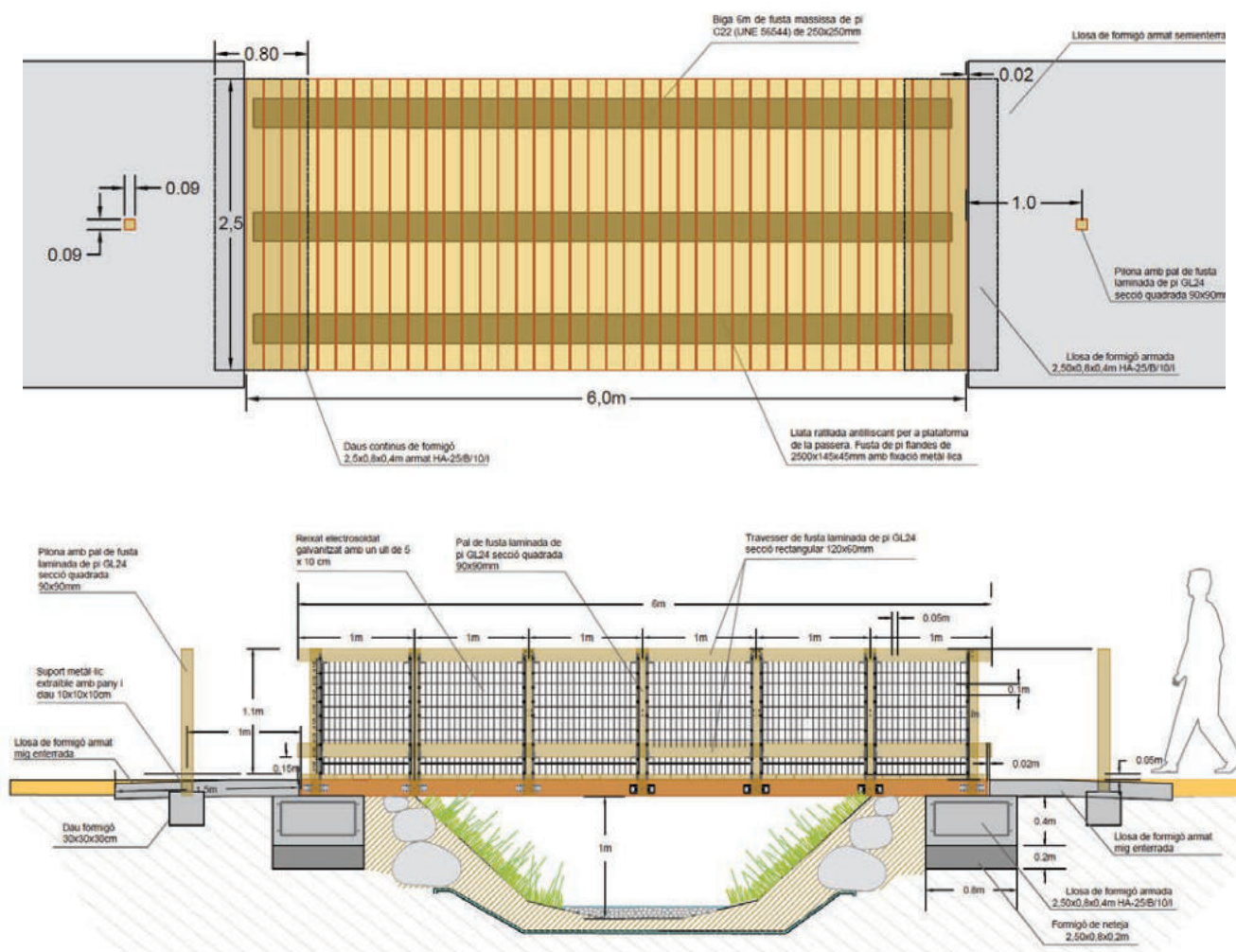
Figura 28 Detalls de la passera de fusta
