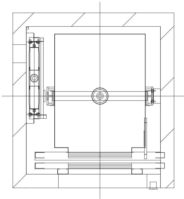
Detall últim nivell 1:25
