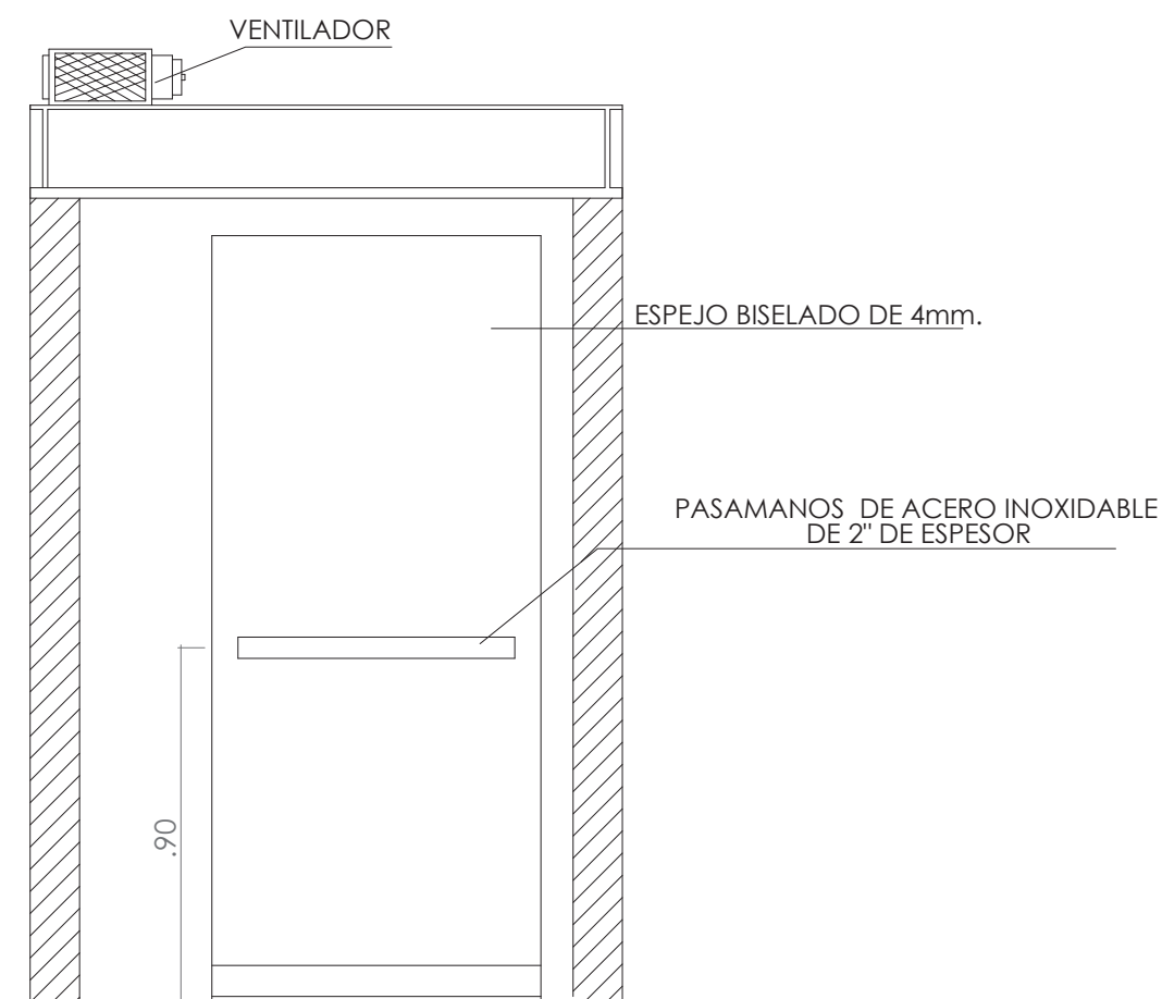
CORTE A'-A'
