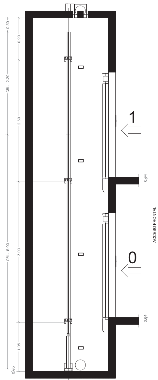
Secció vertical lado limitador 1:50
