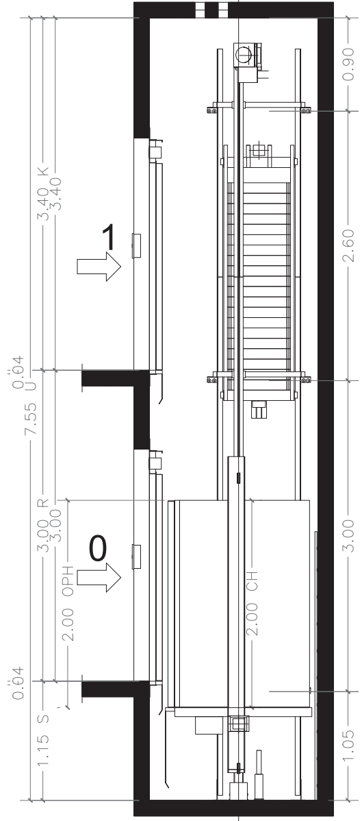
Secció vertical lado máquina 1:50
