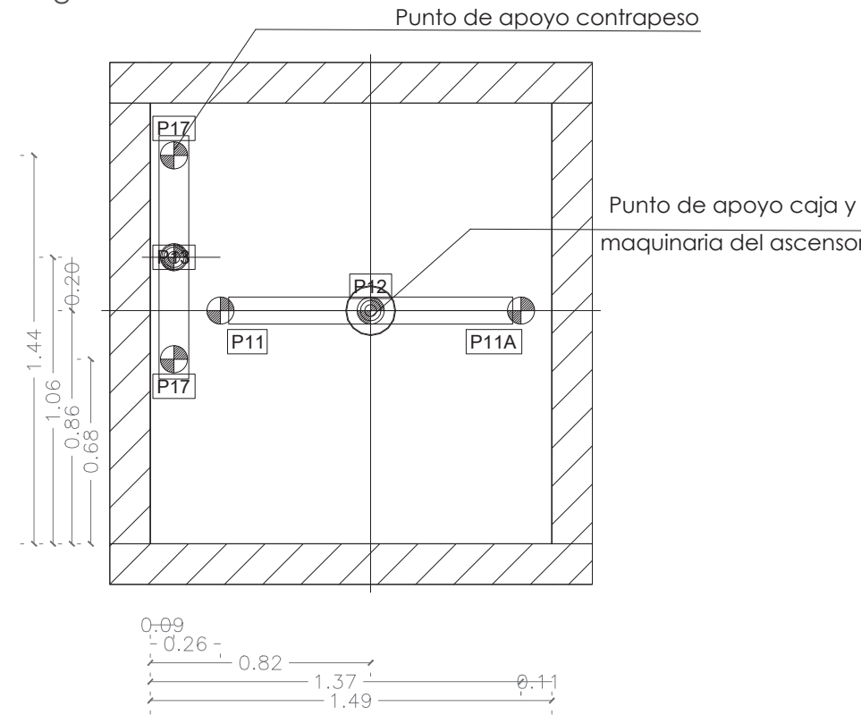
Cargas de foso 1:25
