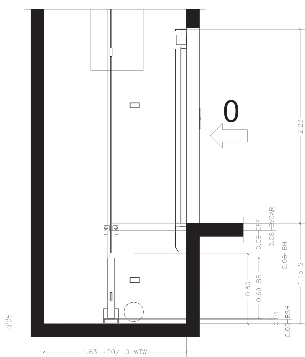
Detall Foso Lado Limitador 1:25
