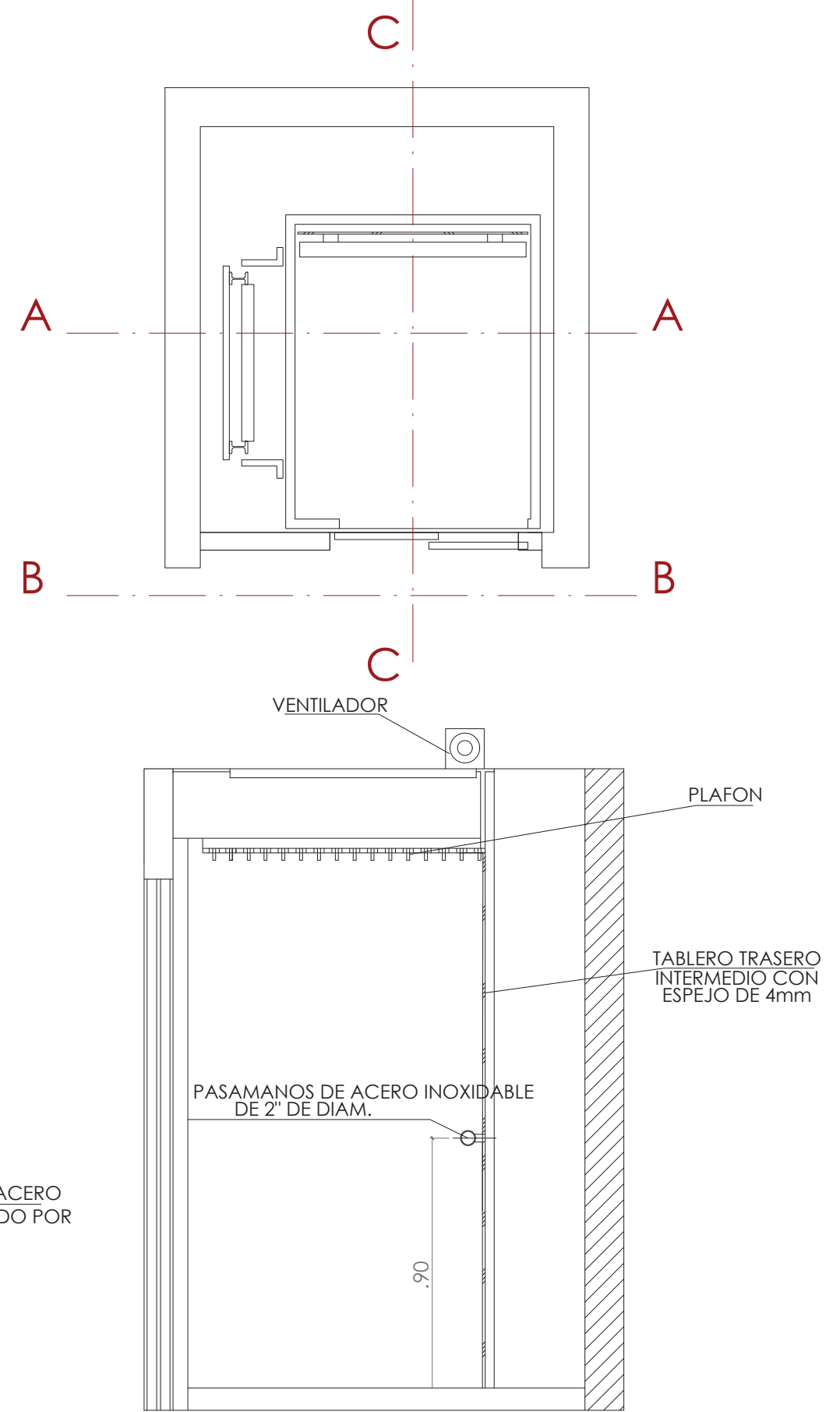
CORTE C'-C'
