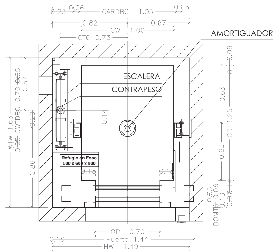
Planta hueco 1:25
