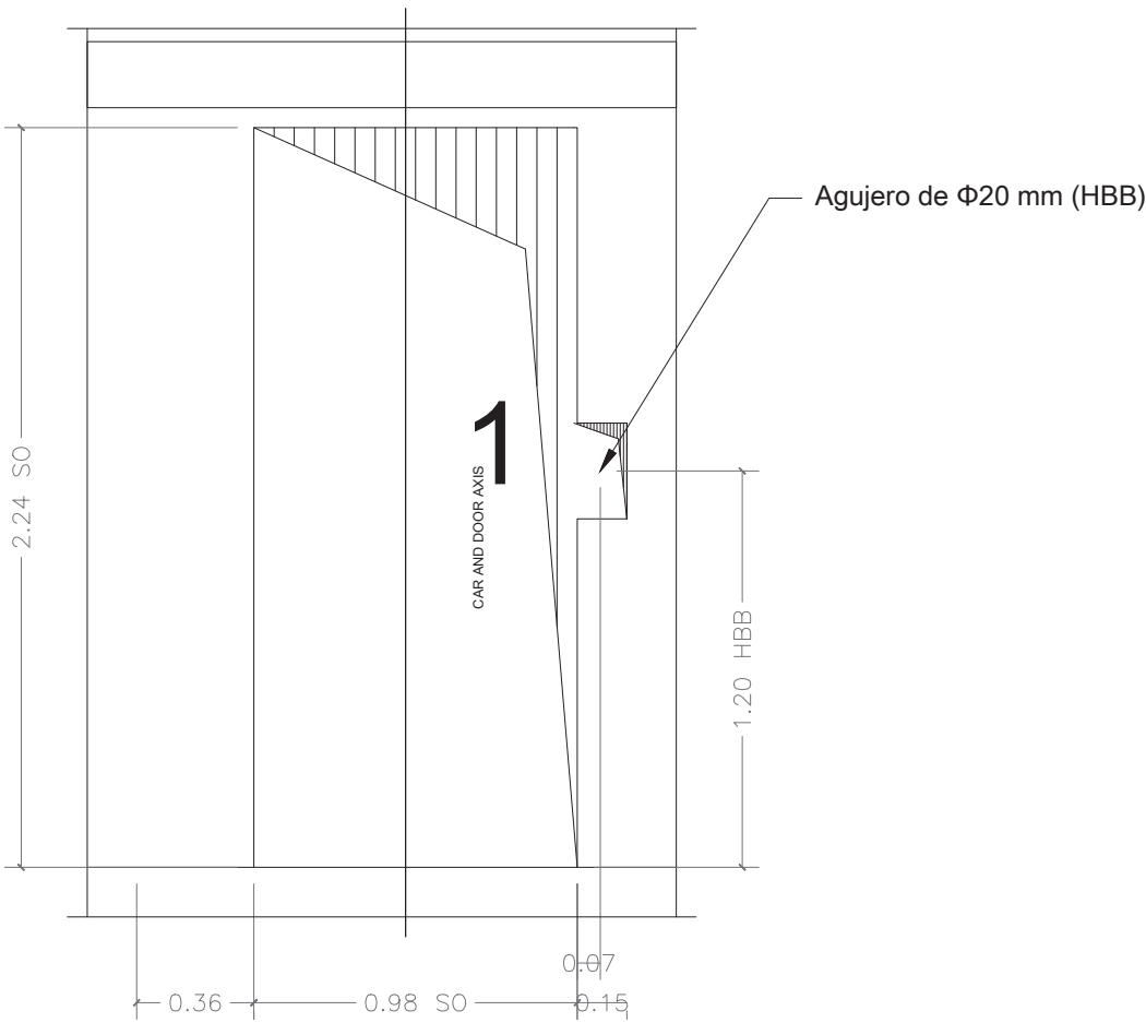
Hueco estructra planta principal 1:25
