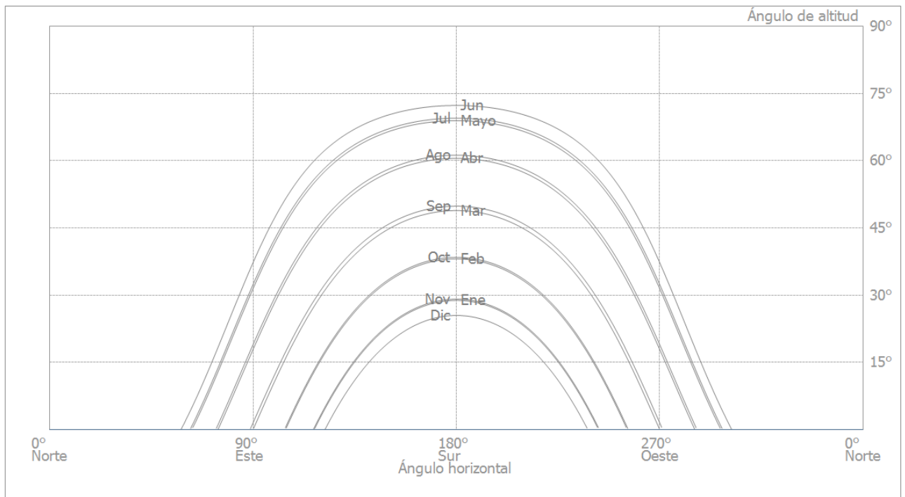
Figura: Horizonte (Planificació 3D)
